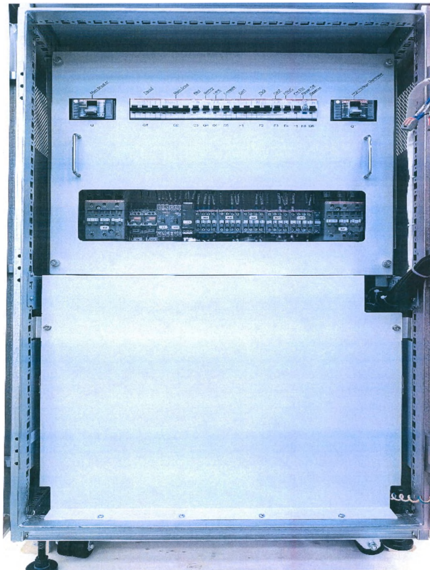
Шкаф электропитания для вариантов исполнения uCT 520 и 528
