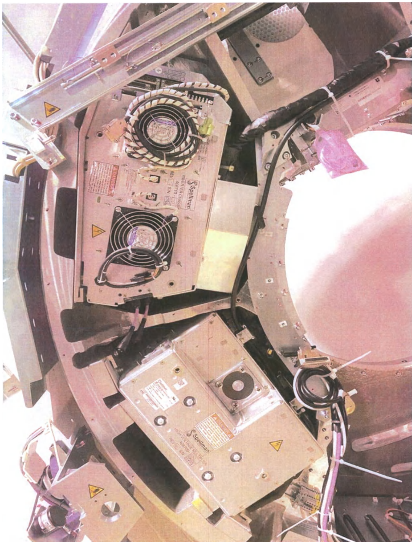
Генератор высоковольтный для вариантов исполнения иСТ 760 и 780
