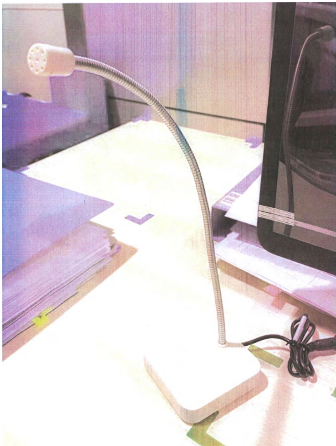
Микрофон с гибким штативом для вариантов исполнения иСТ 760 и 780
