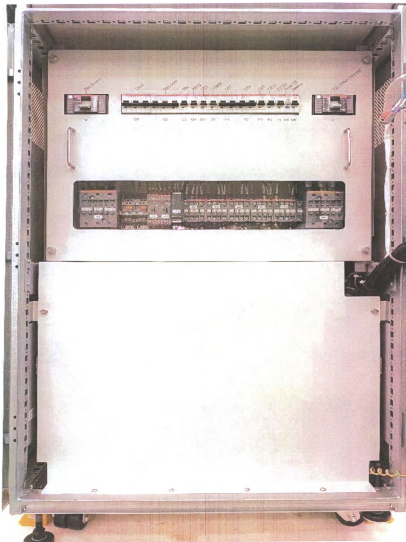
Шкаф электропитания для вариантов исполнения uCT 760 и 780
