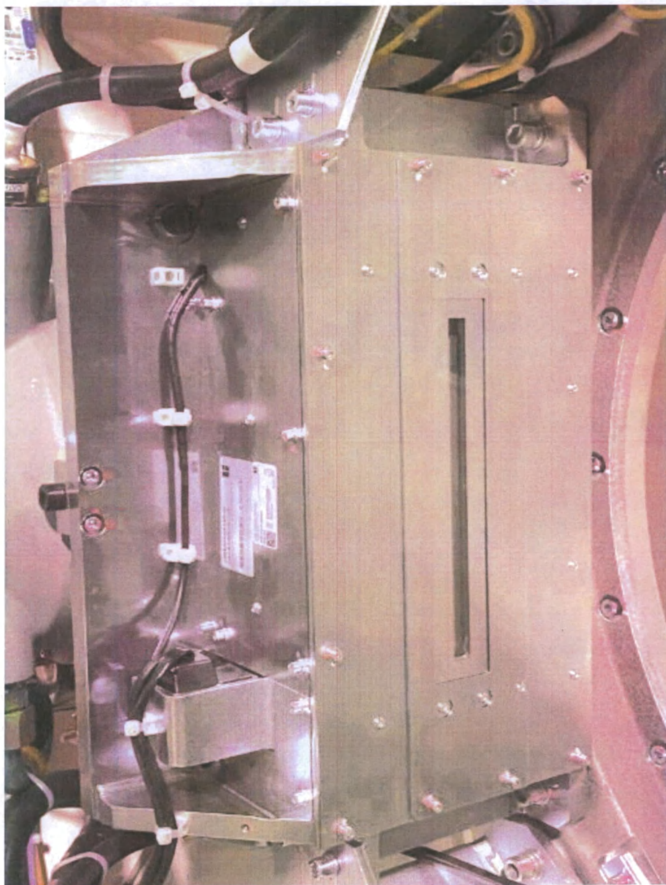
Коллиматор для вариантов исполнения иСТ 760 и 780
