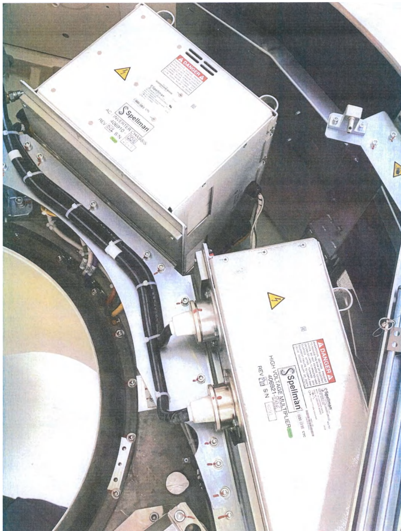
Генератор высоковольтный для вариантов исполнения иСТ 530 и 550
