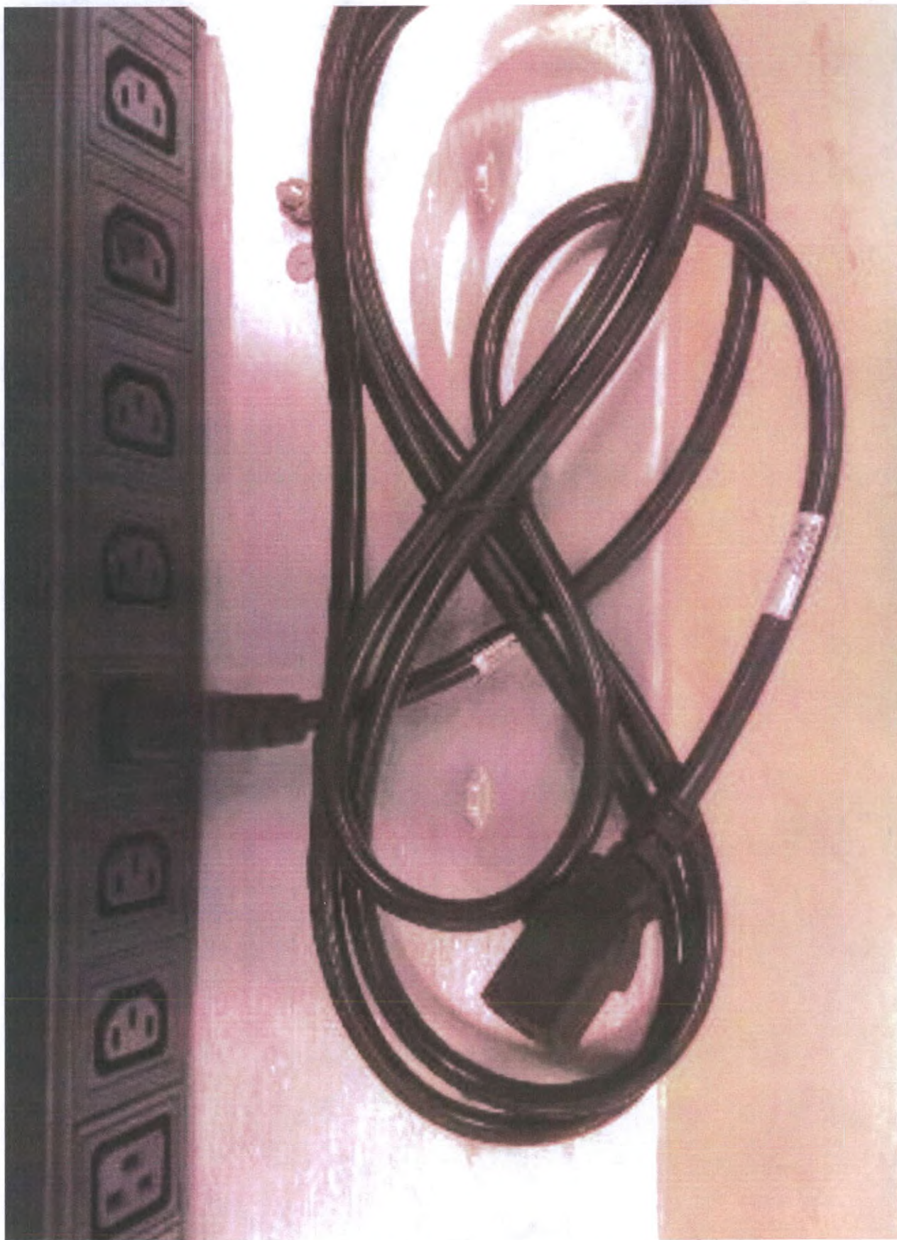
Кабель питания процессора для вариантов исполнения иСТ 530 и 550
