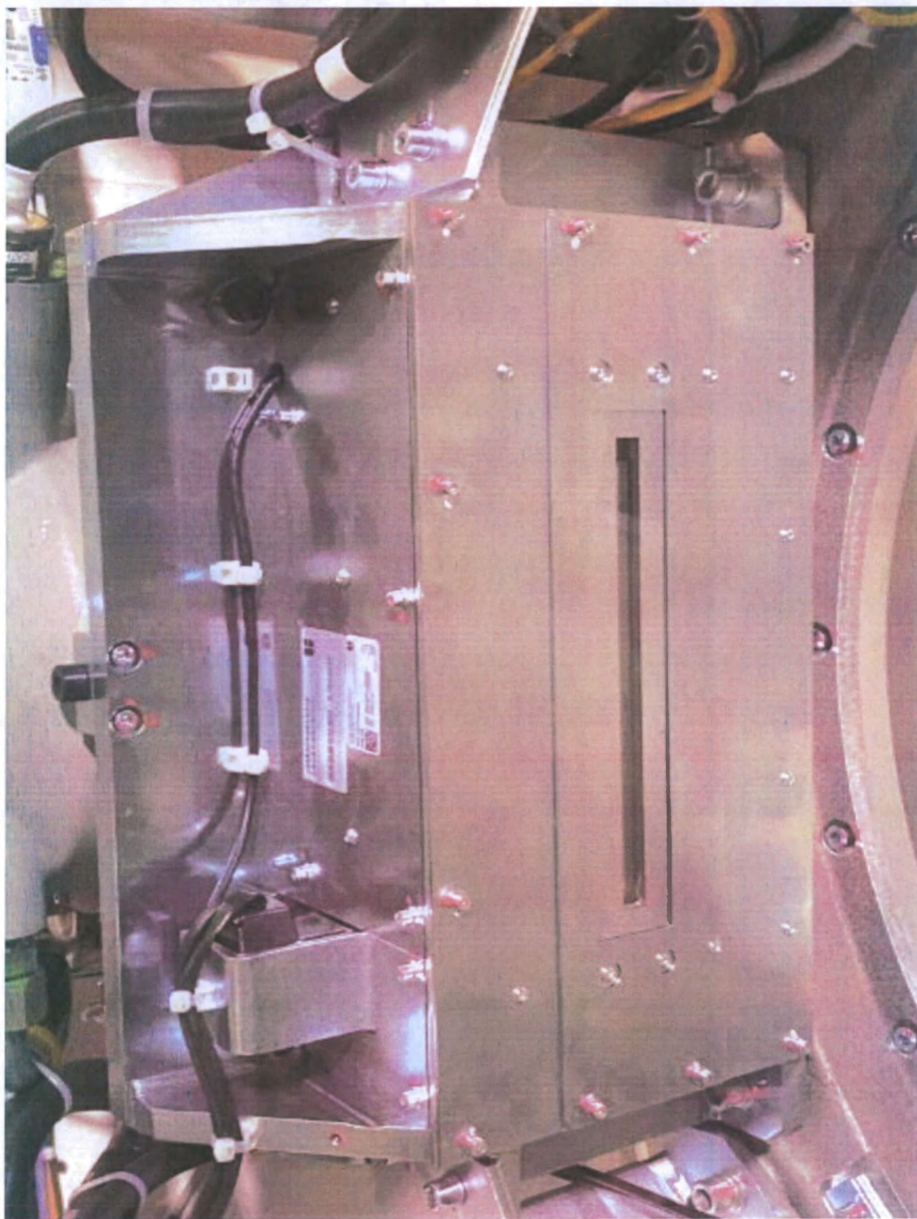
Коллиматор для вариантов исполнения иСТ 530 и 550
