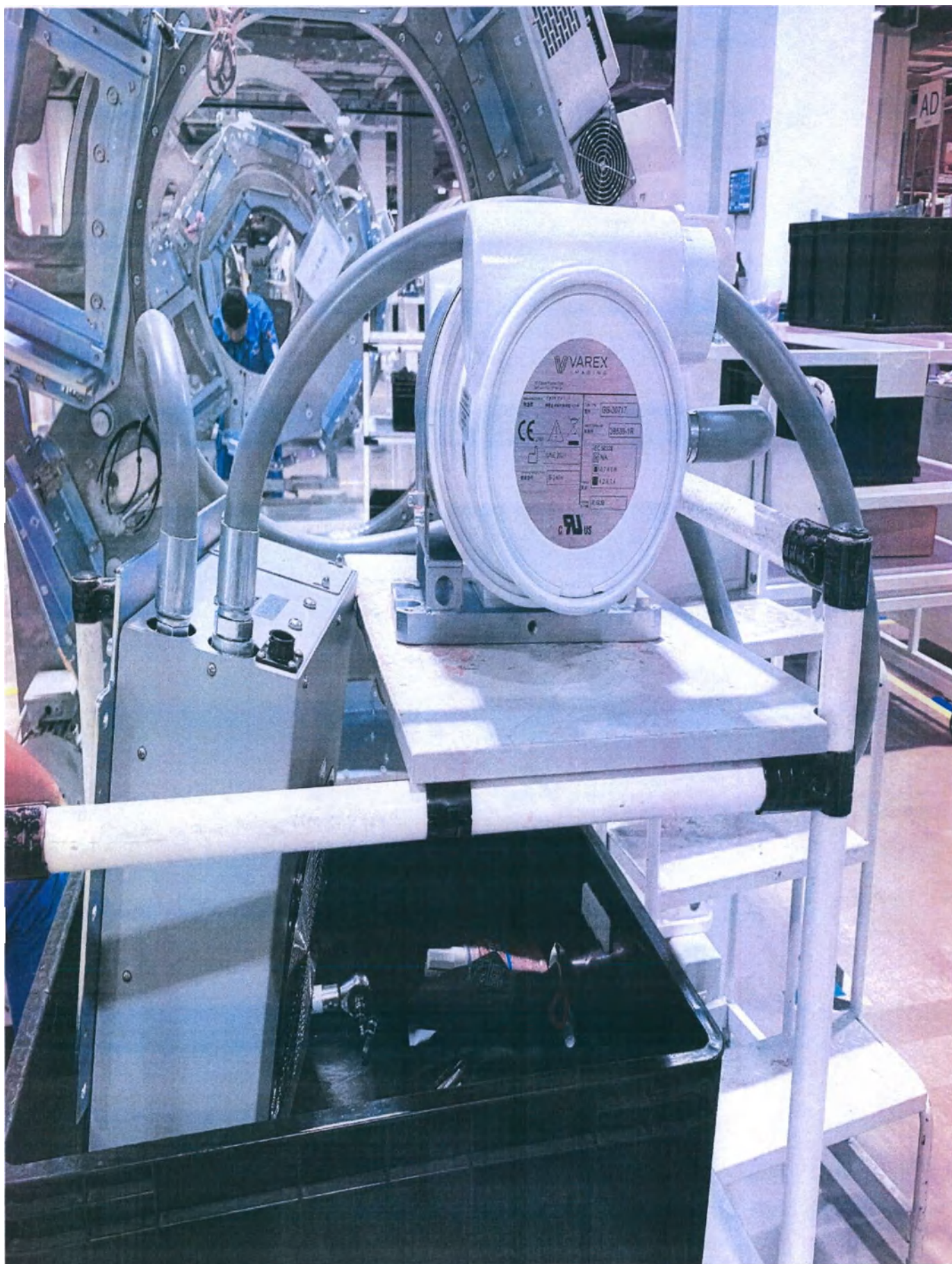
Излучатель рентгеновский для вариантов исполнения uCT 520 и 528
