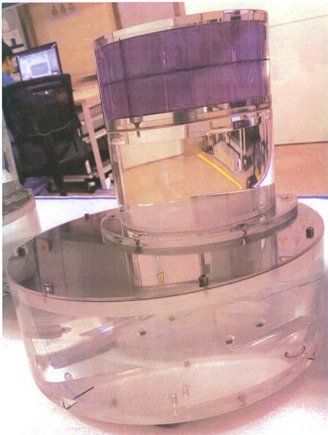
Фантом системный (при необходимости) для вариантов исполнения иСТ 530 и 550
