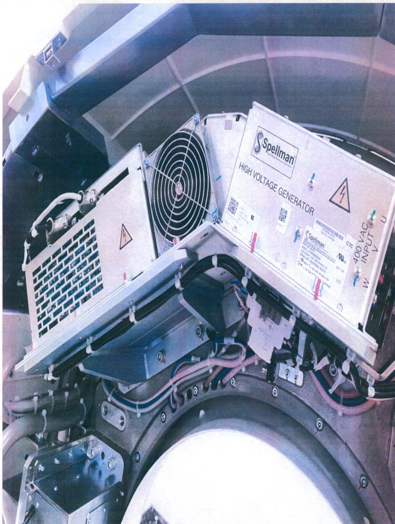
Генератор высоковольтный для вариантов исполнения иСТ 520 и 528
