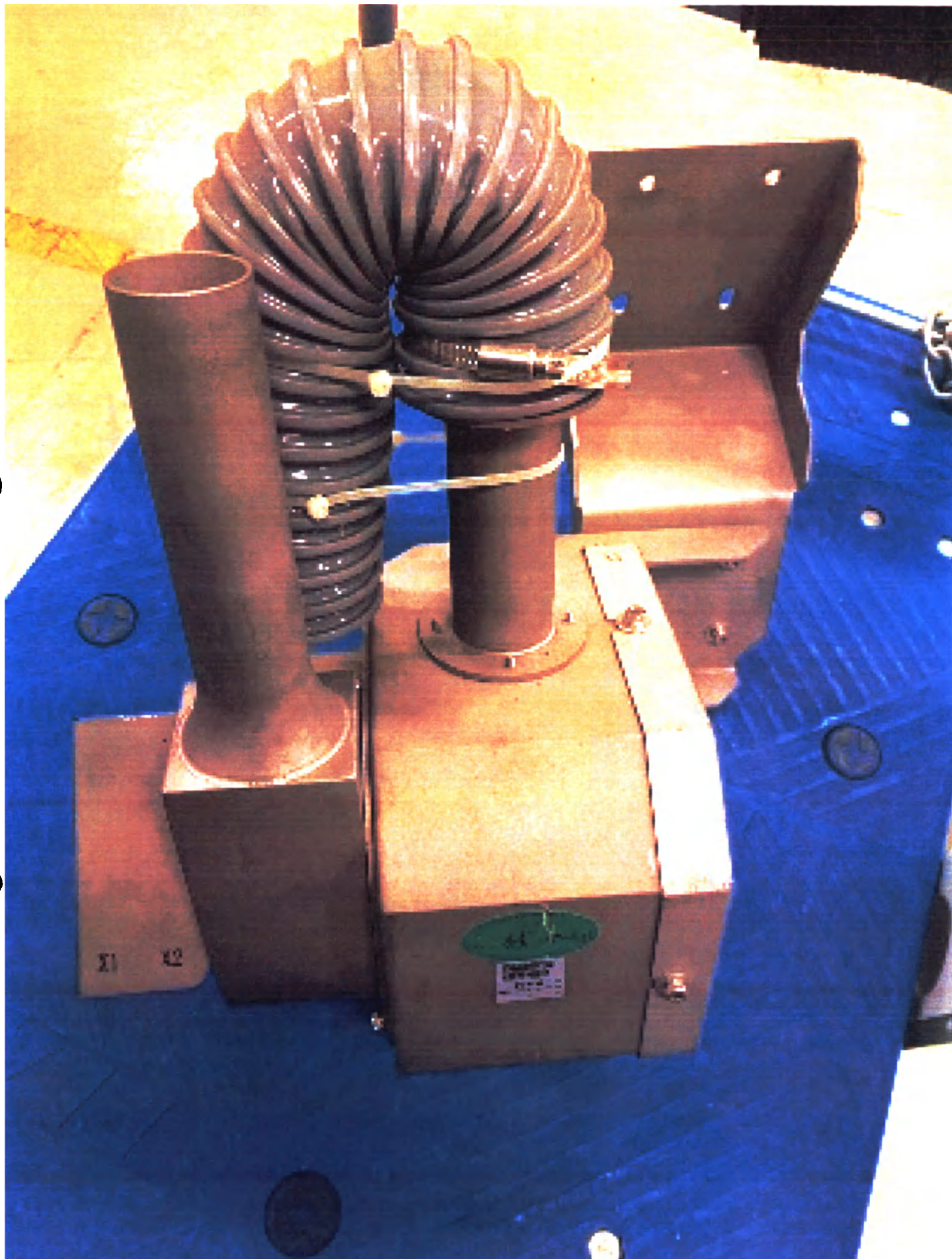
Система подачи воздуха для варианта исполнения uMR 570
