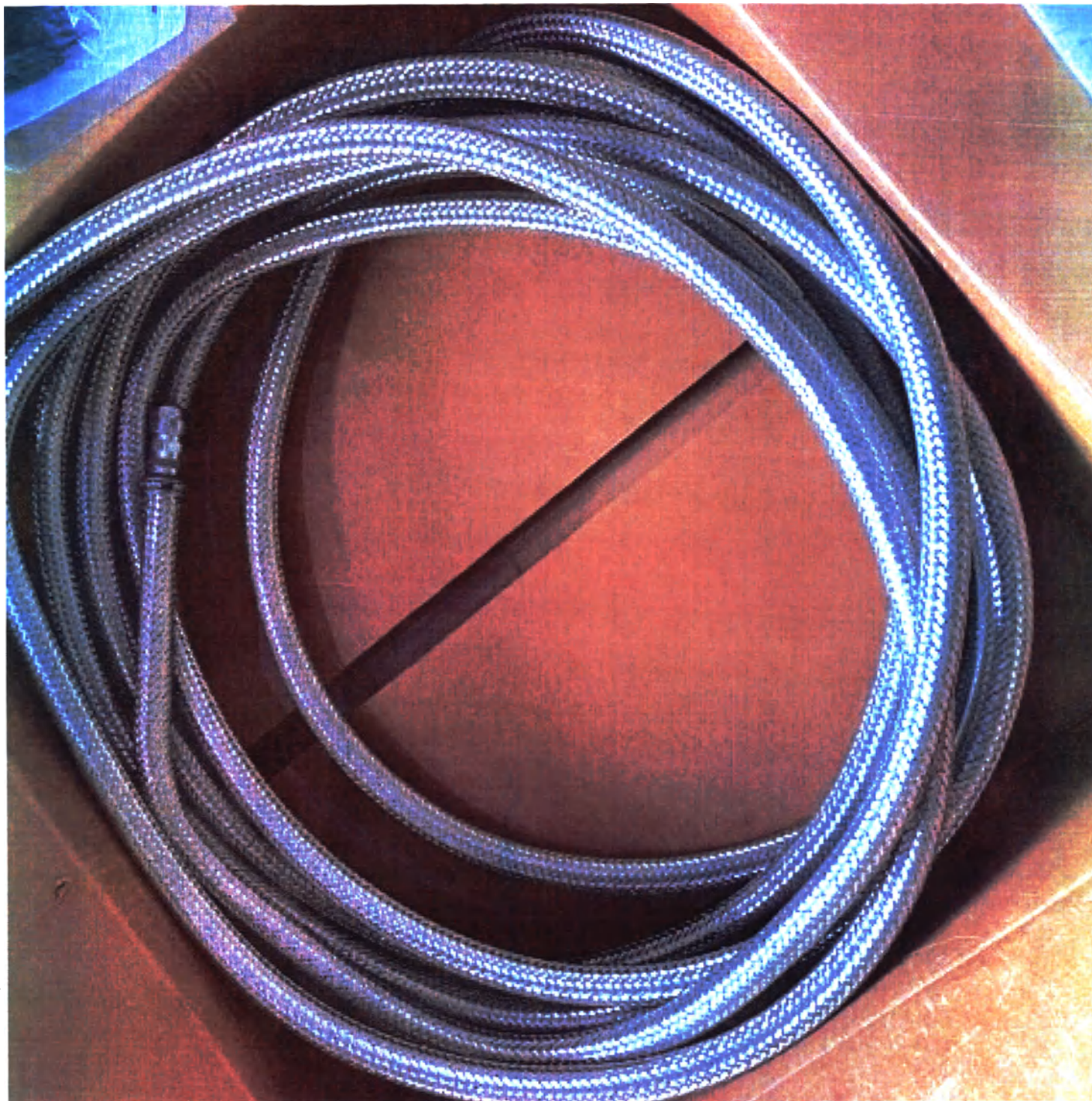
Линия подачи геля для варианта исполнения uMR Omega
