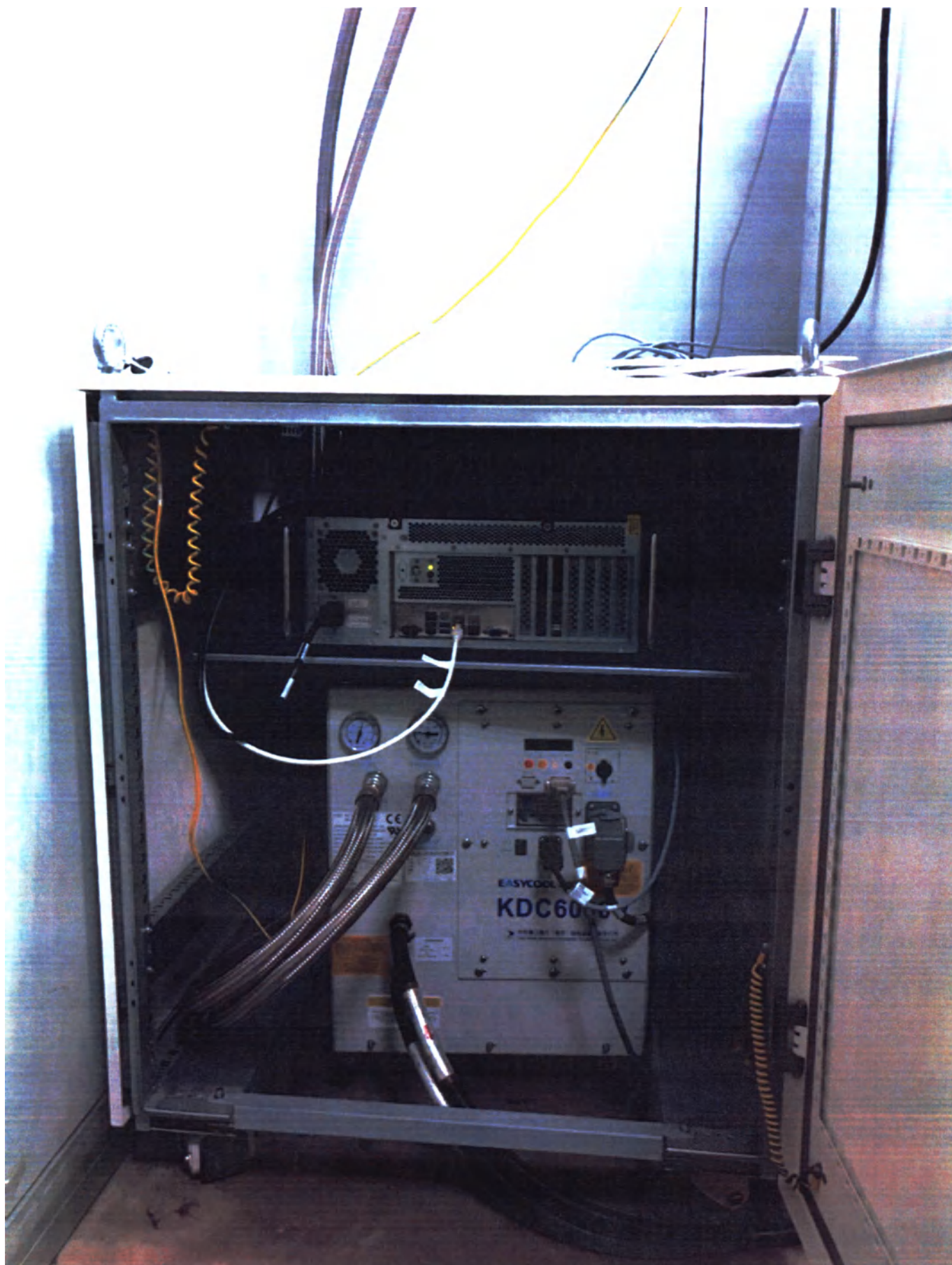
Шкаф M0 CAS (при необходимости) для вариантов исполнения uMR 580 и 588
