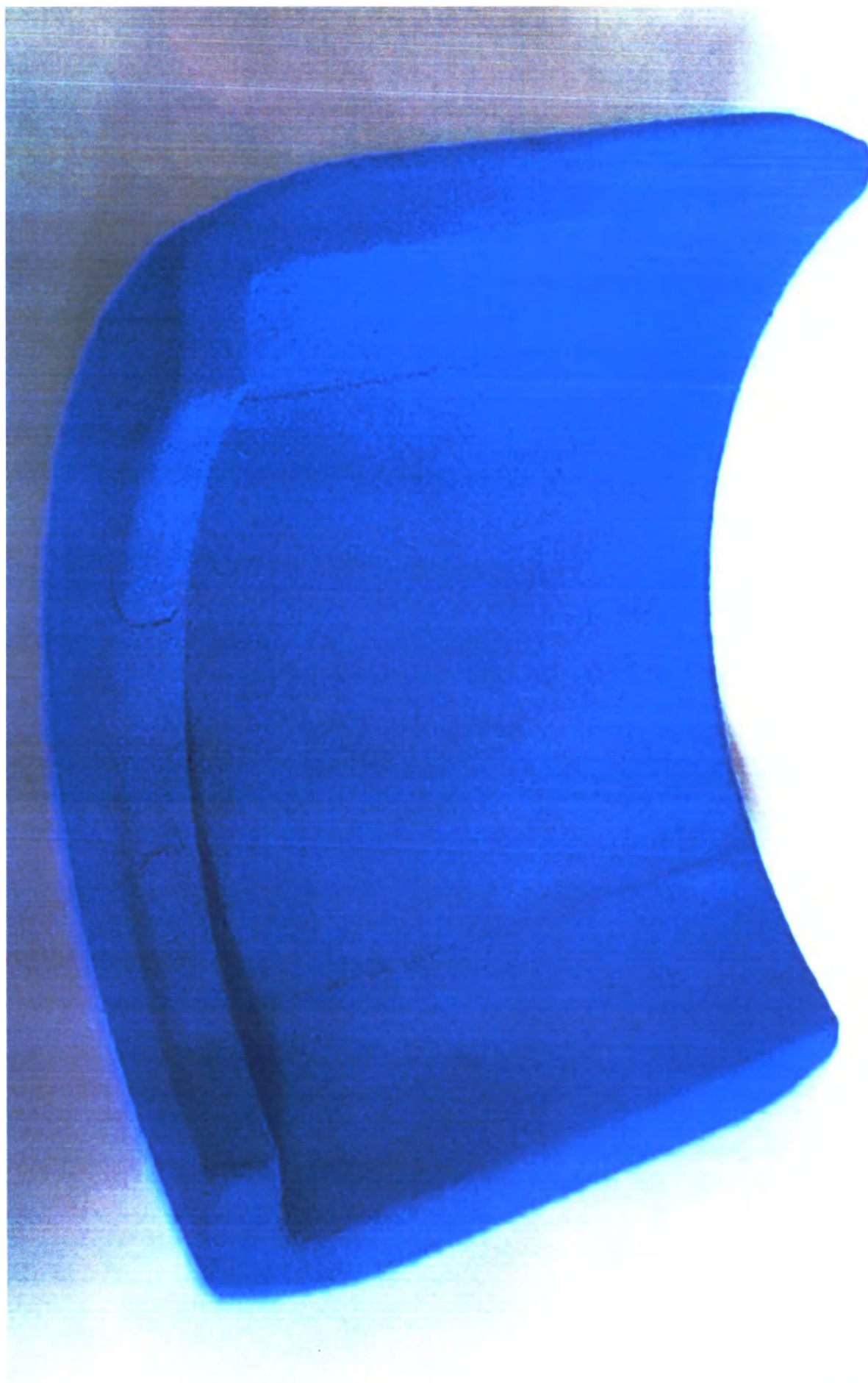
Поддон под водный фантом ACR для вариантов исполнения uMR 580 и 588
