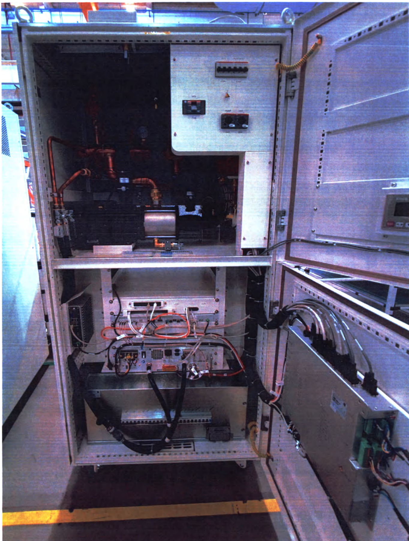
Электрический шкаф для вариантов исполнения uMR 580 и 588
