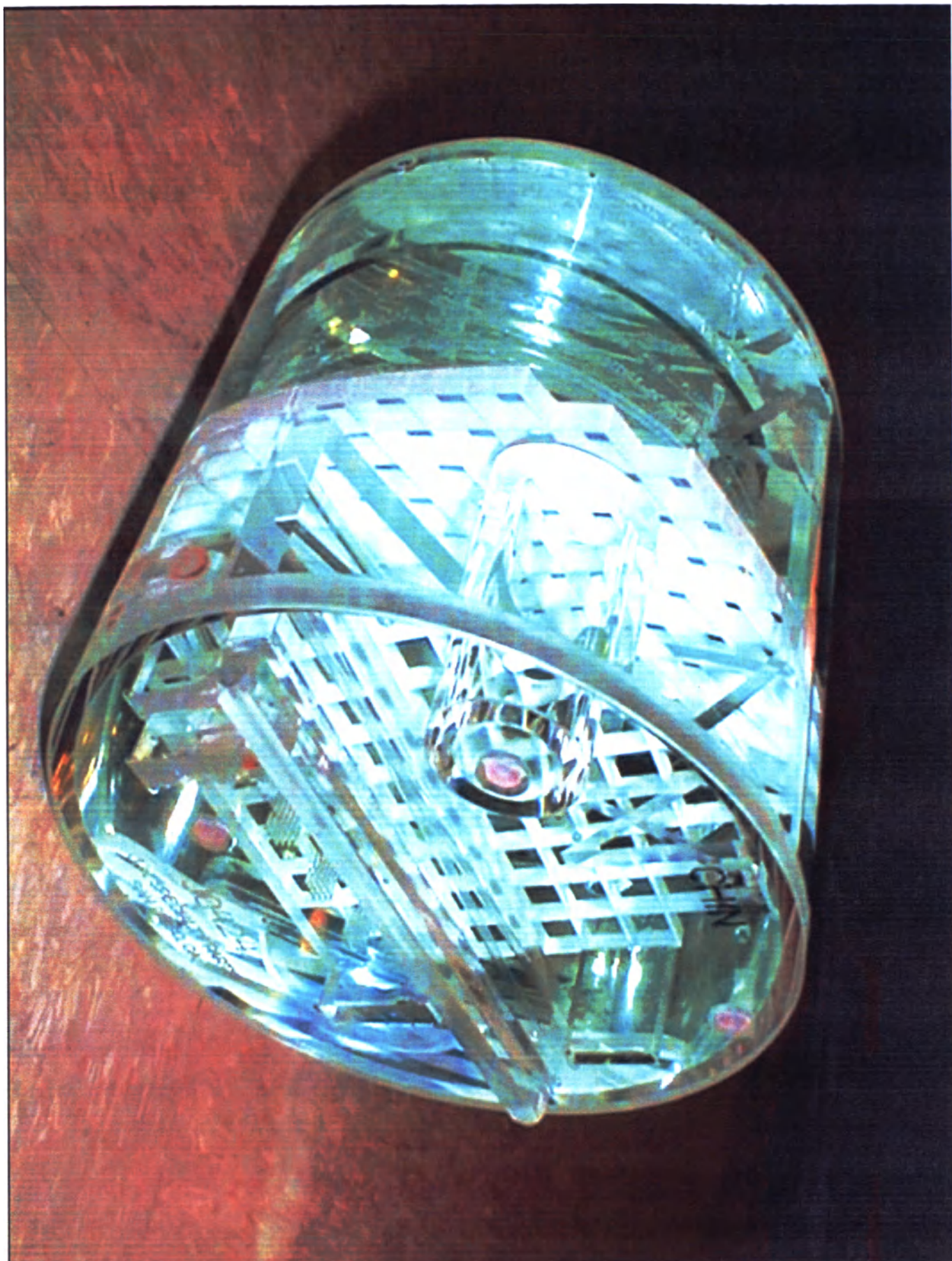
Водный фантом ACR для варианта исполнения uMR 570
