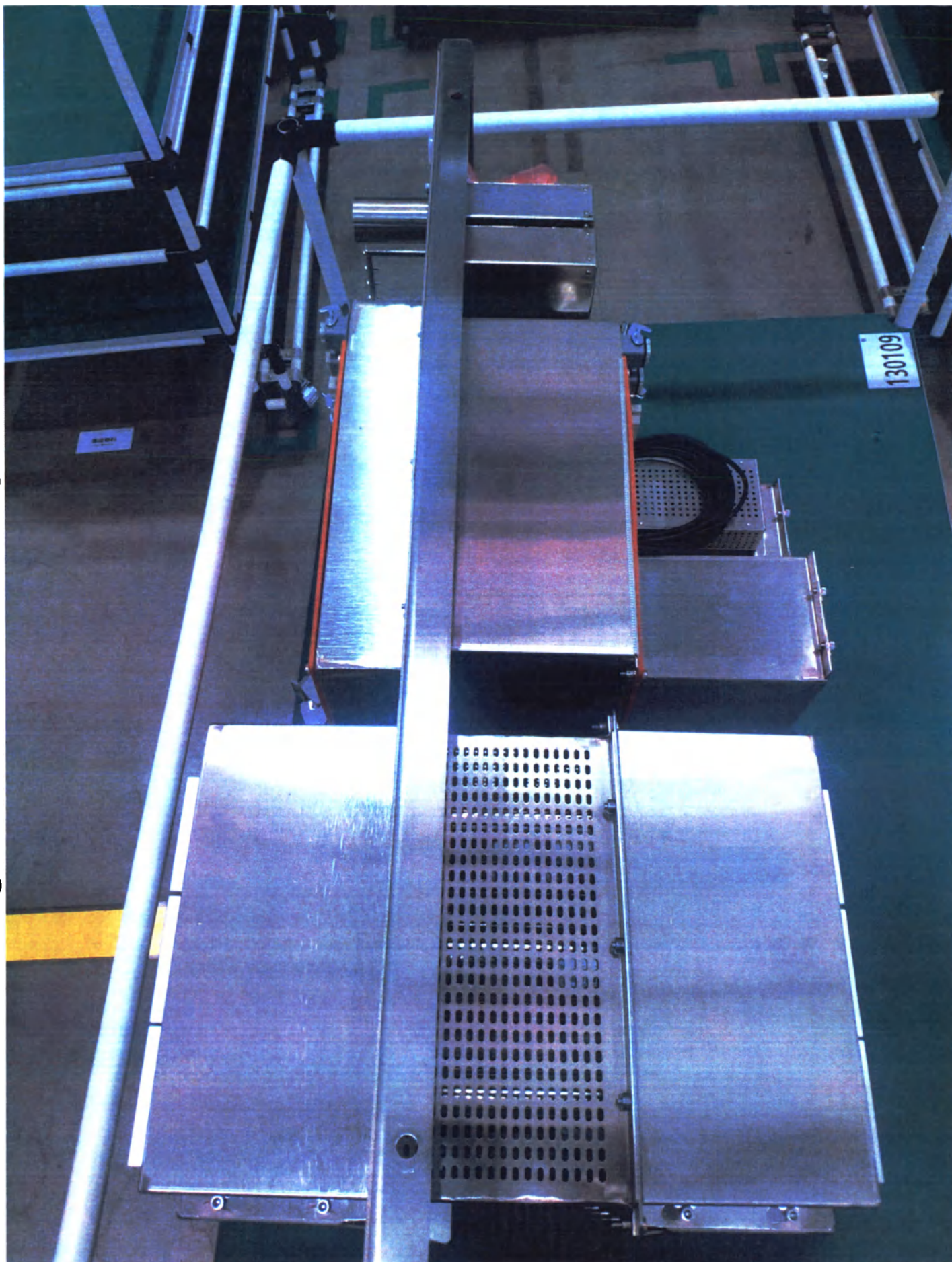
Пластина фильтра для варианта исполнения uMR 570
