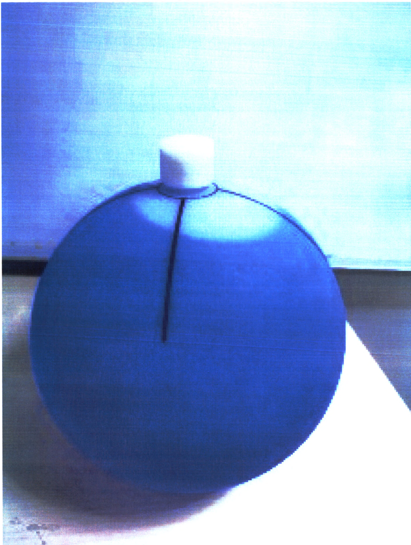
Водный фантом D250 для варианта исполнения uMR 780
