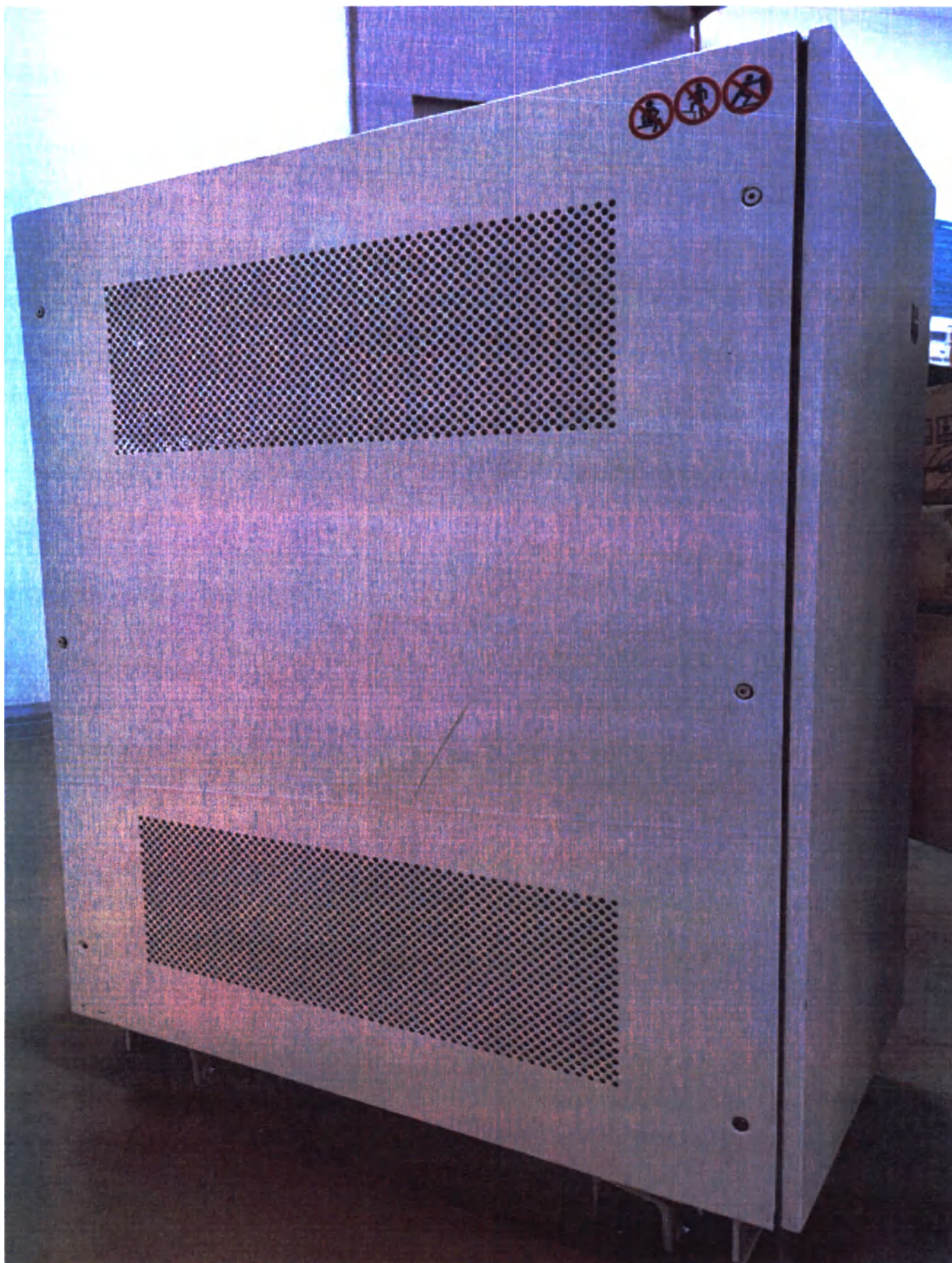
Автотрансформатор 15кВА (при необходимости) для варианта исполнения uMR Omega
