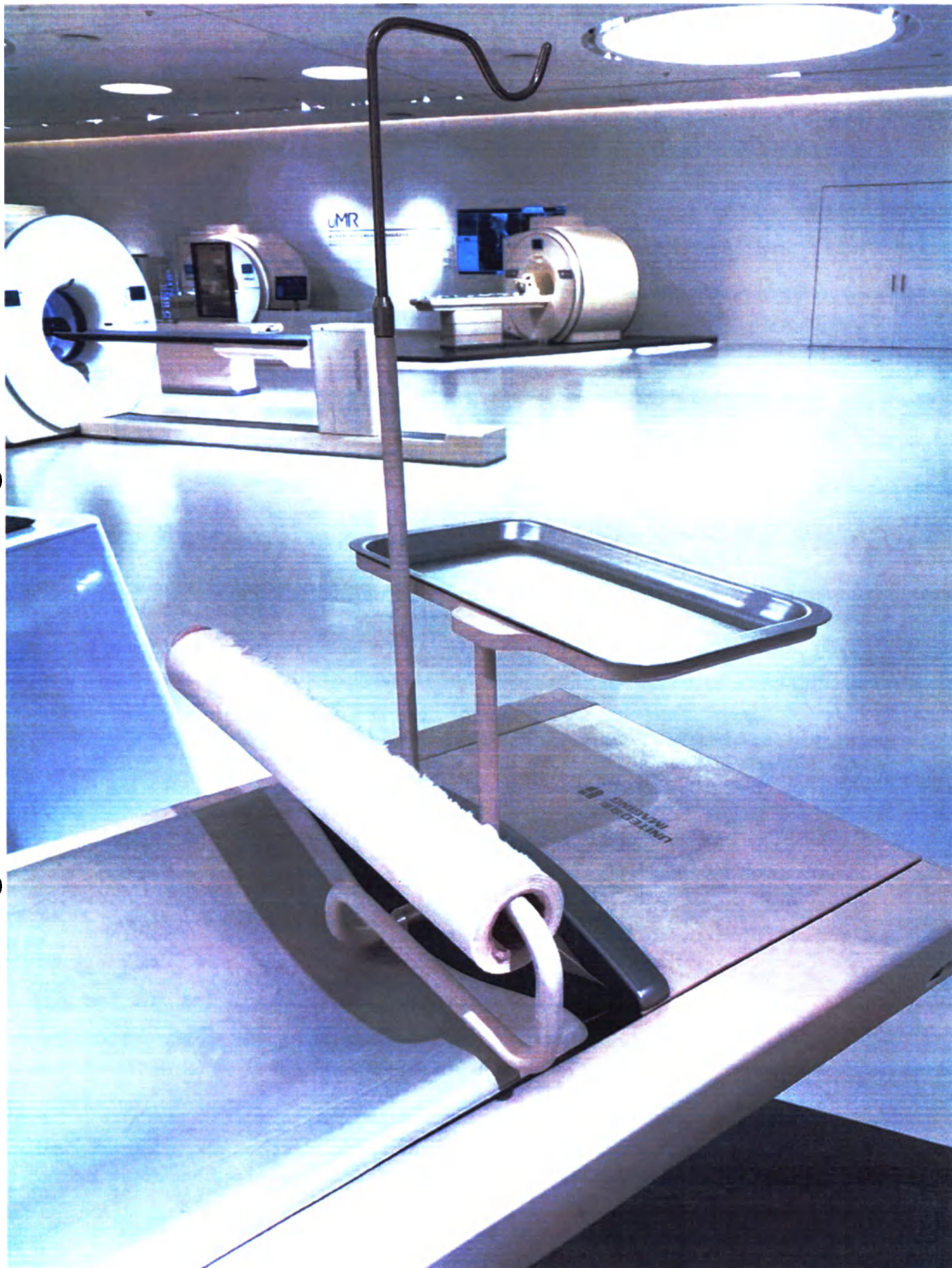
Бумага рулонная с держателем (при необходимости) для варианта исполнения uMR 570
