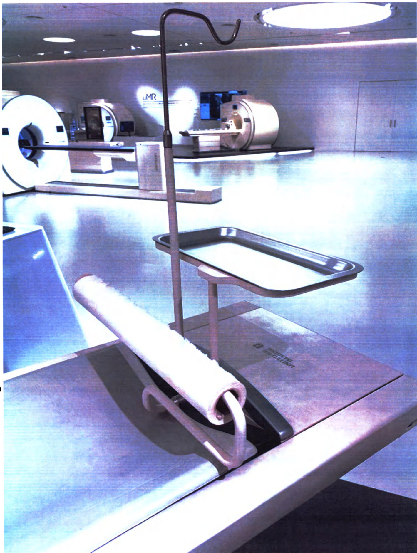
Стойка с капельницей (при необходимости) для вариантов исполнения uMR 580 и 588
