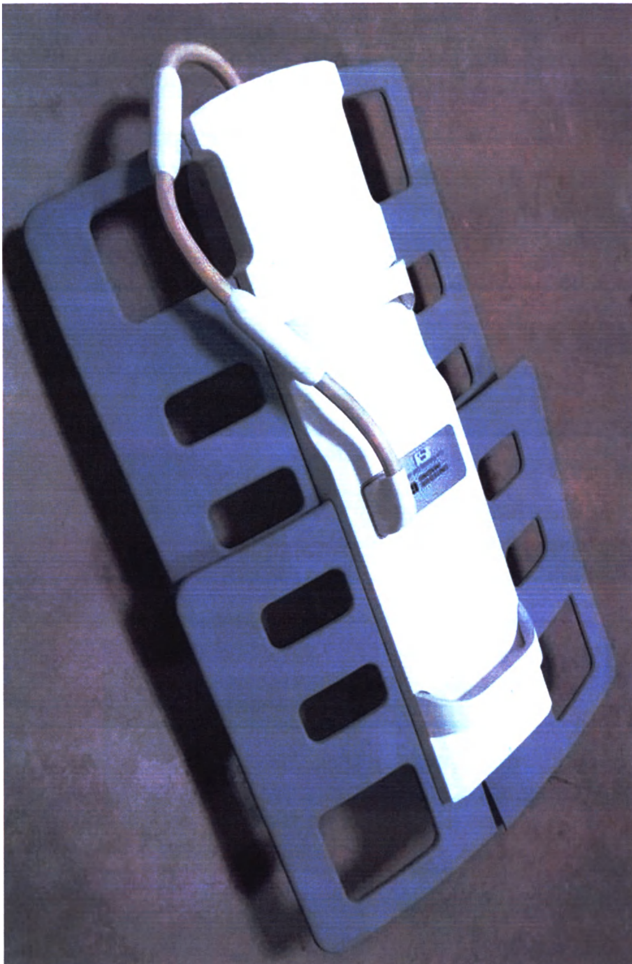
Катушка для нижних конечностей (при необходимости) для вариантов исполнения uMR 580 и 588
