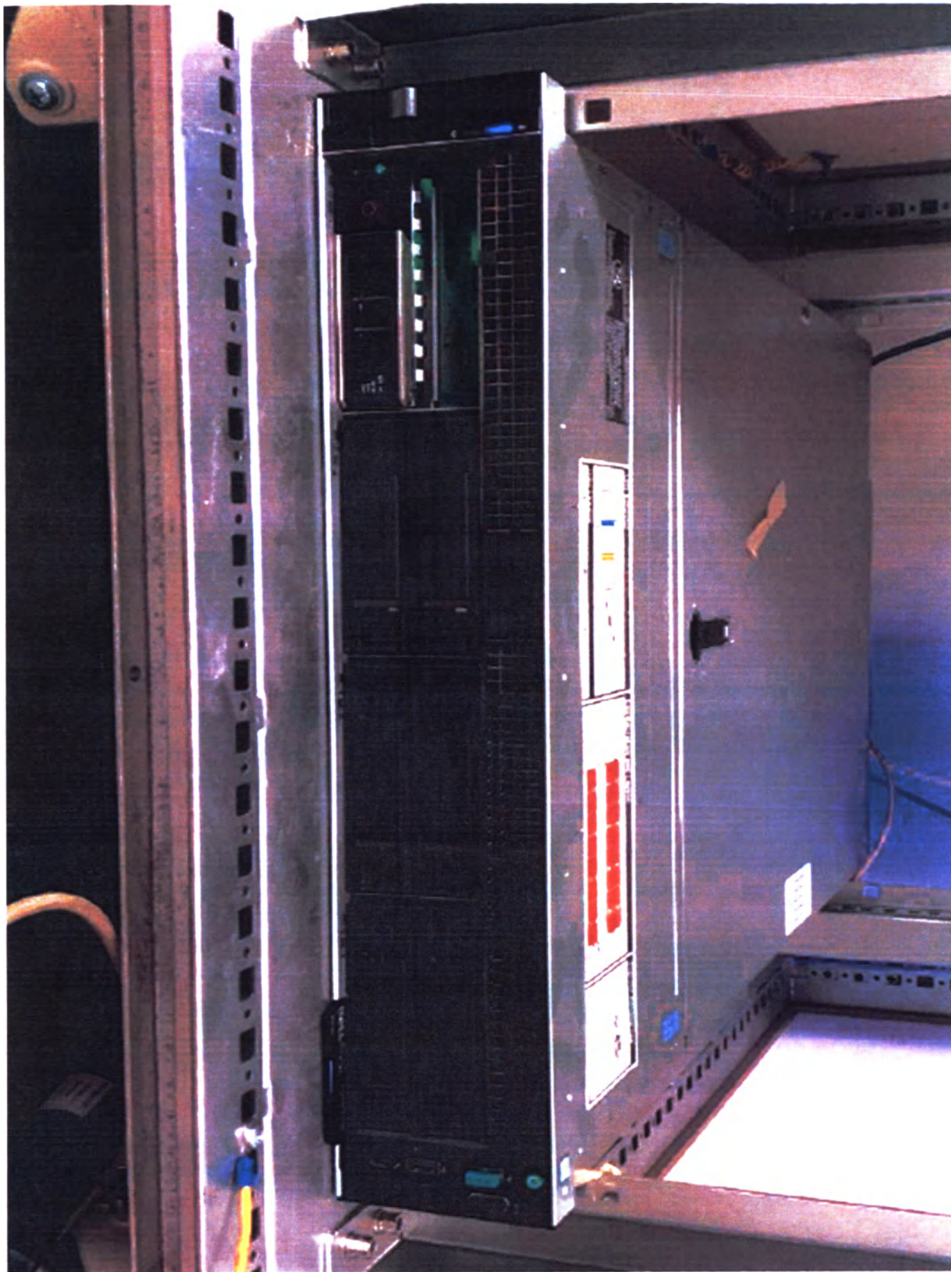
Вычислительный сервер для варианта исполнения uMR 780
