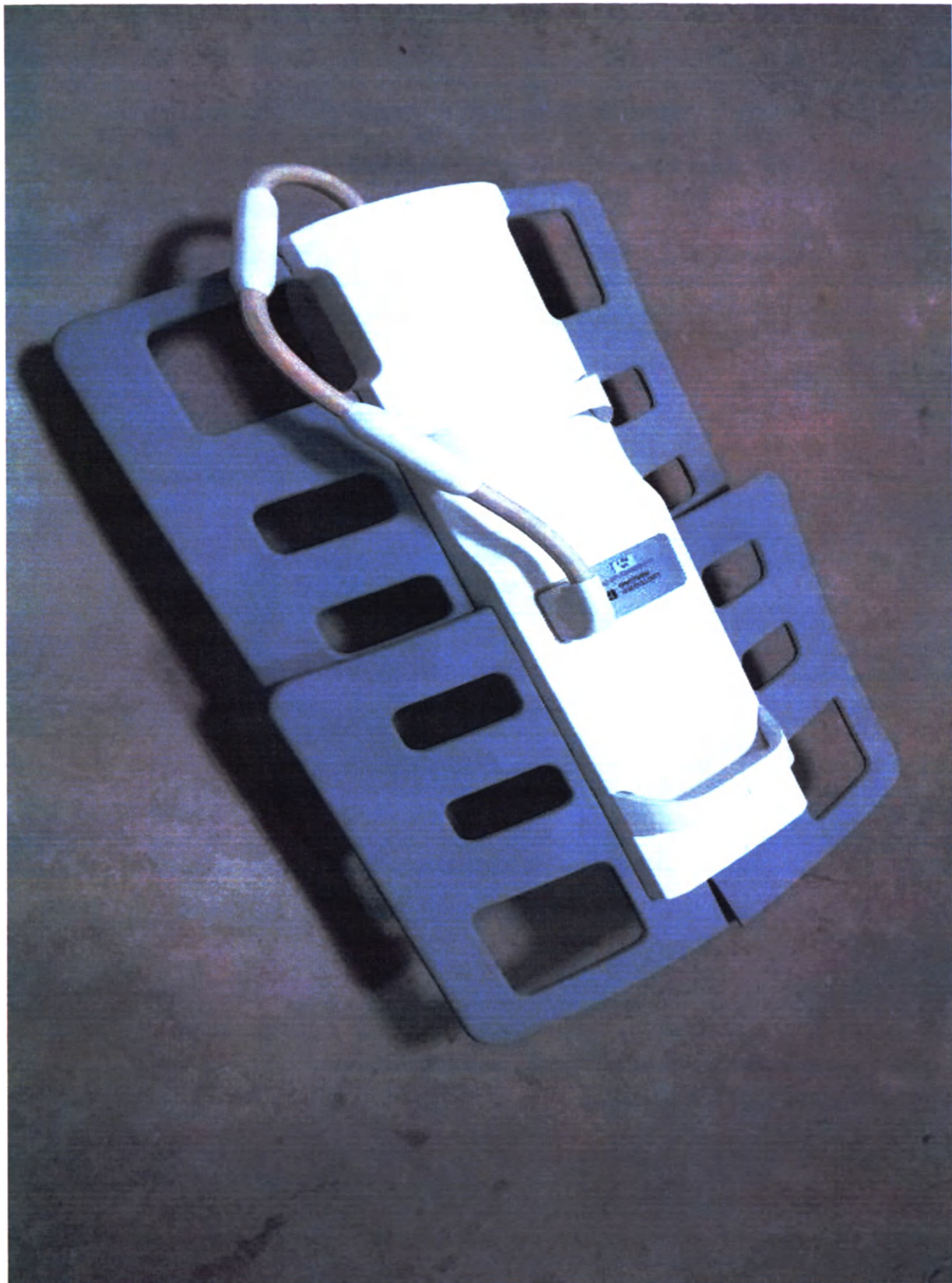
Катушка для нижних конечностей-24 для варианта исполнения uMR 570
