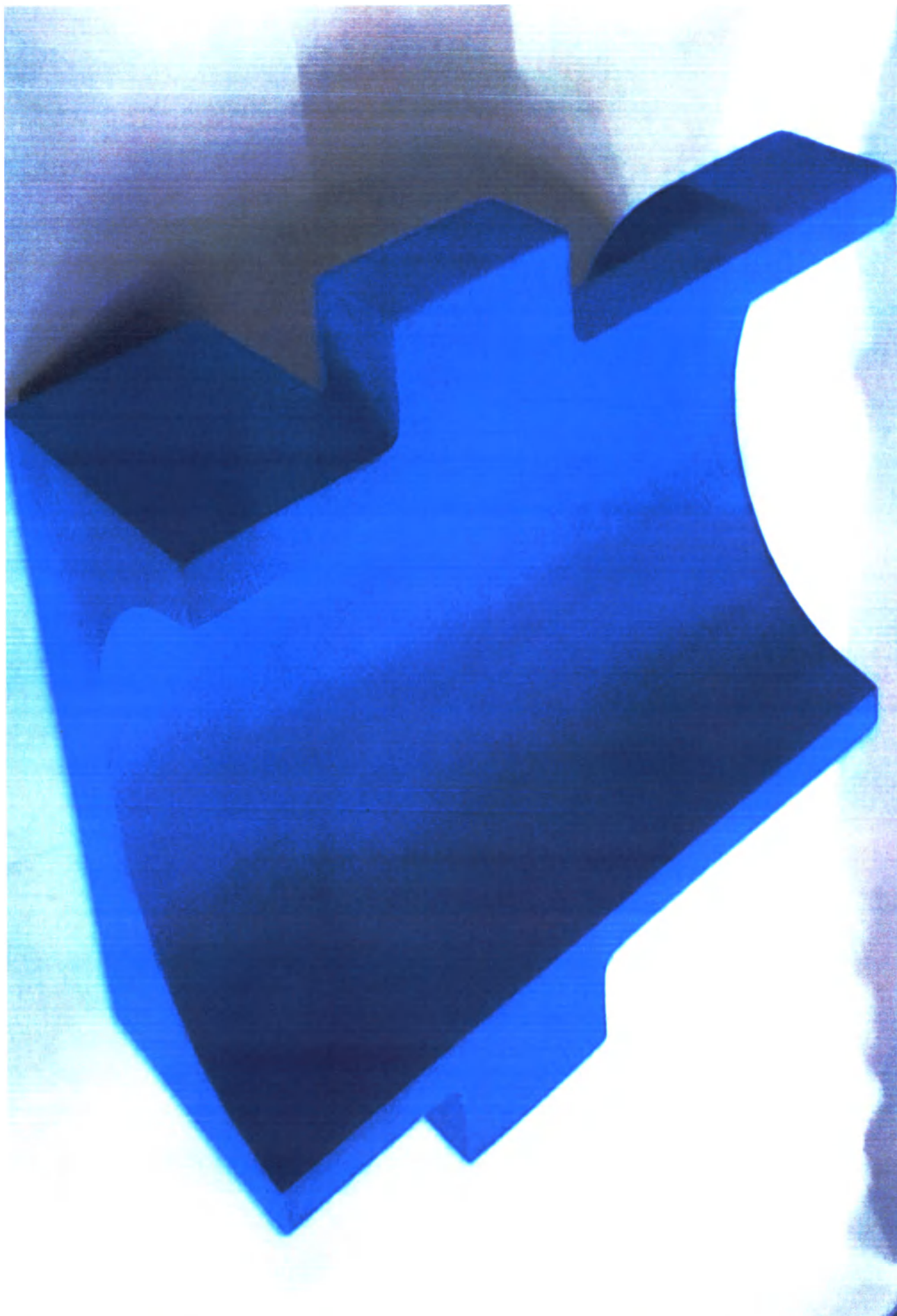
Поддон под водный фантом катушки для головы и шеи для вариантов исполнения uMR 580 и 588
