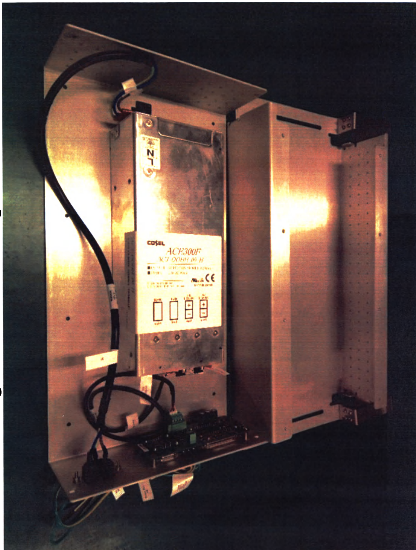
Блок питания для варианта исполнения uMR 780
