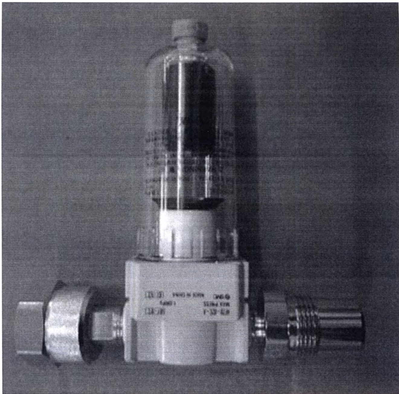
Фильтр - влагосорбник для блока ИВЛ (вход подачи кислорода)
