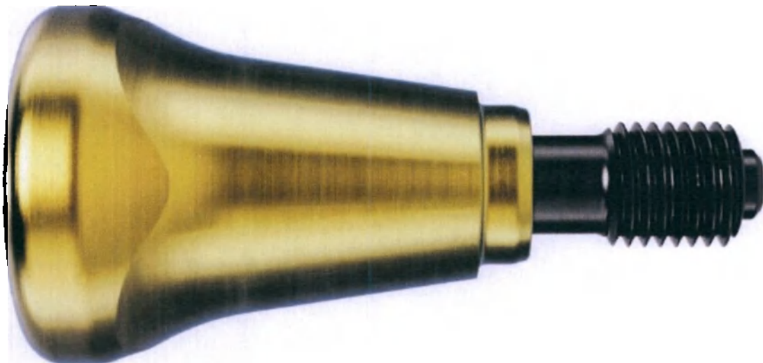
Формирователь десны Healing Abutment Nobel Biocare N1 TCC RP Ø4.5x7 мм
