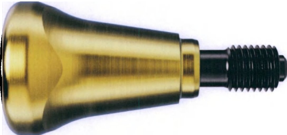
Формирователь десны Healing Abutment Nobel Biocare NI TCC RP Ø4.5x5 мм
