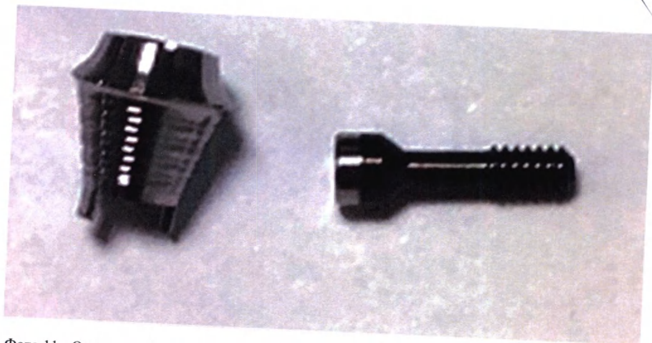
Фото 11 - Основание универсальное Universal Base Non-Engaging External Hex RP 1.0 мм с ВИНТОМ
