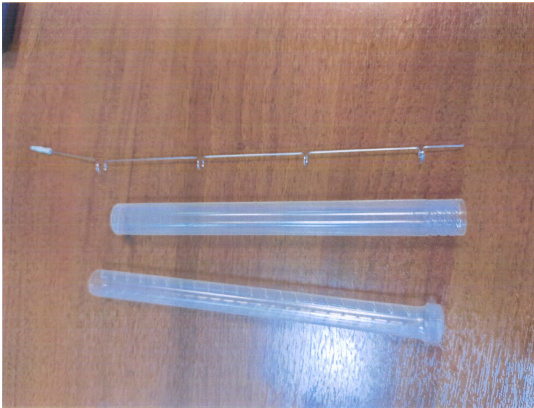
Фото 2.1 Распылитель ирригационный для электродвигателей ELAN 4 electro (1 шт./уп.), варианты исполнения: GA258SU, GA259SU, GA261SU, GA262SU, GA263SU, GA264SU, GA265SU, GA266SU, GA267SU, GA268SU, GA269SU - общий вид изделия
