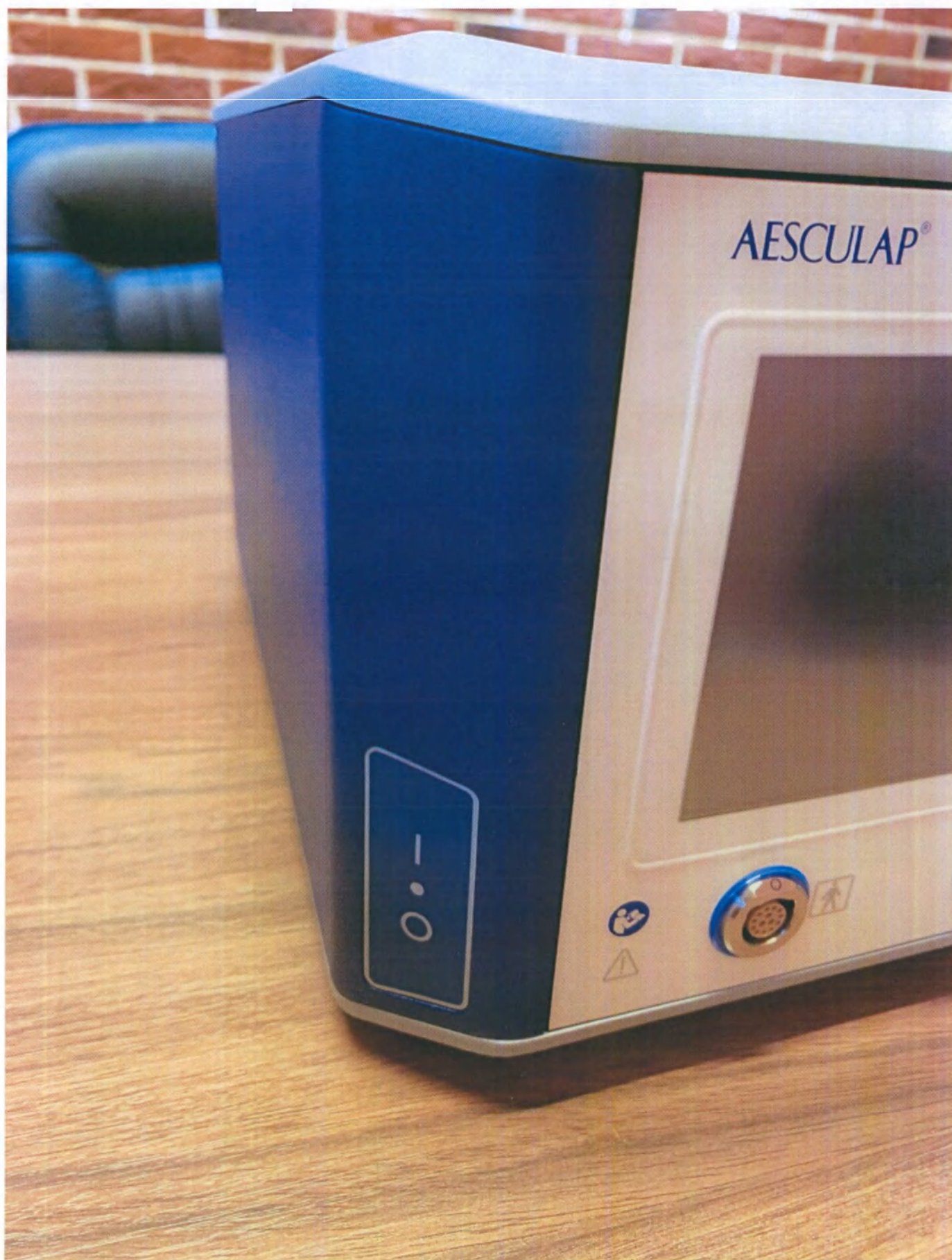
Фото 1.3 Блок управления хирургической моторной системой с питанием от сети ELAN 4 electro: GA800– вид изделия сбоку
