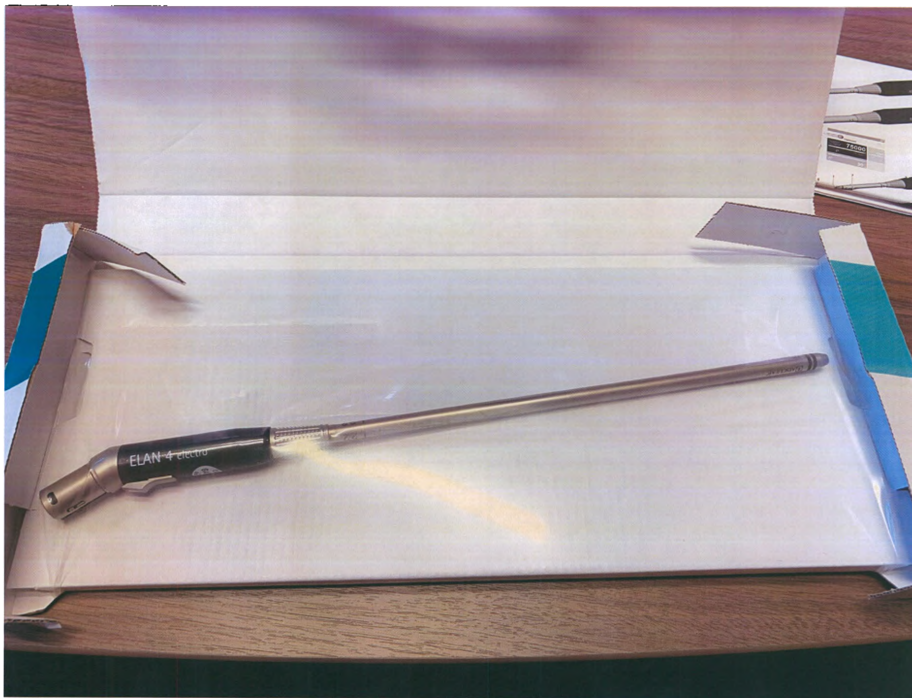
Фото 6.1 Дрель для бора с питанием от сети ELAN 4 electro, 2 кольца L22: GA869 – общий вид изделия.
