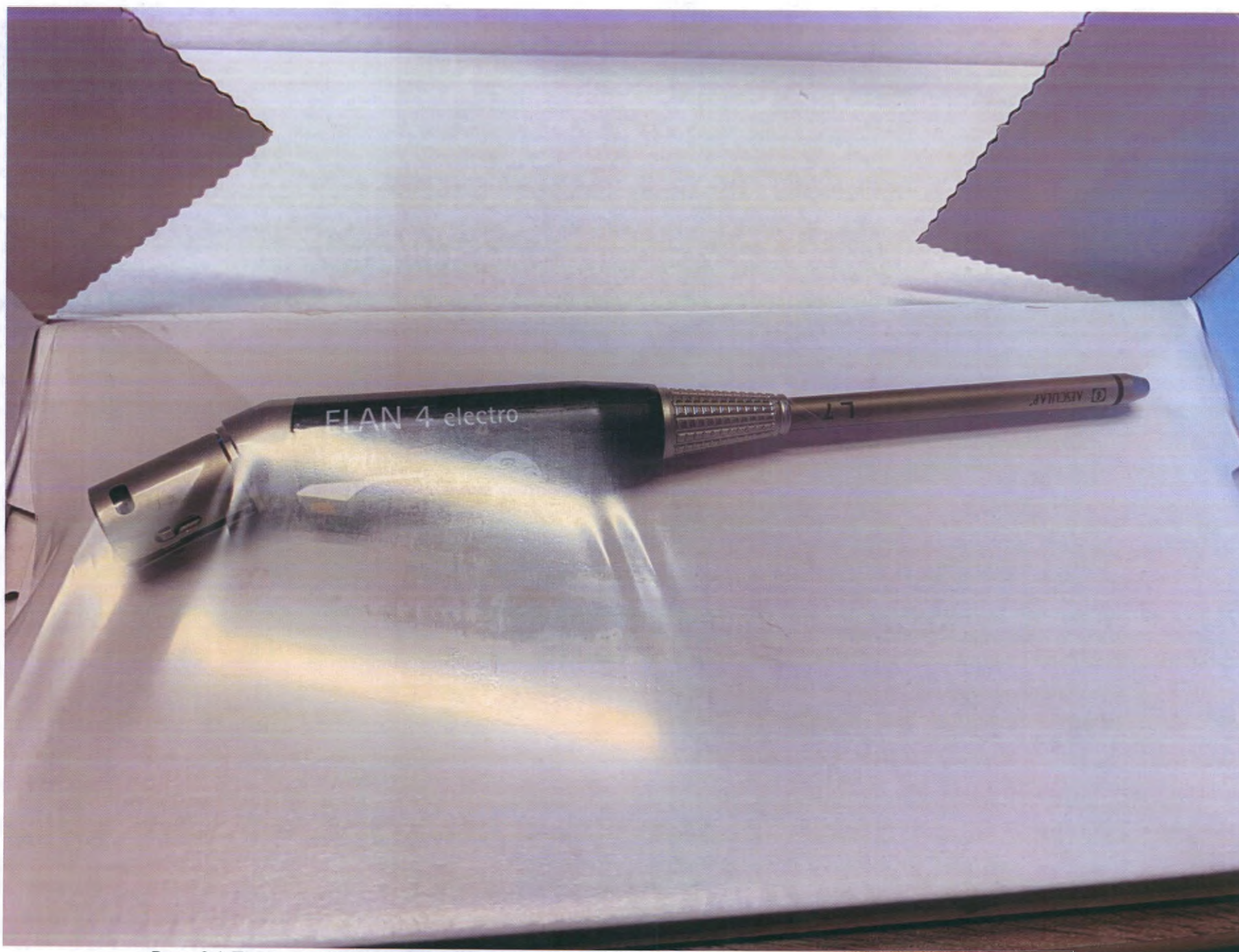
Фото 3.1 Дрель для бора с питанием от сети ELAN 4 electro, 1 кольцо L7: GA862 – общий вид изделия
