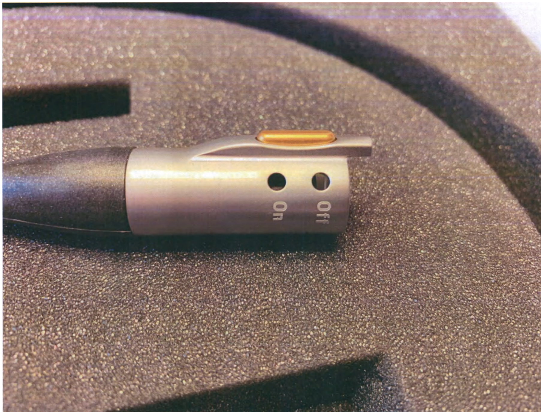
Фото 1.3 Кабель без рукоятки для управления электродвигателем хирургическим ELAN 4 electro: GA806- муфта для подключения рабочего элемента
