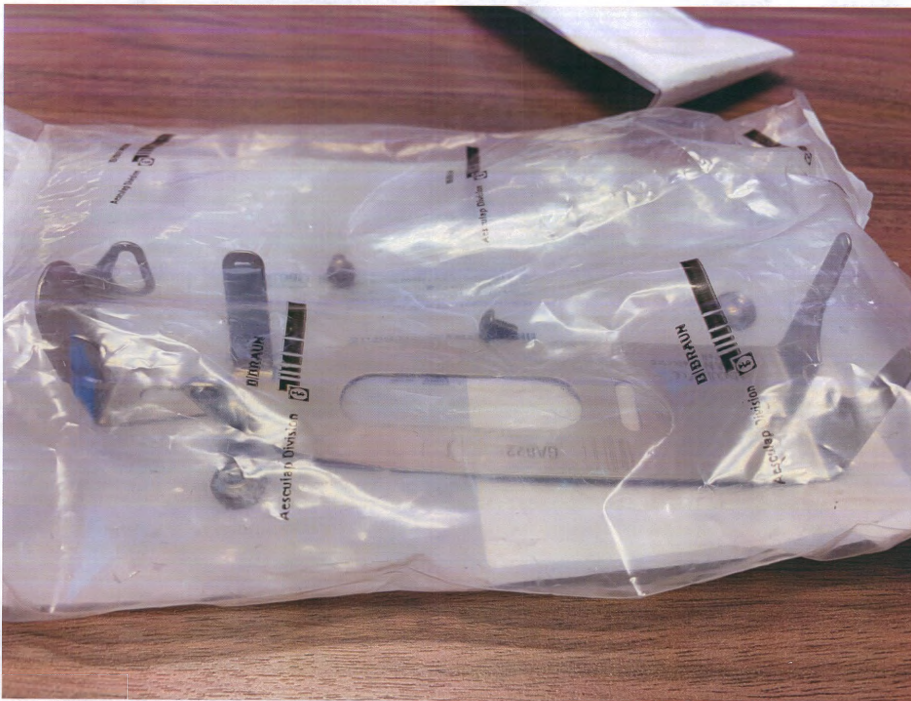
Фото 3.3 Фиксатор Eccos (1 шт./уп.), варианты исполнения: GB073R, GB076R , GB085R, GB082R, GB083R, GB088R, GB086R, GB087R, GB077R, GB072R – общий вид изделия.
