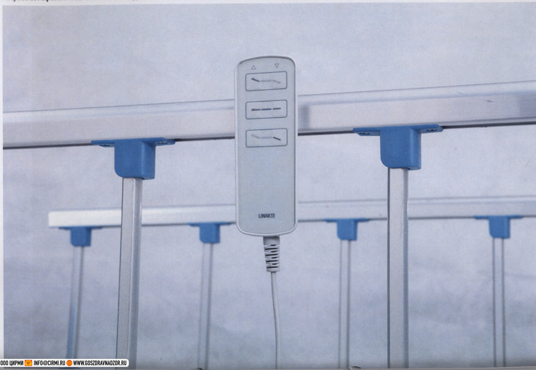
Рисунок 25: Кровать медицинская многофункциональная электрическая HECAI с принадлежностями, LS-EA 5013 (боковое ограждение)
