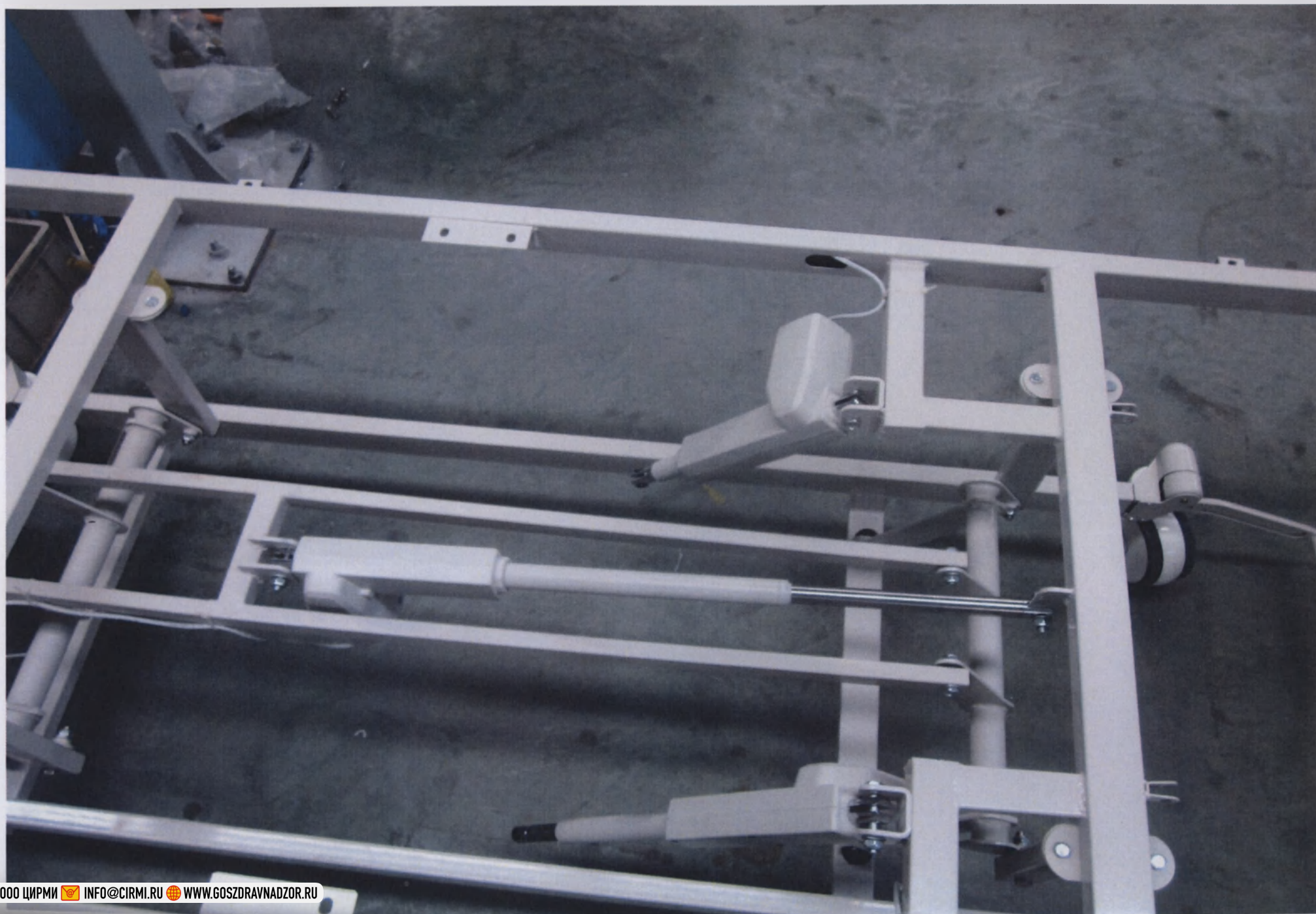
Рисунок 27: Кровать медицинская многофункциональная электрическая НЕСАІ с принадлежностями, LS-EA 013 (электропривод)
