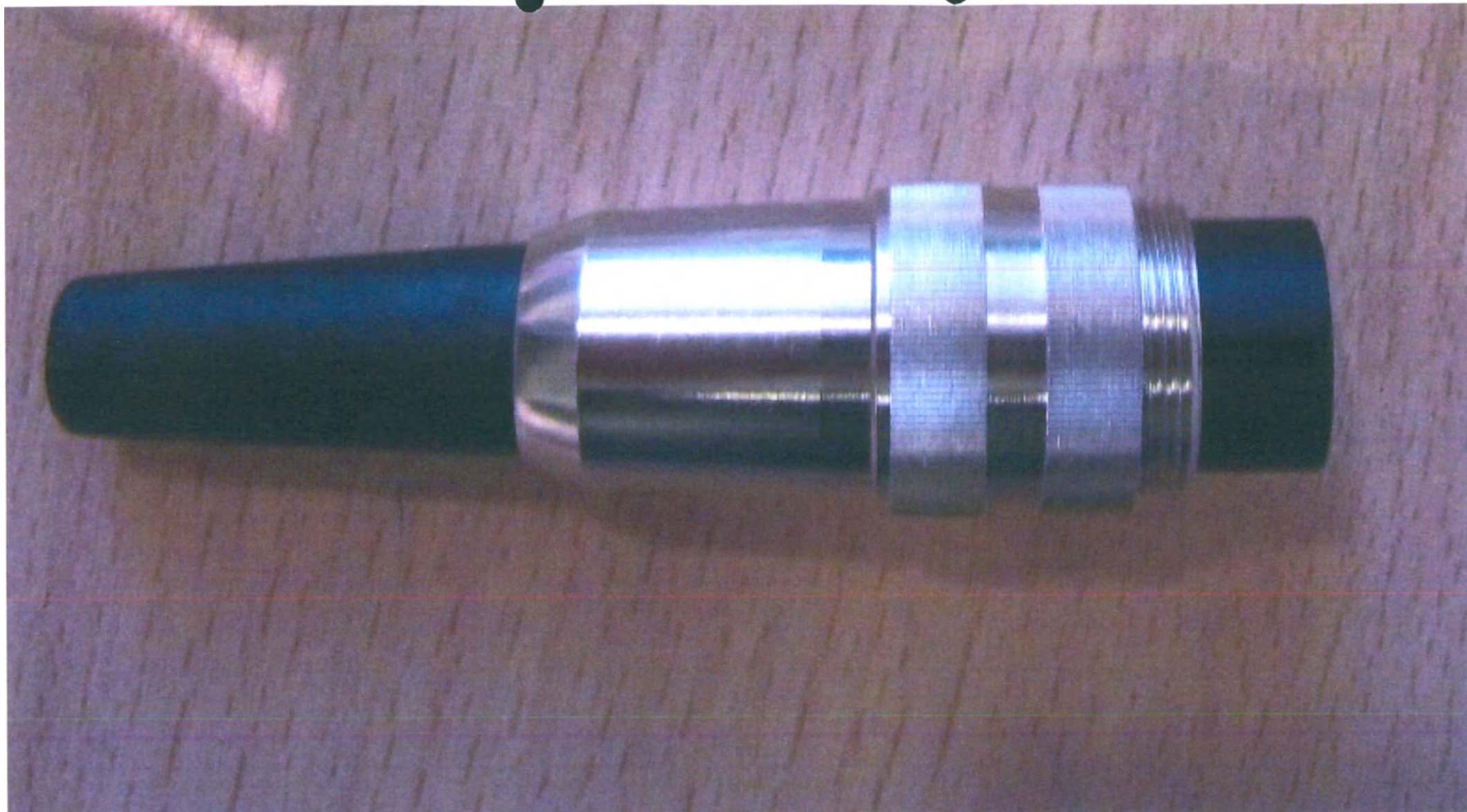
Аппарат медицинский лазерный с принадлежностями вариант исполнения «СмартКсайд 2 » (SmartXide 2 ). Разъем блокиратора двери
