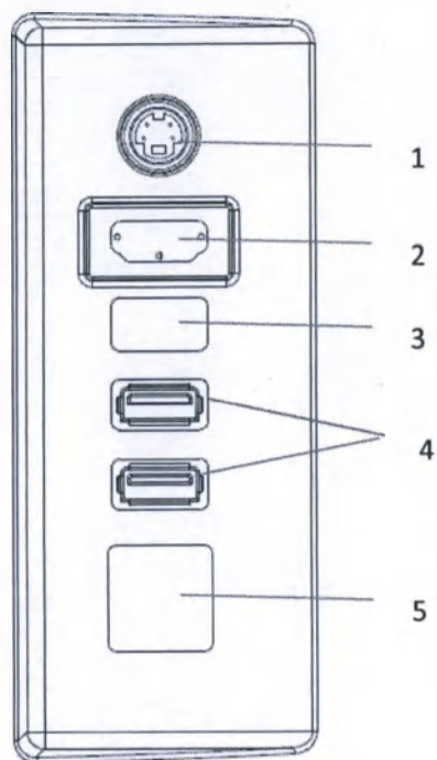
Рис. 6.2.6. Порты ввода-вывода
