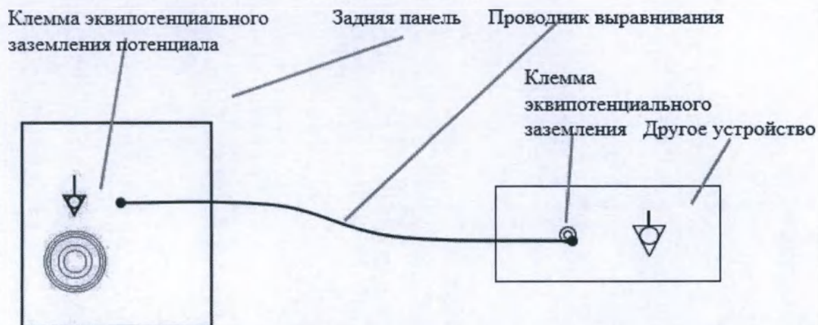
Рис. 6.2.7. Схема подключения эквипотенциального заземления
