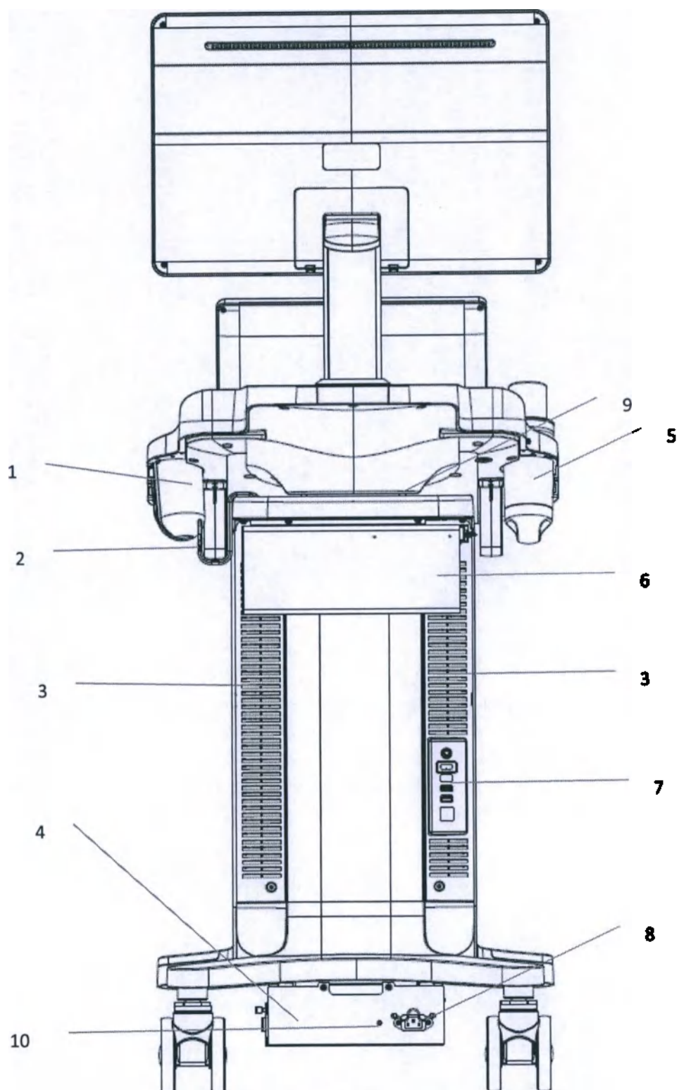
Рис. 6.2.5. Вид сзади
