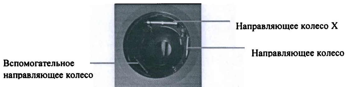
Рис. 16.3.2. Направляющие колеса X и Y и вспомогательное направляющее колесо
