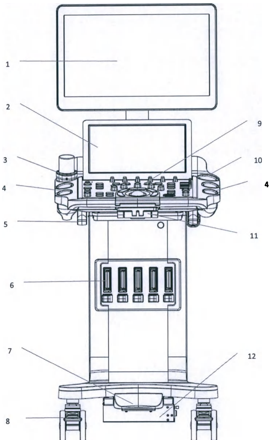
Рис. 6.1.1. Вид спереди
