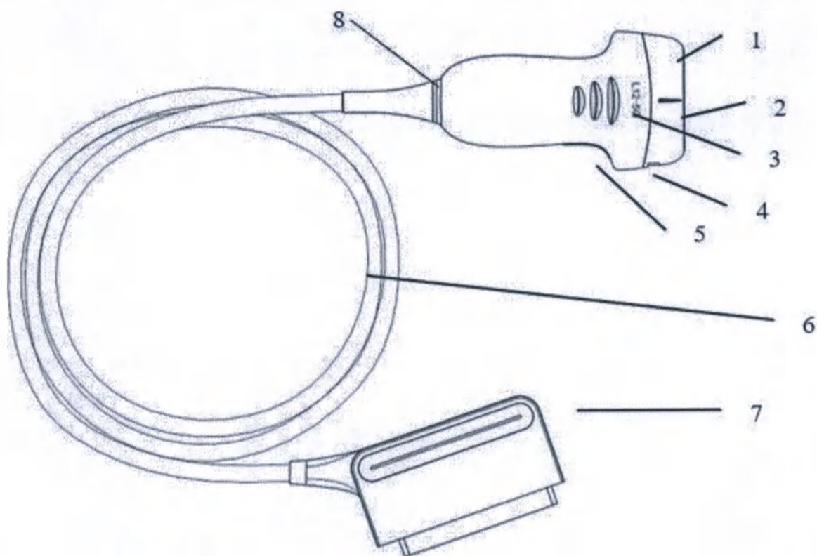
Рис. 9.2.1. Датчик линейный ультразвуковой L12-5Q
