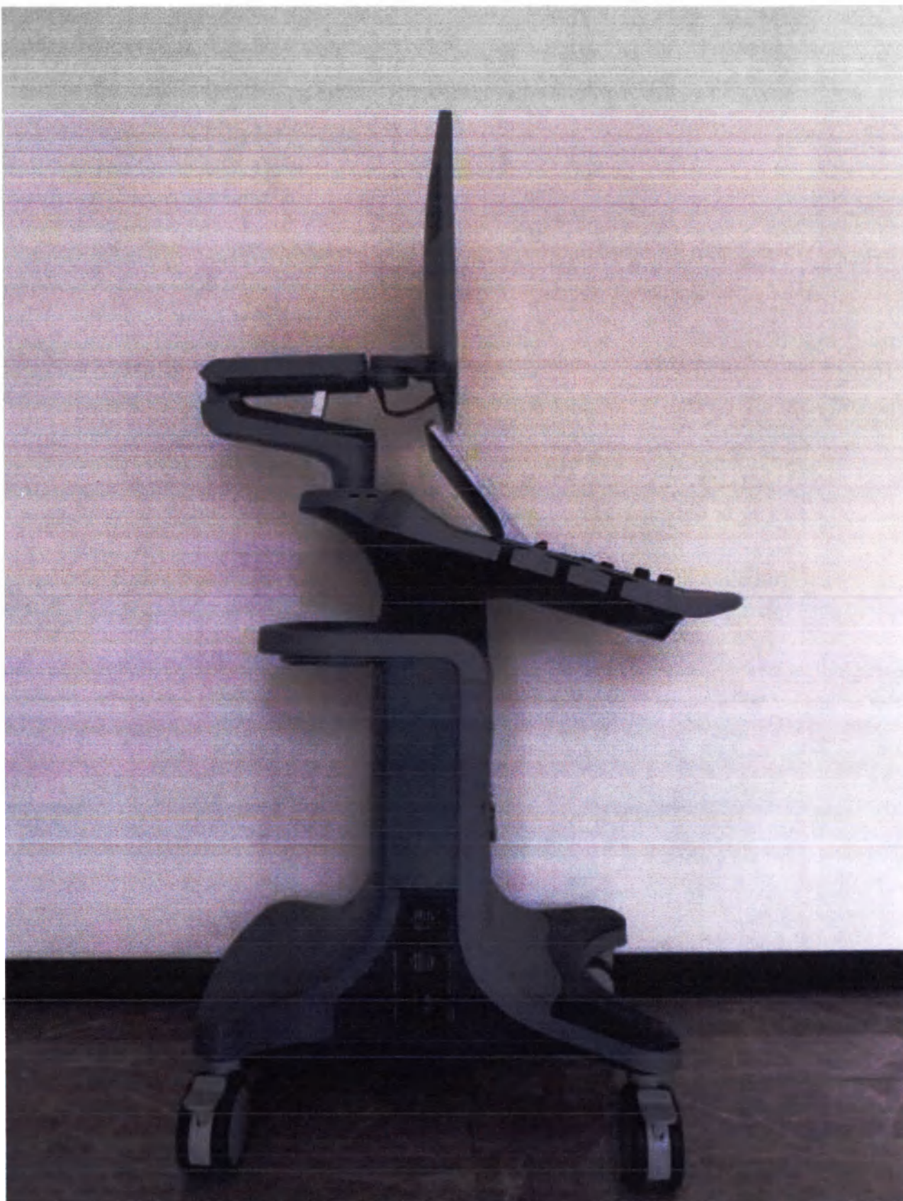
Внешний вид системы ультразвуковой Acclarix LX88 (вид слева)
