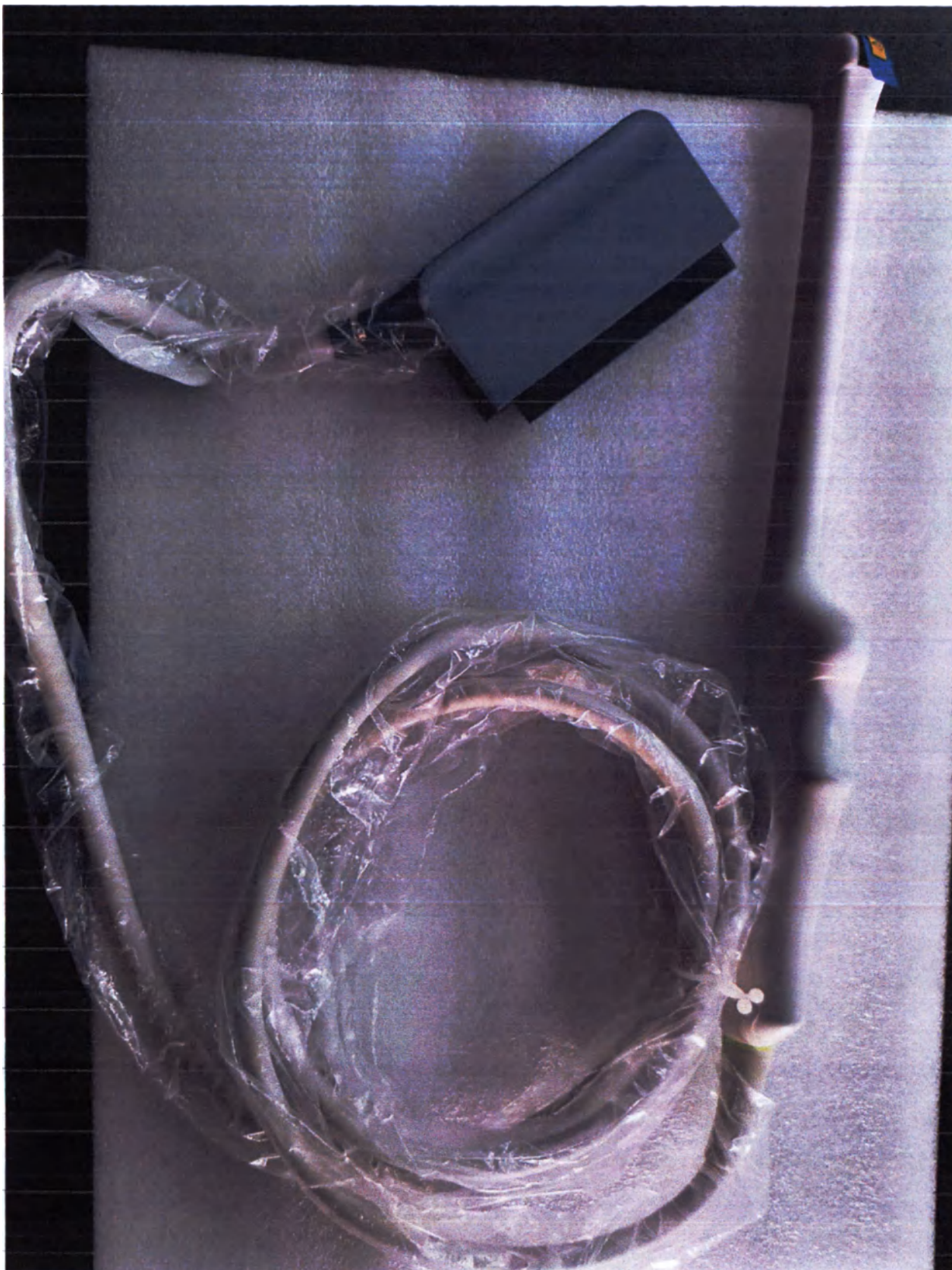
Датчик внутриспостной ультразвуковой E10-3HQ
