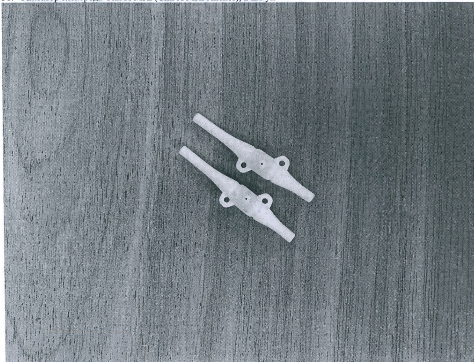
38. Фиксатор электрода Clik X MRI (Clik X MRI Anchor), 2 шт/уп
