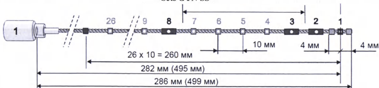
Наборы рентгеноконтрастных катетеров X-Ray Catheter Set с кодировкой 1-9, 10-18, 1-18, 19-30, длина 30 см, 50 см.
