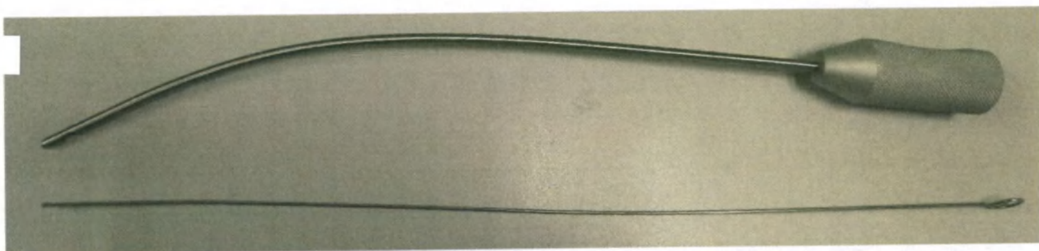
Канюля для липосакции аспирационная с окончанием в виде конуса, тремя центральными отверстиями и двумя боковыми прорезями, изогнутая, с соединением со шприцом катетерного типа 3G+2BC
