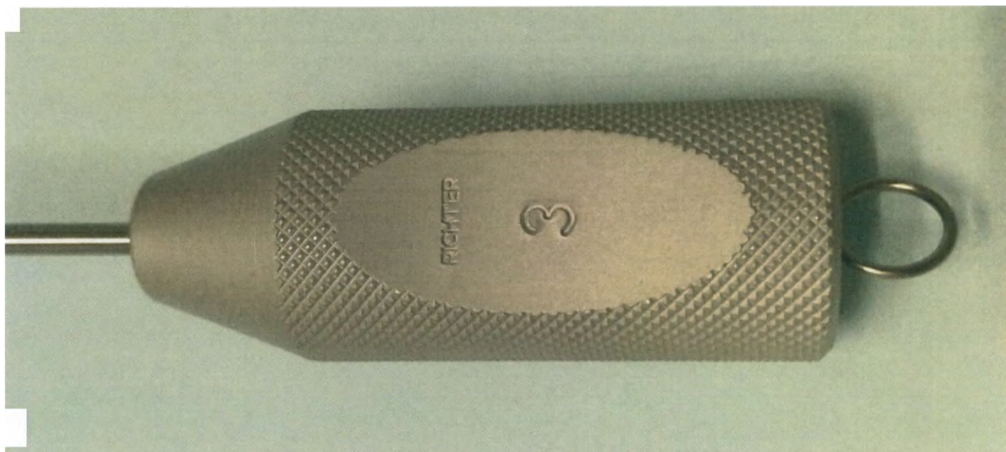
Канюля для липосакции аспирационная с плоским концом в виде шпателя, одним центральным отверстием и четырьмя боковыми прорезями, прямая, с соединением со шприцом катетерного типа РУР
