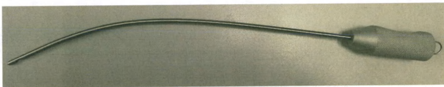
Канюля для липосакции аспирационная с окончником в виде конуса, двумя центральными отверстиями и двумя боковыми прорезями, изогнутая, с соединением со шприцом катетерного типа 3G+1BC
