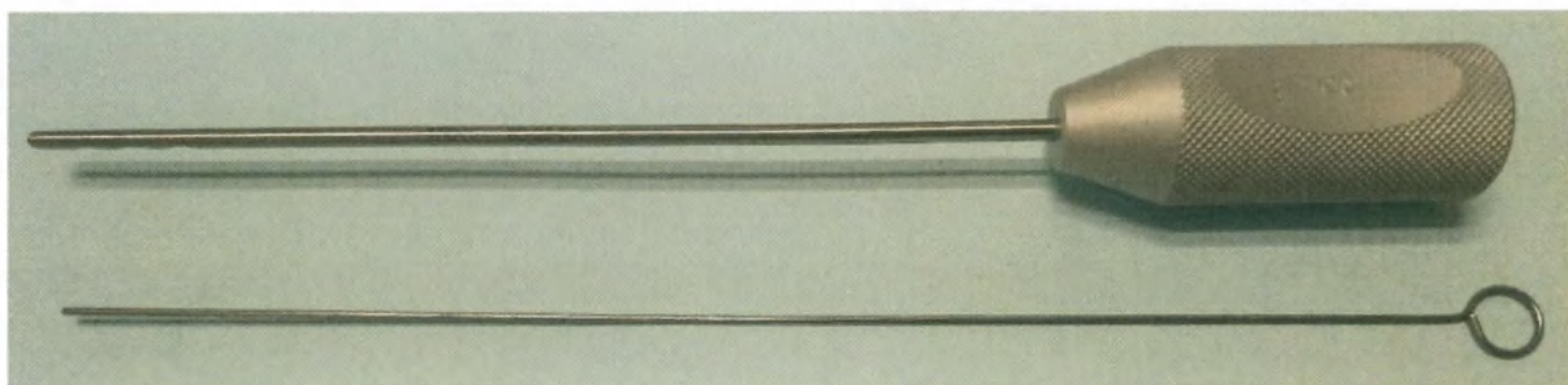
Канюля для липосакции аспирационная с концом типа "basket" и одним центральным отверстием, прямая, с соединением со шприцом катетерного типа BTDR
