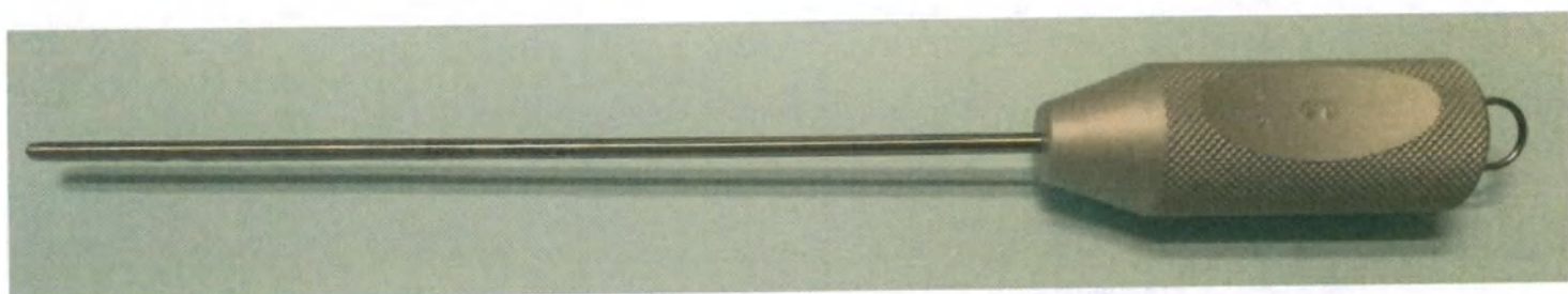
Канюля для липосакции аспирационная с 1 овальным отверстием и 3 овальными отверстиями на диаметрально противоположной поверхности, прямая, с соединением со шприцом катетерного типа 3HR+2RR
