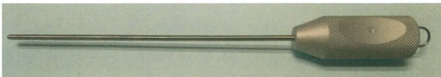
Канюля для липосакции аспирационная с тупым зауженным концом и 2 овальными отверстиями с разных сторон, прямая, с соединением со шприцом катетерного типа KCR
