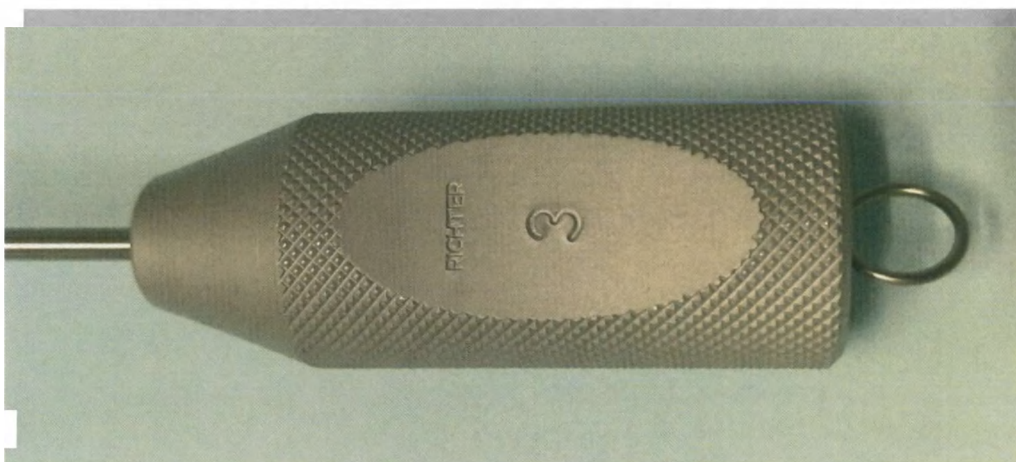
Канюля для липосакции аспирационная с концом типа "basket" и одним центральным отверстием, прямая, с соединением со шприцом катетерного типа BTDR
