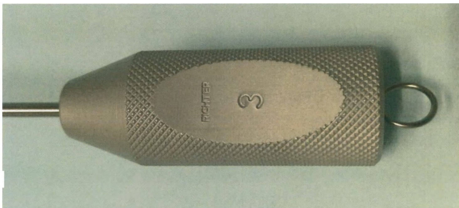
Канюля для липосакции аспирационная с тупым зауженным концом и 2 овальными отверстиями с разных сторон, прямая, с соединением со шприцом катетерного типа KCR
