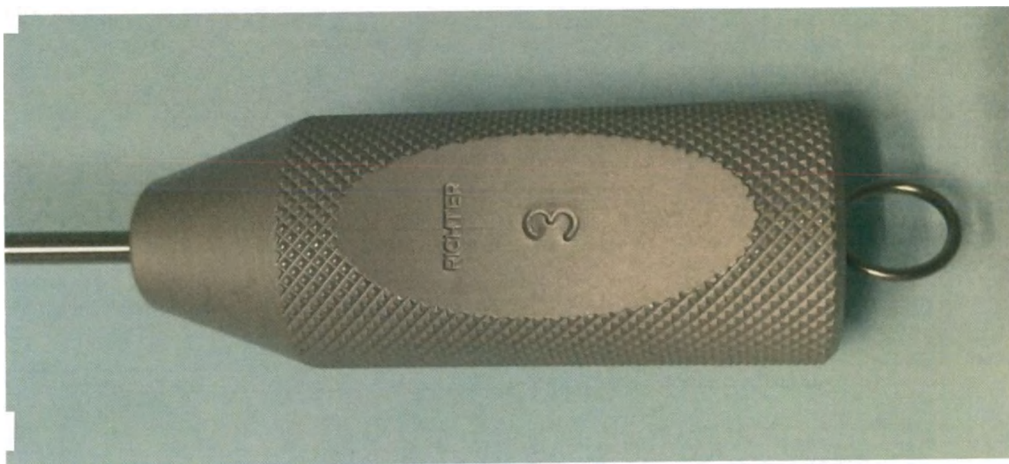
Канюля для липосакции аспирационная с окончником в виде конуса, двумя центральными отверстиями и двумя боковыми прорезями, угловая, с соединением со шприцом катетерного типа 3G+1BB
