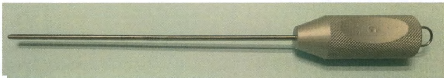
Канюля для липосакции аспирационная с плоским концом в виде шпателя, одним центральным отверстием и четырьмя боковыми прорезями, прямая, с соединением со шприцом катетерного типа PYR
