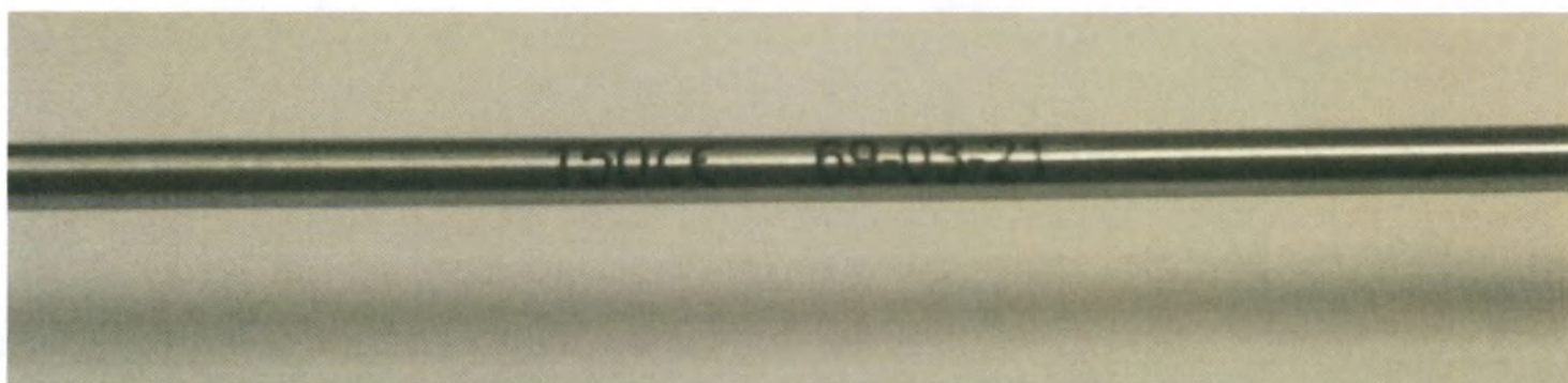
Канюля для липосакции аспирационная с 5 боковыми прорезями по диаметру, изогнутая, с соединением со шприцом катетерного типа 5ALC
