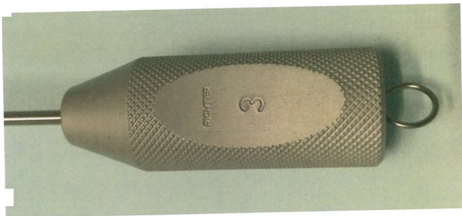
Канюля для липосакции аспирационная с 6 отверстиями по диаметру, прямая, с соединением со шприцом катетерного типа LeR
