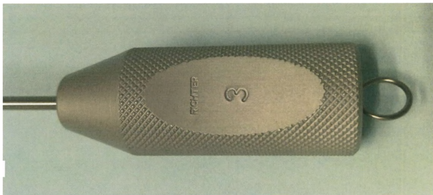
Канюля для липосакции аспирационная с 1 овальным отверстием и зауженным кончиком, прямая, с соединением со шприцом катетерного типа STRR
