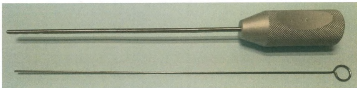
Канюля для липосакции аспирационная с 15 круглыми отверстиями, прямая, с соединением с шприцом катетерного типа ЗНМФР
