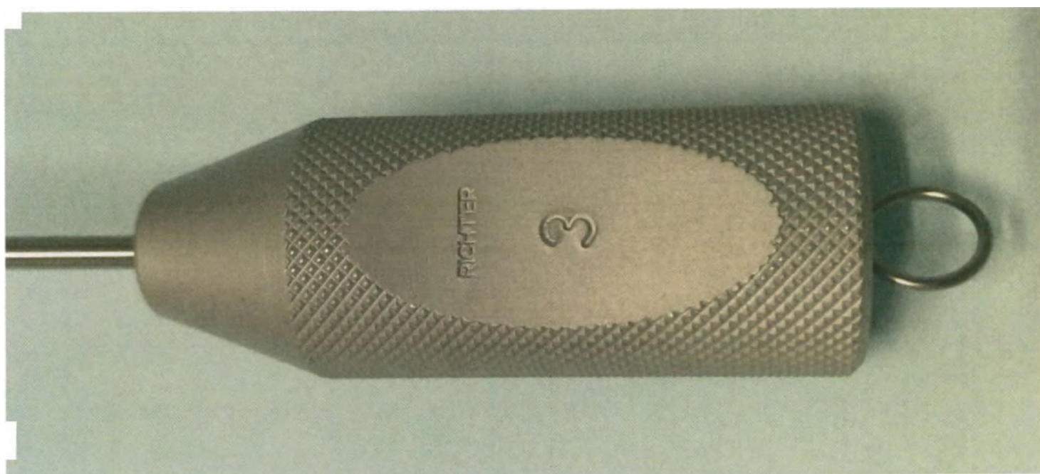
Канюля для липосакции аспирационная с окончанием в виде конуса, четыремa центральными отверстиями и двумя боковыми прорезями, прямая, с соединением со шприцом катетерного типа 3G+3BR
