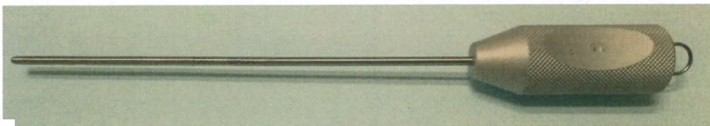
Канюля для липосакции аспирационная с плоским концом в виде шпателя, одним центральным отверстием и двумя боковыми прорезями, прямая, с соединением со шприцом катетерного типа P3GR
