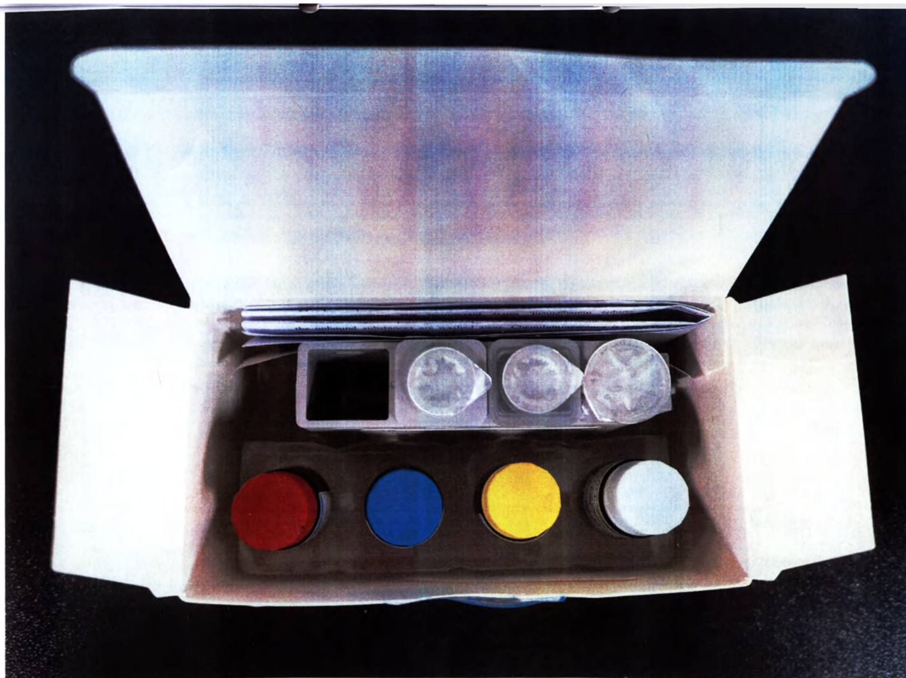
Общий вид медицинского изделия (Набор реагентов для количественного определения нейронспецифической енолазы электрохемилюминесцентным методом на анализаторах ECL для диагностики in vitro (Neuronen-Spezifische Enolase (eCLIA) / NSE))
