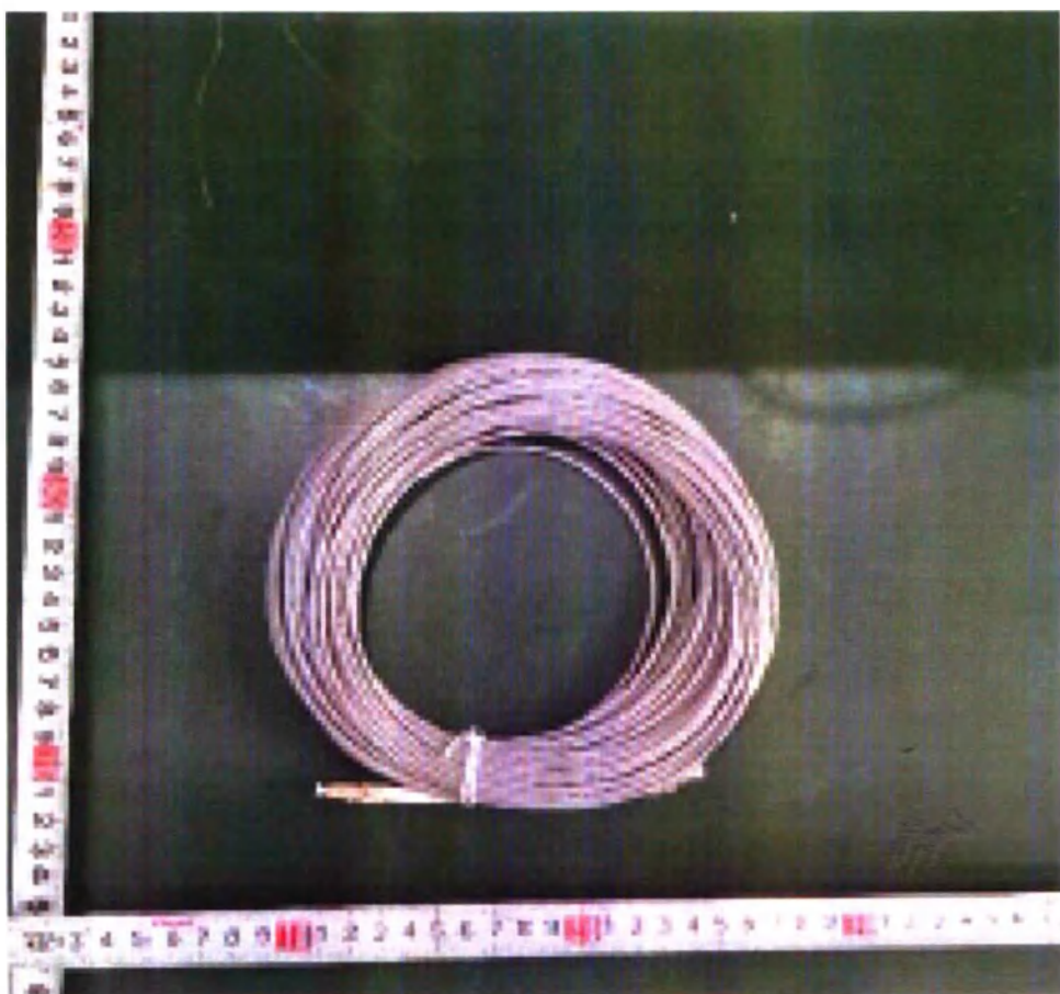
Фото 18 Кабель волоконно-оптический для передачи данных от Гентри к консоли оператора
