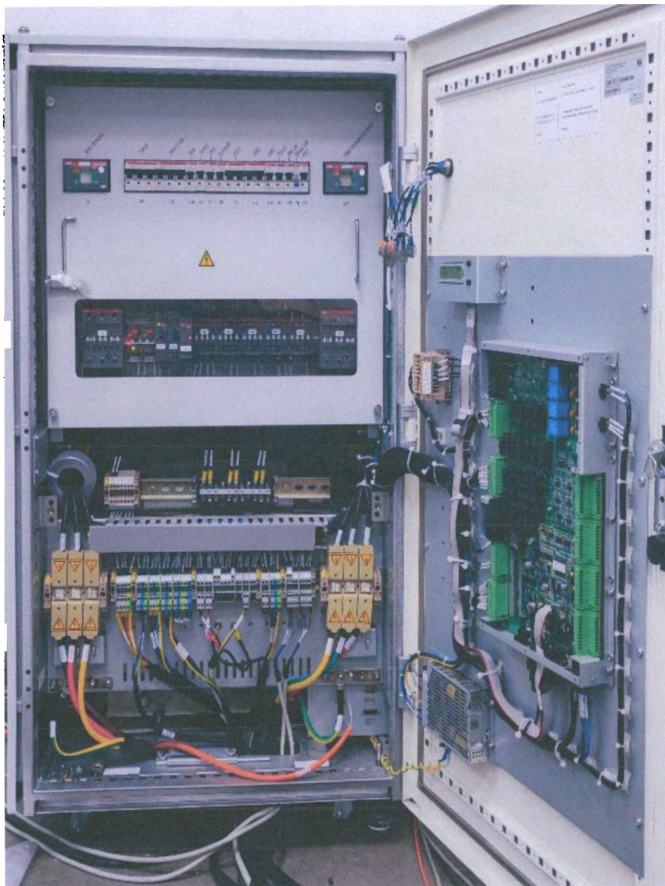
Шкаф высоковольтного питания для варианта исполнения uMI 550
