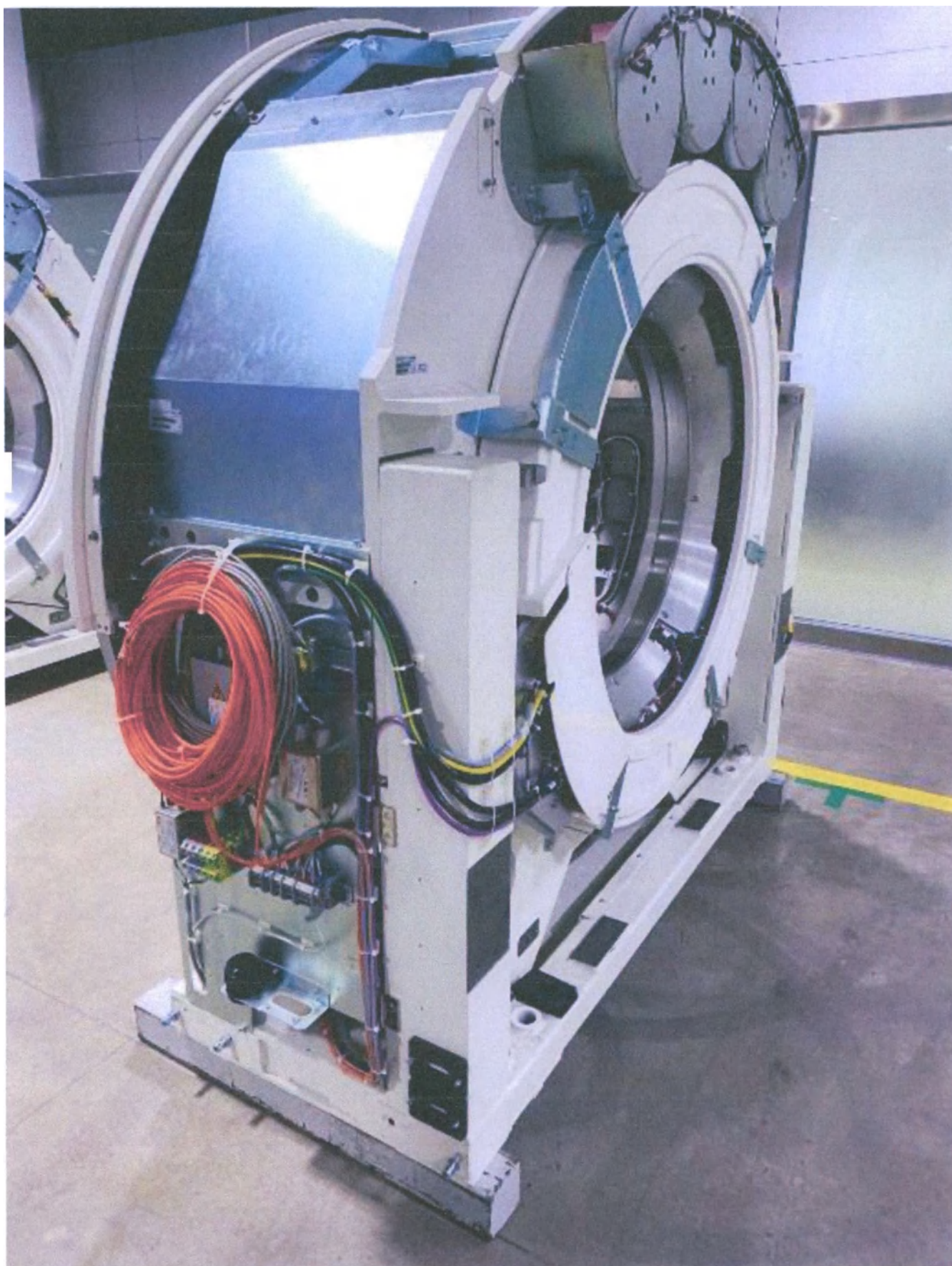
КТ-гептри для варианта исполнения иМІ 780
