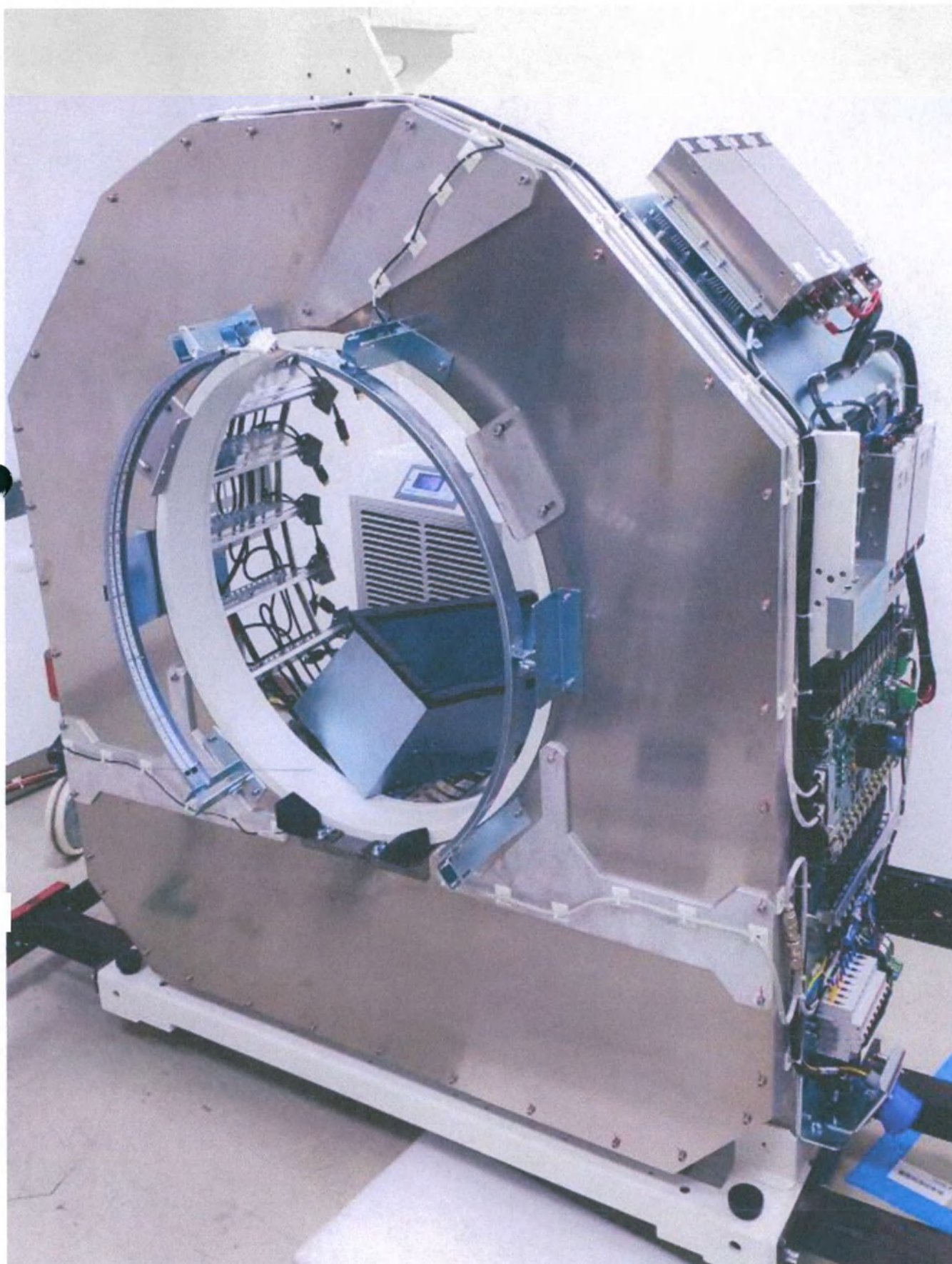
ПЭТ-генри для варианта исполнения uMI 550
