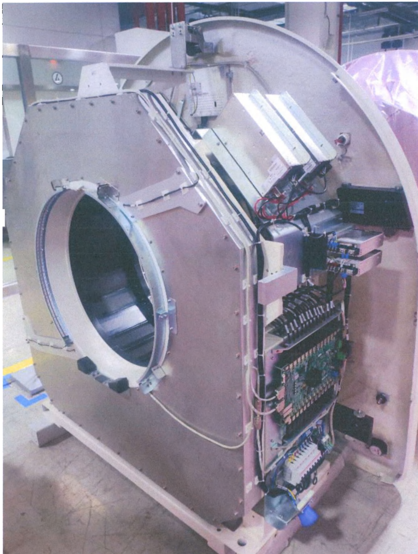
ПЭТ-гептри для варианта исполнения шМІ 780
