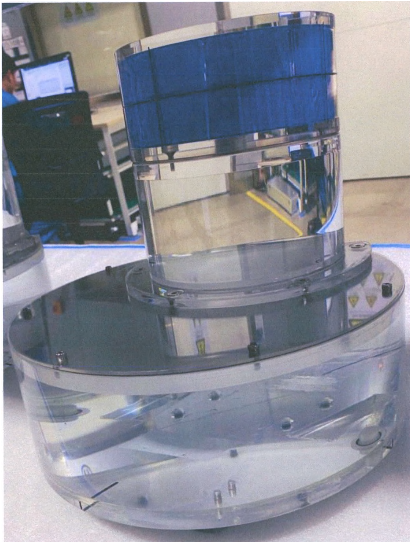
Фантом системный U16 для варианта исполнения uMI 550
