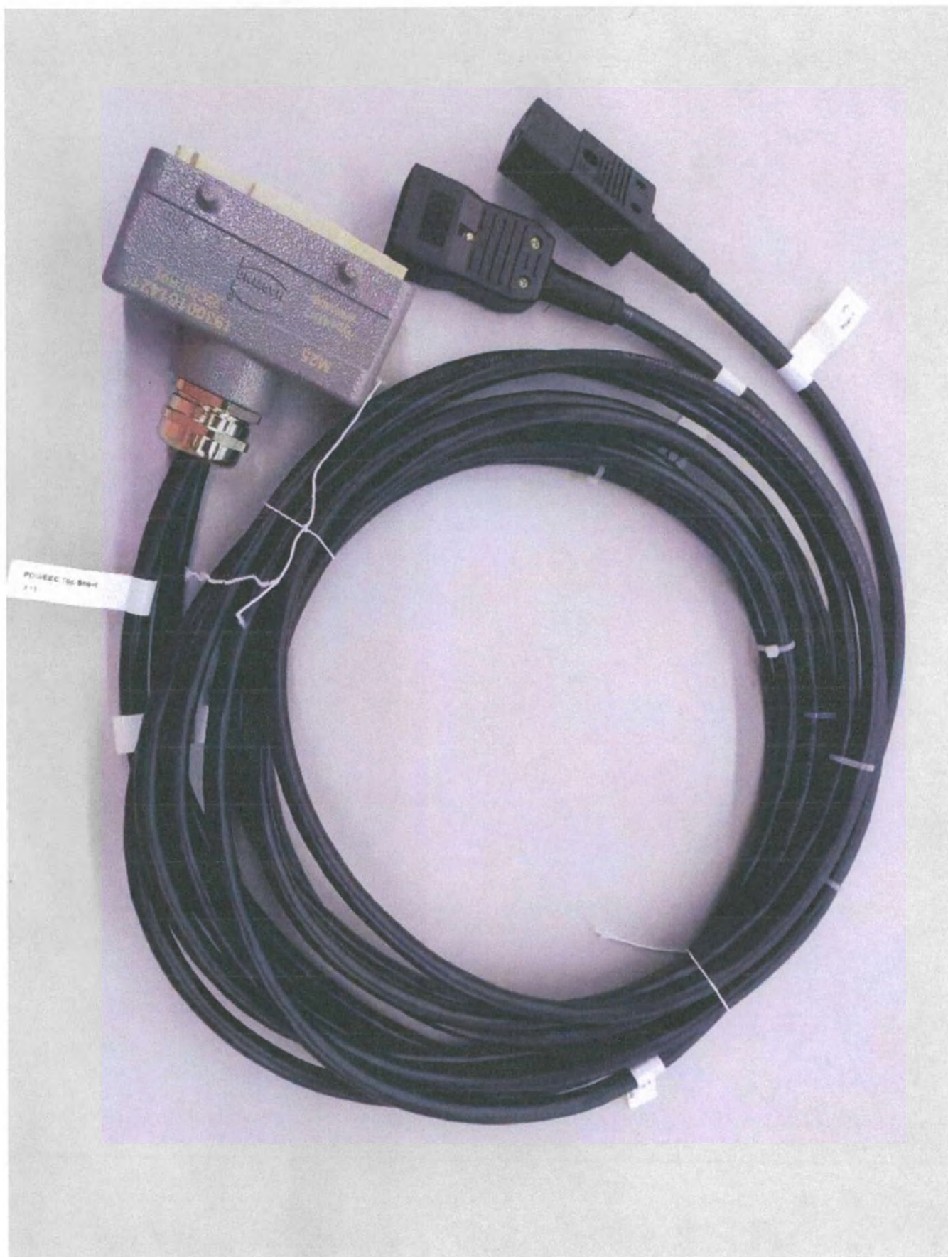
Кабель UPS (при необходимости) для варианта исполнения uMI 550
