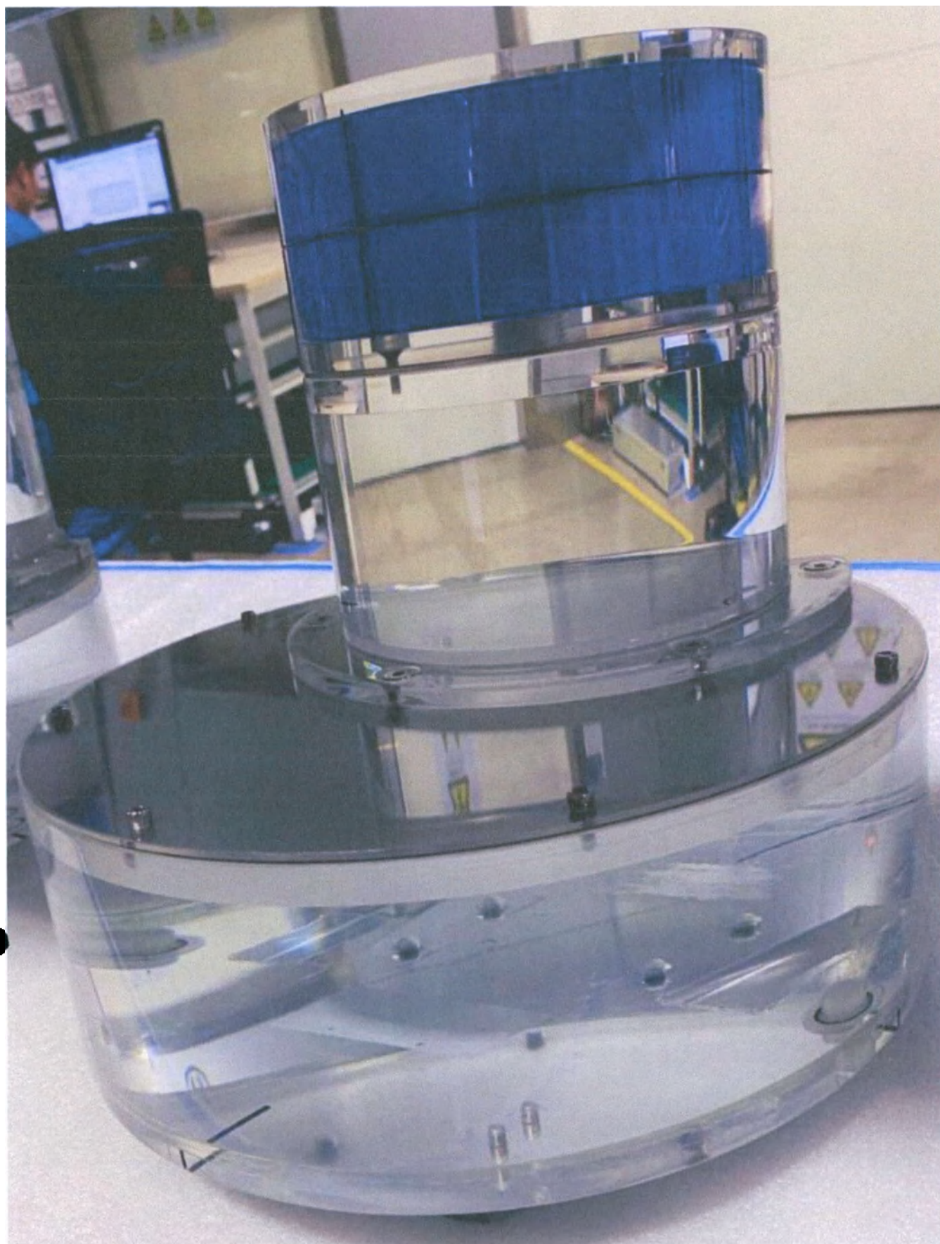
Фантом системный U16 для варианта исполнения uMI 780
