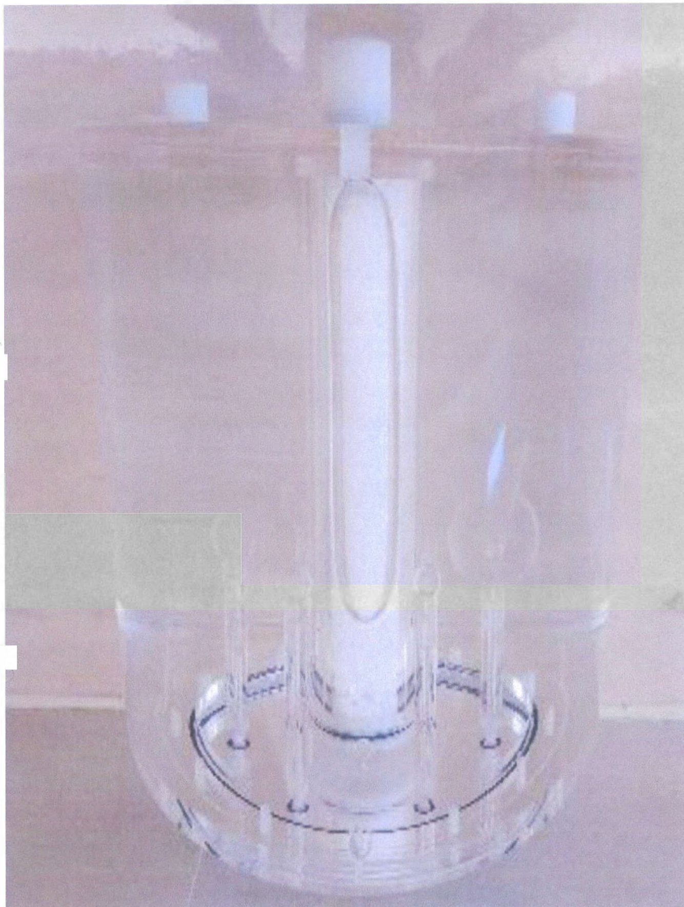
Фантом для теста NEMA (при необходимости) для варианта исполнения uMI 780
