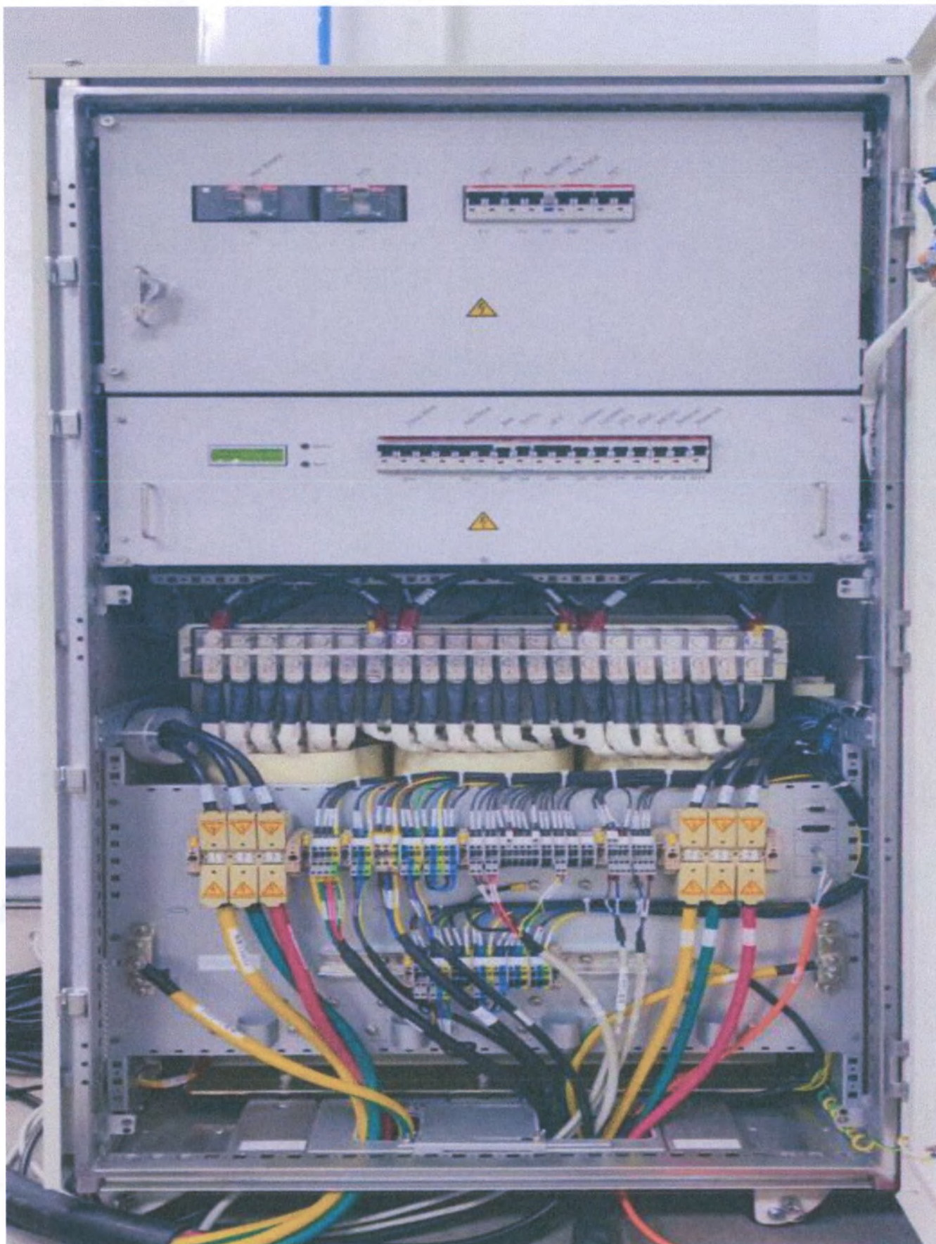
Шкаф высоковольтного питания для варианта исполнения uMI 780
