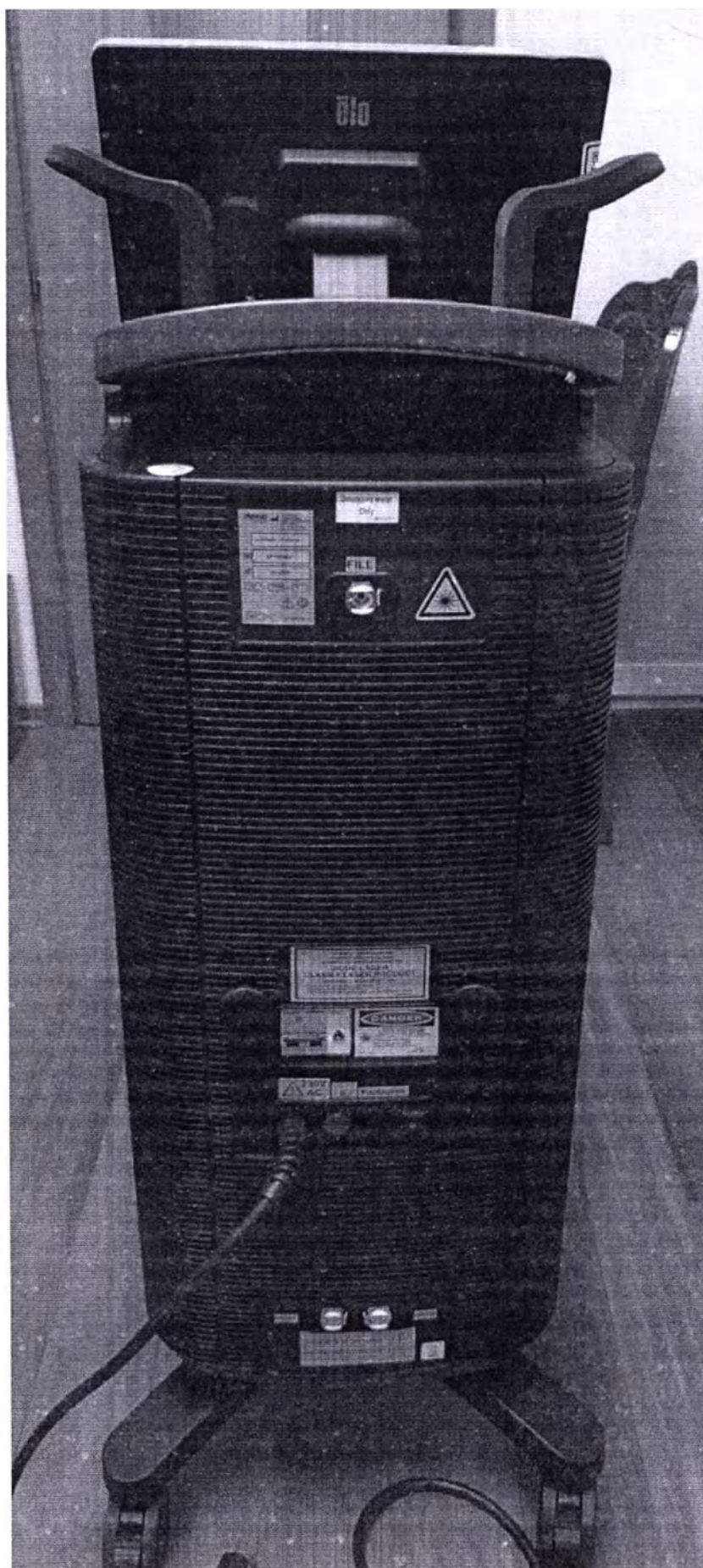
Аппарат лазерный многофункциональный Soprano Titanium (вид сзади)
