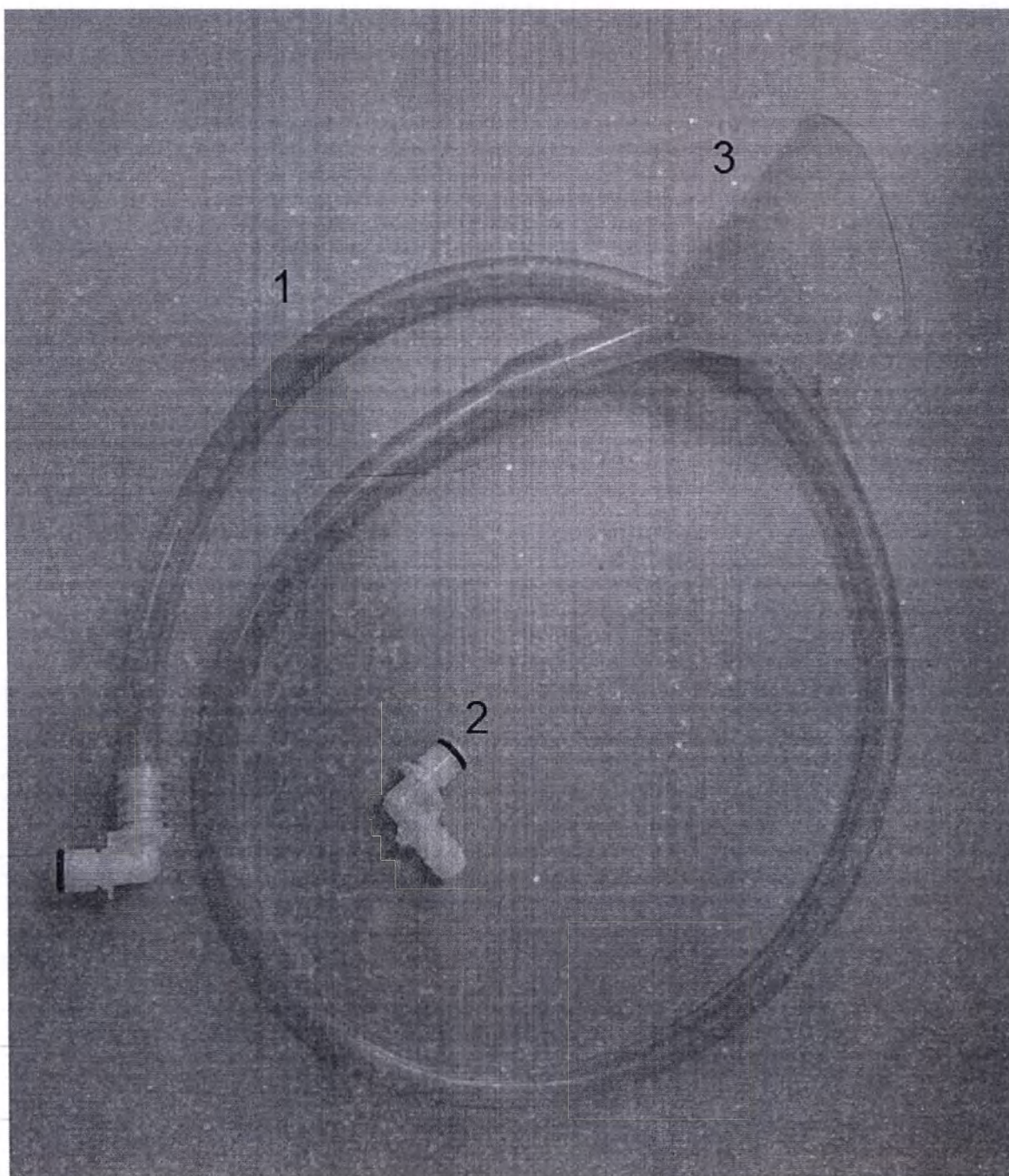
Комплект для заливки воды в систему охлаждения: 1 – Шланг, 2 – Втулка соединительная угловая для шланга, 3 – Воронка.
