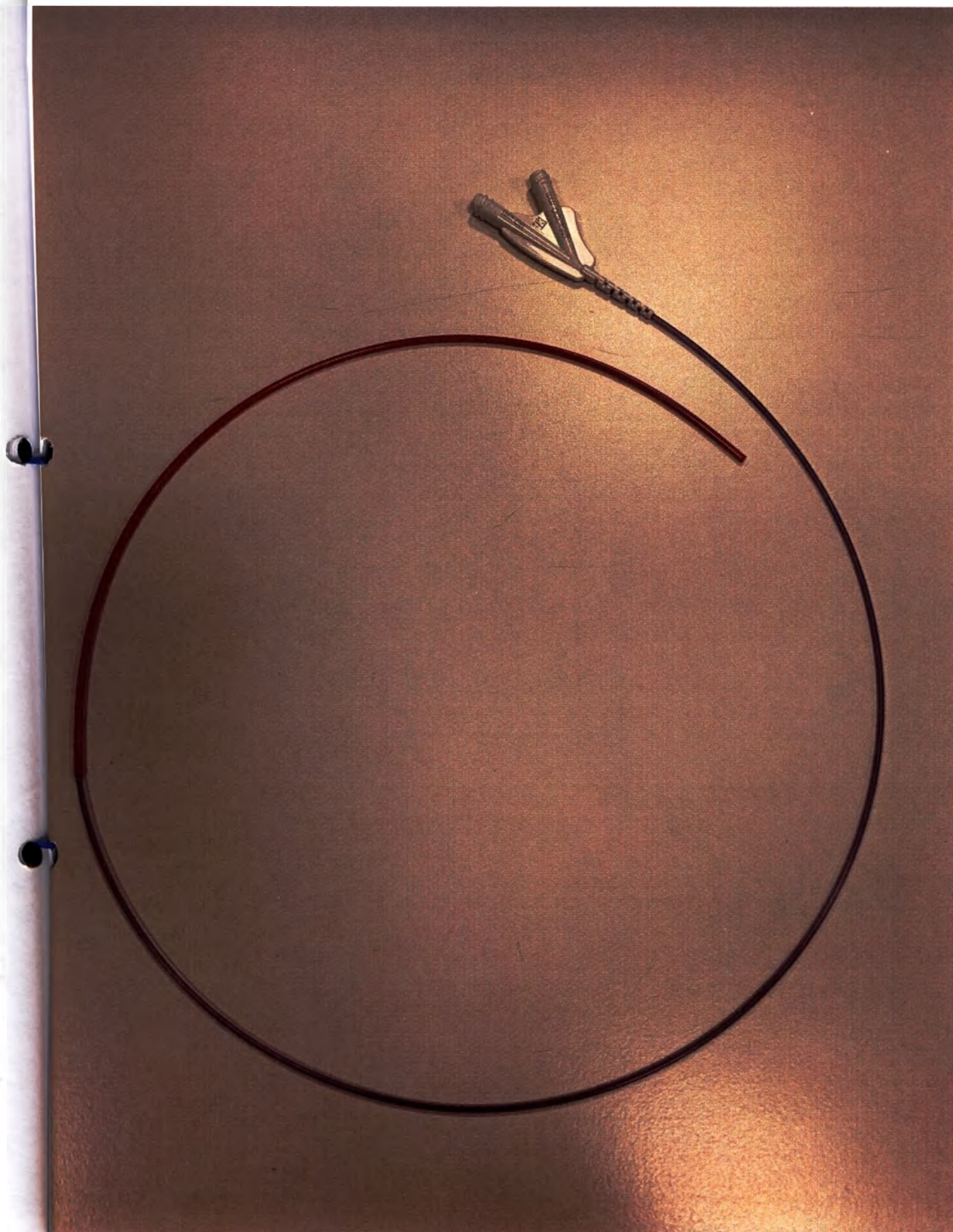
Рисунок 11. Катетер баллонный для ЧТА Admiral Xtreme: номинальный диаметр баллона (мм) 5.0; номинальная длина баллона (мм) 300; рабочая длина катетера (см) 80
