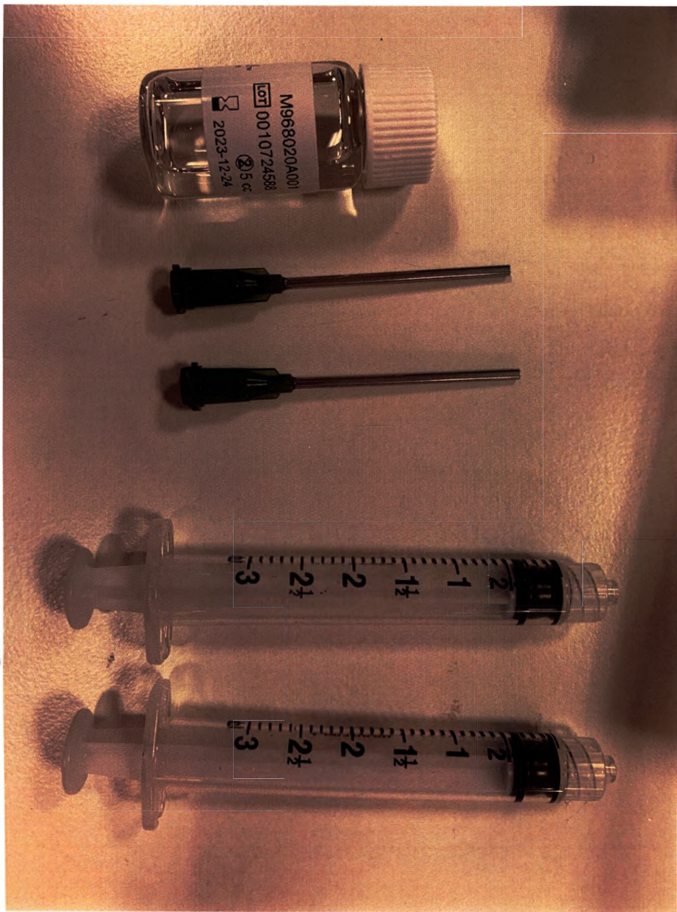
Рисунок 6. Флакон биологического клея VenaSeal, 5 мл - 1 шт., Наконечник-дозатор - 2 шт., Шприц, 3 мл - 2 шт.
