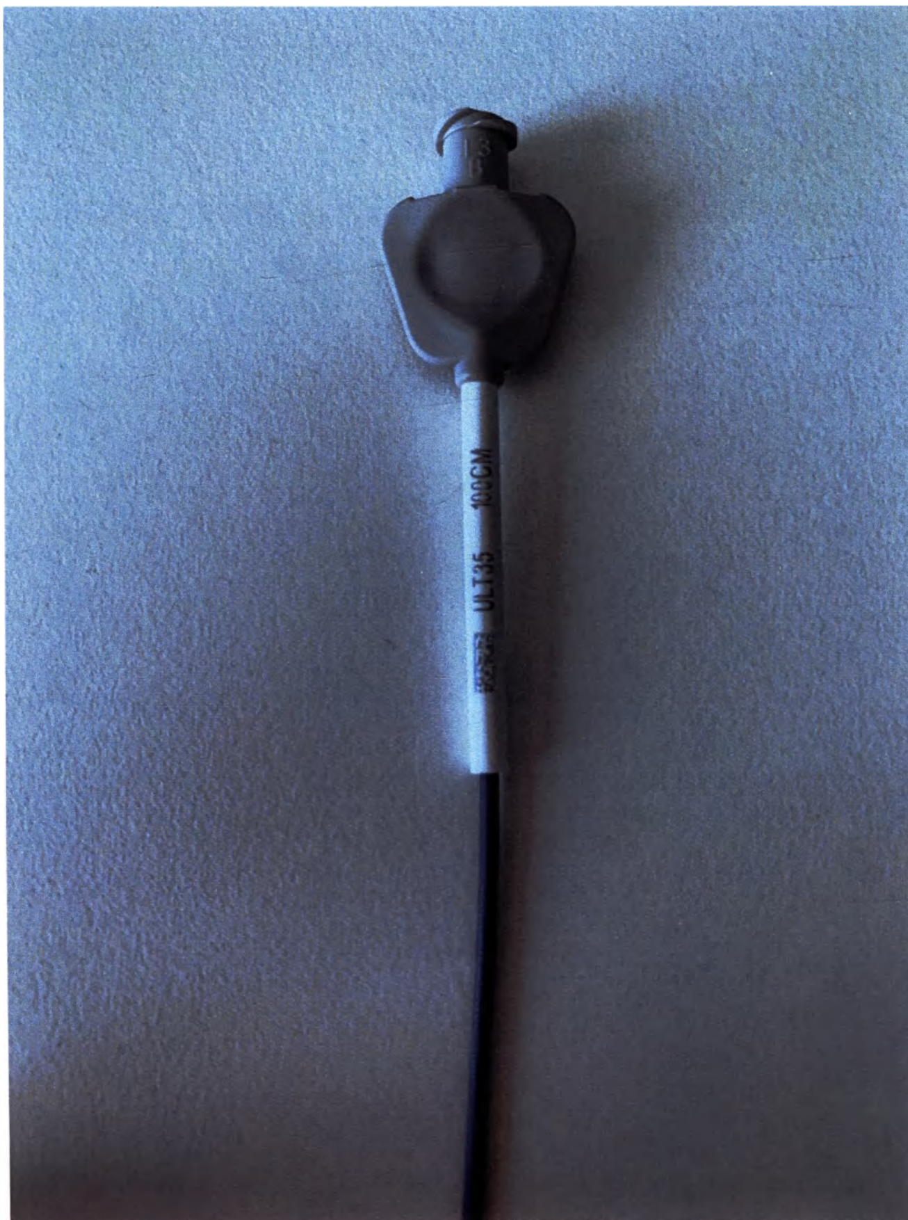
Рисунок 4. Катетер диагностический ангиографический DxTerity ULTRA (маркировка катетера)
