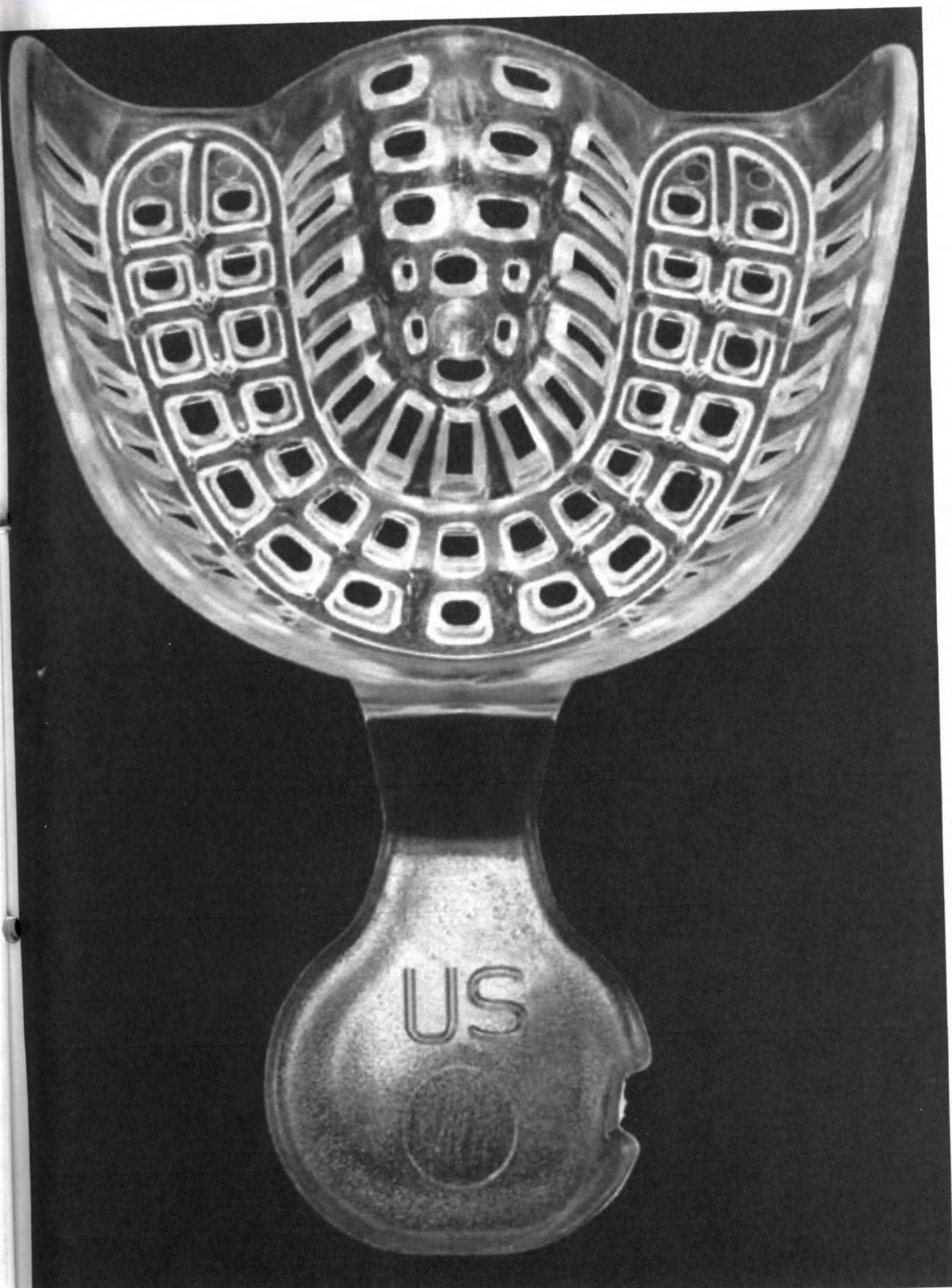
Рис. 11 – Ложка оттискная стоматологическая для снятия слепков полости рта Implant Tray в исполнении: US
