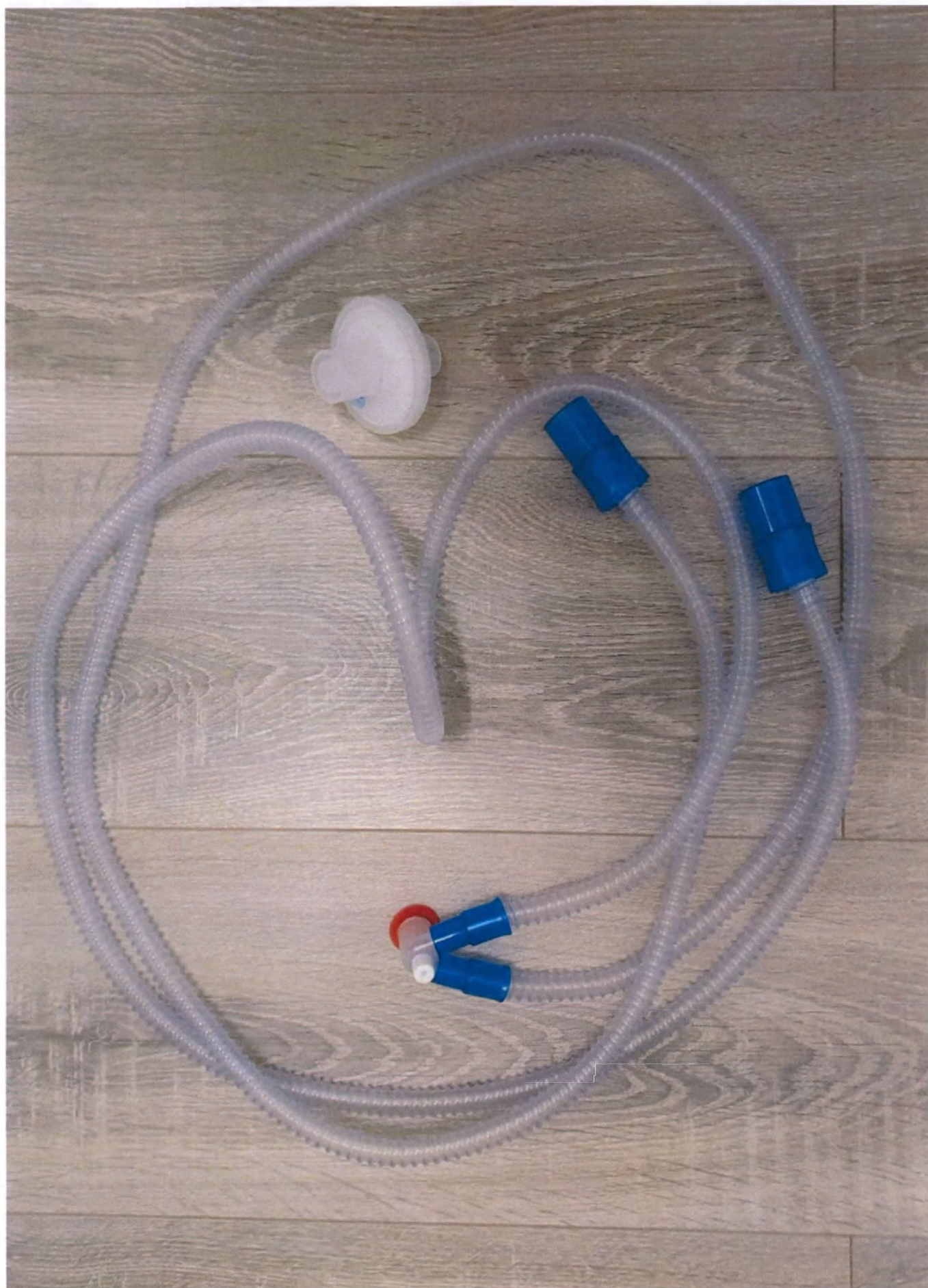
Неонатальный гладкоствольный (1 шт.), длина 150/175 см, с фильтром бактериально-вирусным (1 шт.).
