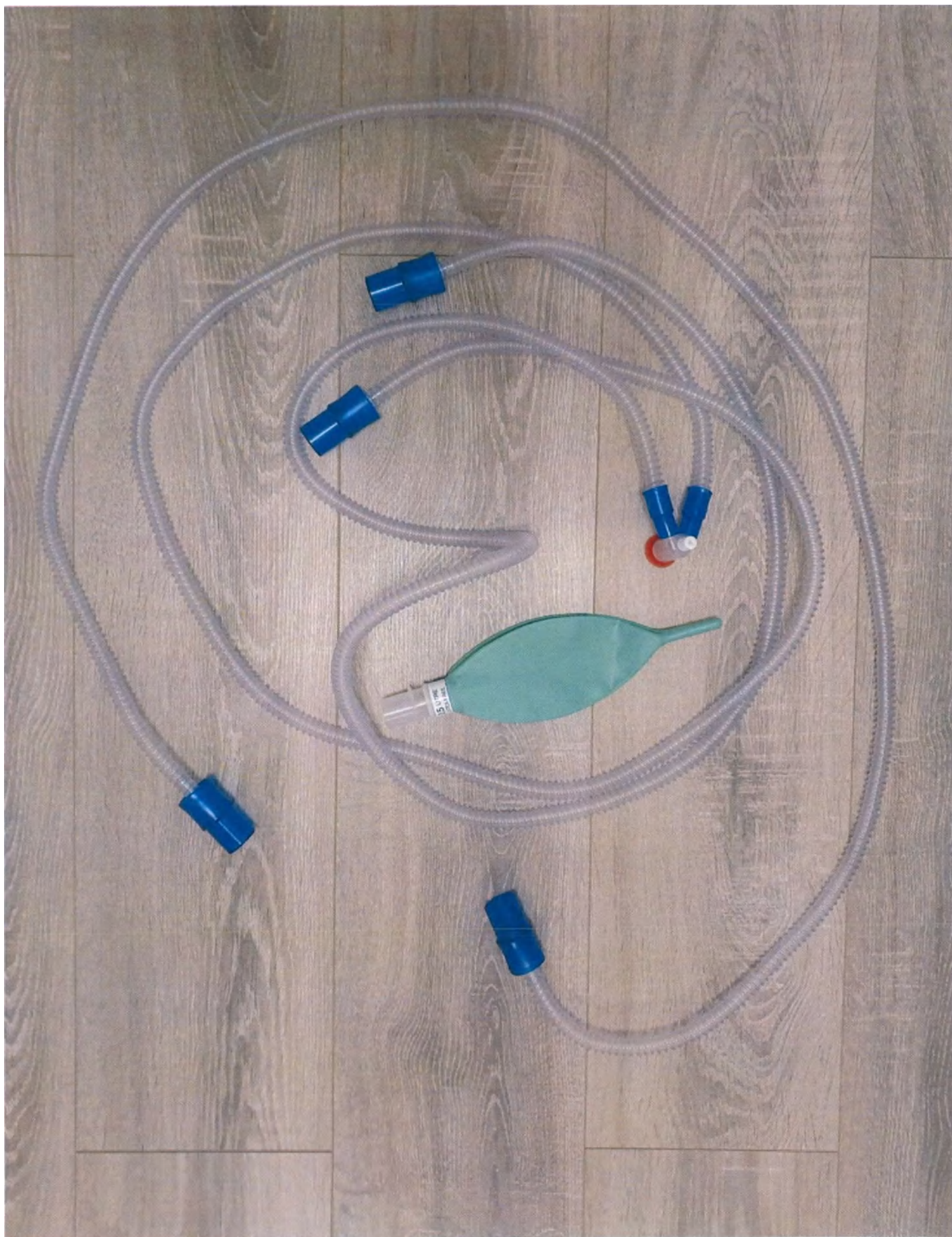
Неонатальный гладкоствольный (1 шт.), длина 150/175 см, с лимбом (1 шт.), с коннектором 22/22 мм (1 шт.), с мешком резервуарным 0.5л из неопрена (1 шт.).
