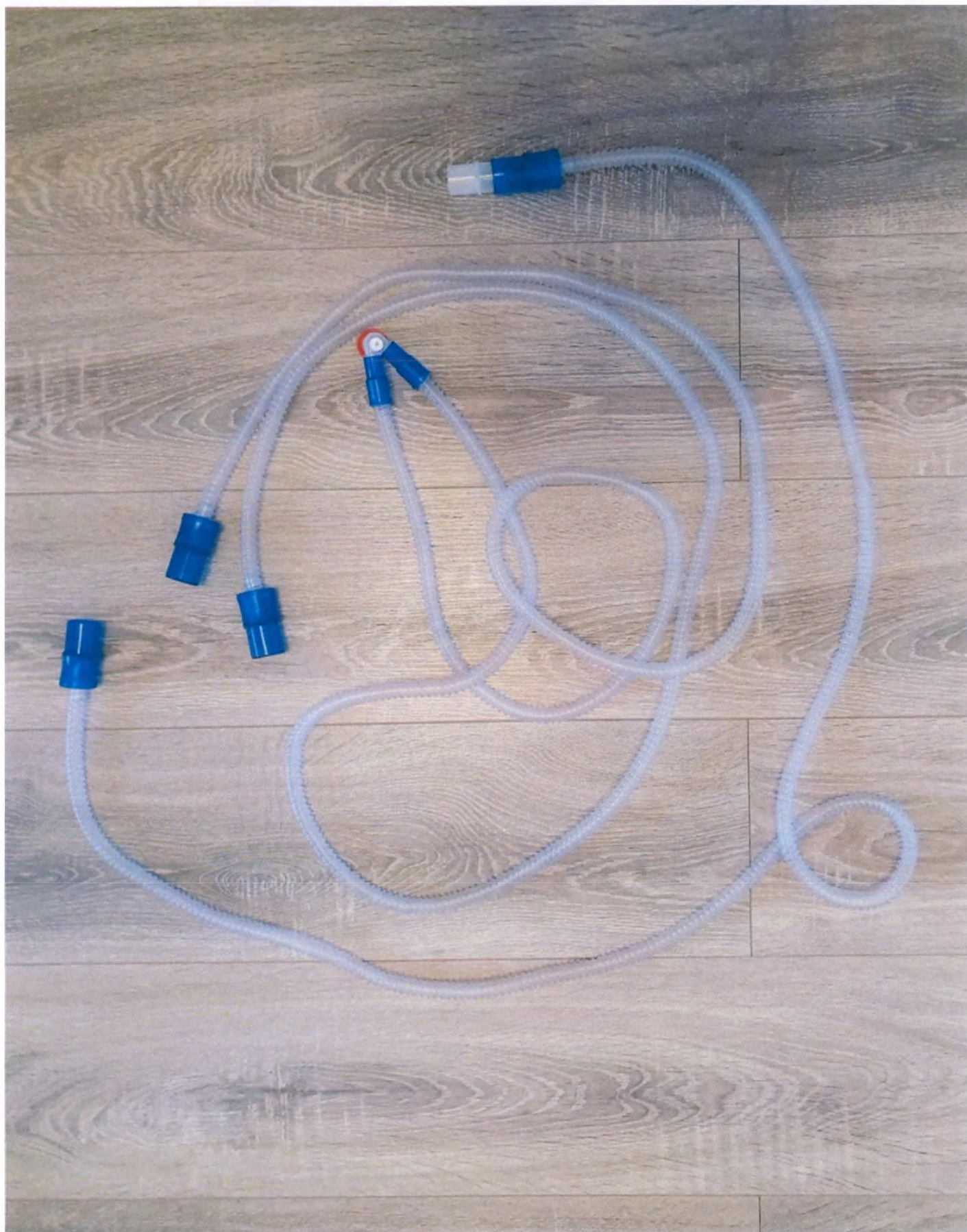
10. Неонатальный гладкоствольный (1 шт.), длина 150/175 см, с лимбом (1 шт.), с коннектором 22/22 мм (1 шт.).
