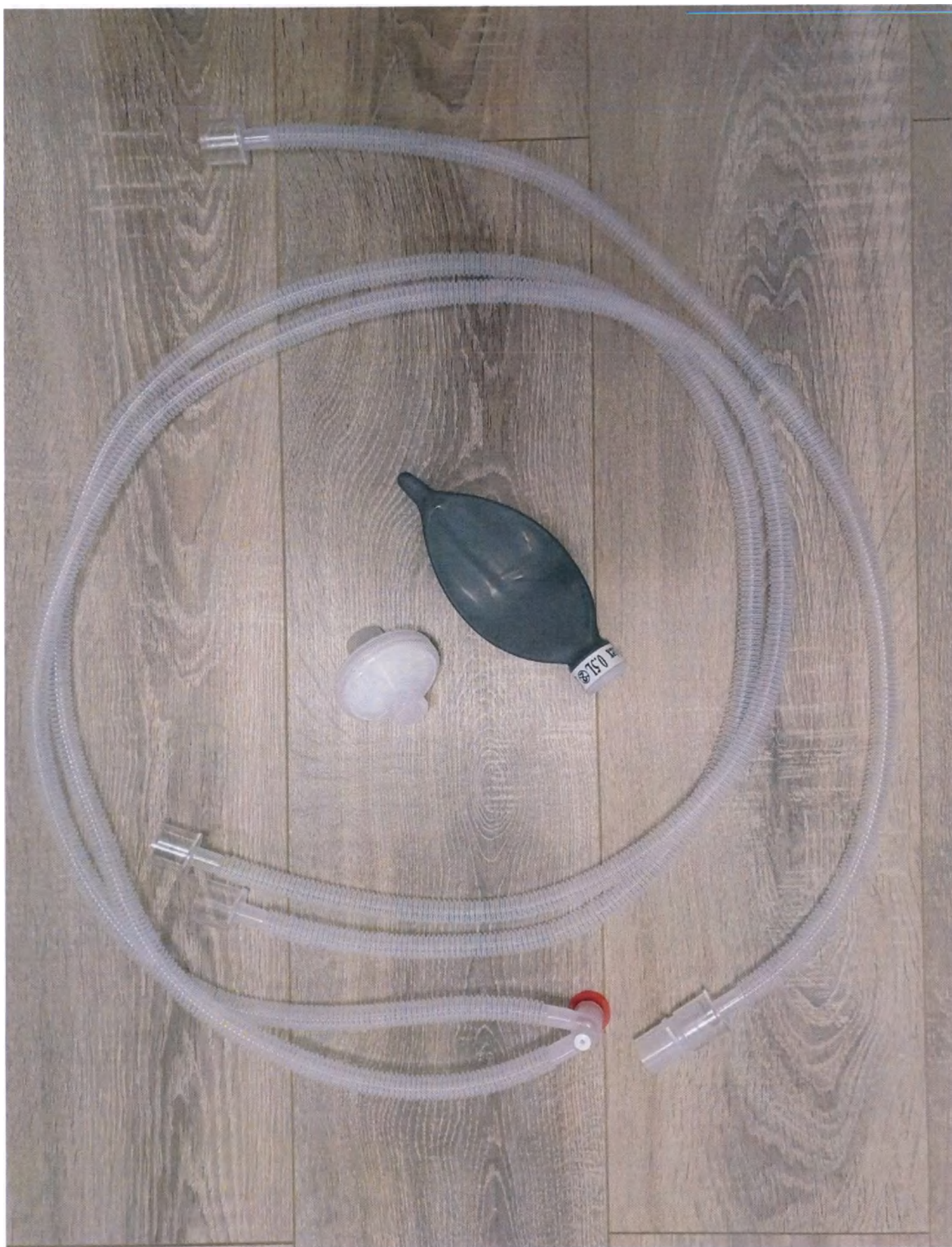
Неонатальный гофрированный (1 шт.), длина 160 см, с лимбом (1 шт.), с коннектором 22/22 мм (1 шт.), с мешком резервуарным 0.5л из латекса (1 шт.), с фильтром бактериально-вирусным (1 шт.).
