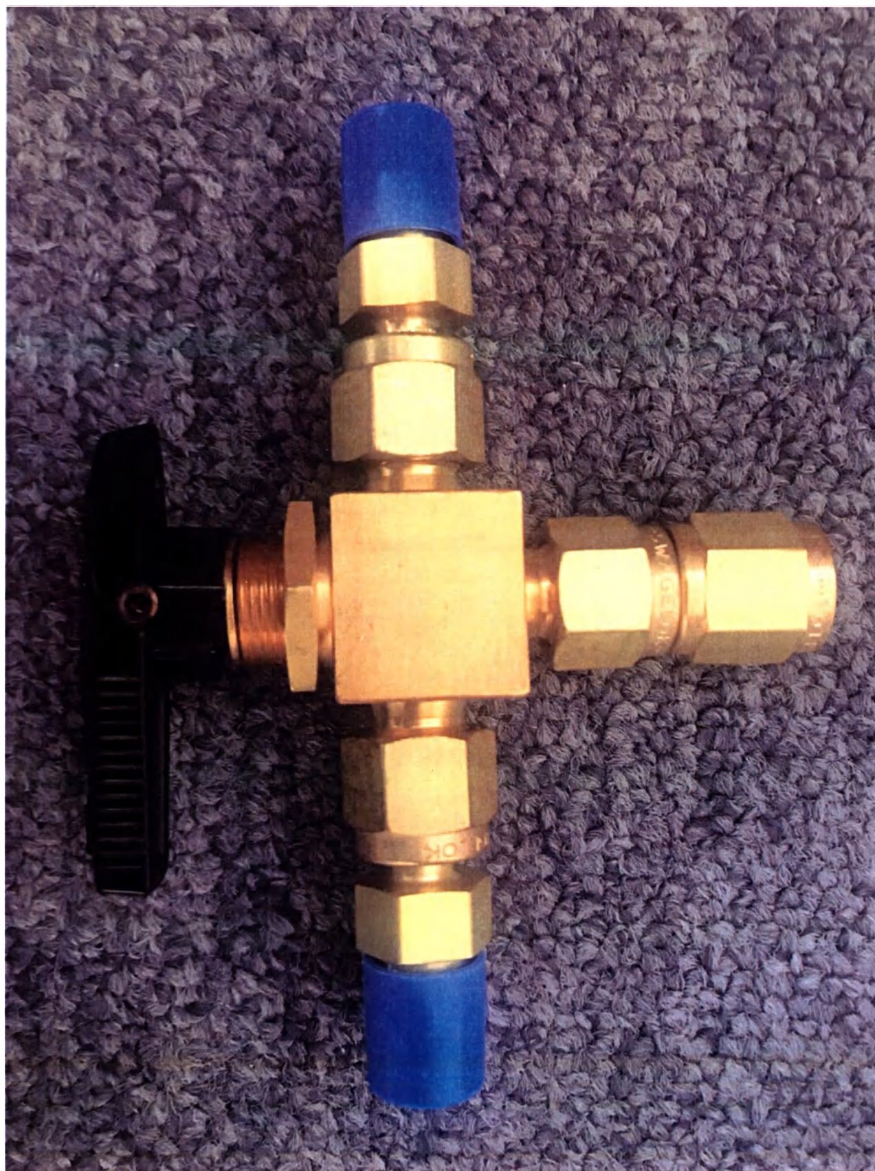
Общий вид изделия Переключающий клапан CO2 для инфляторов
