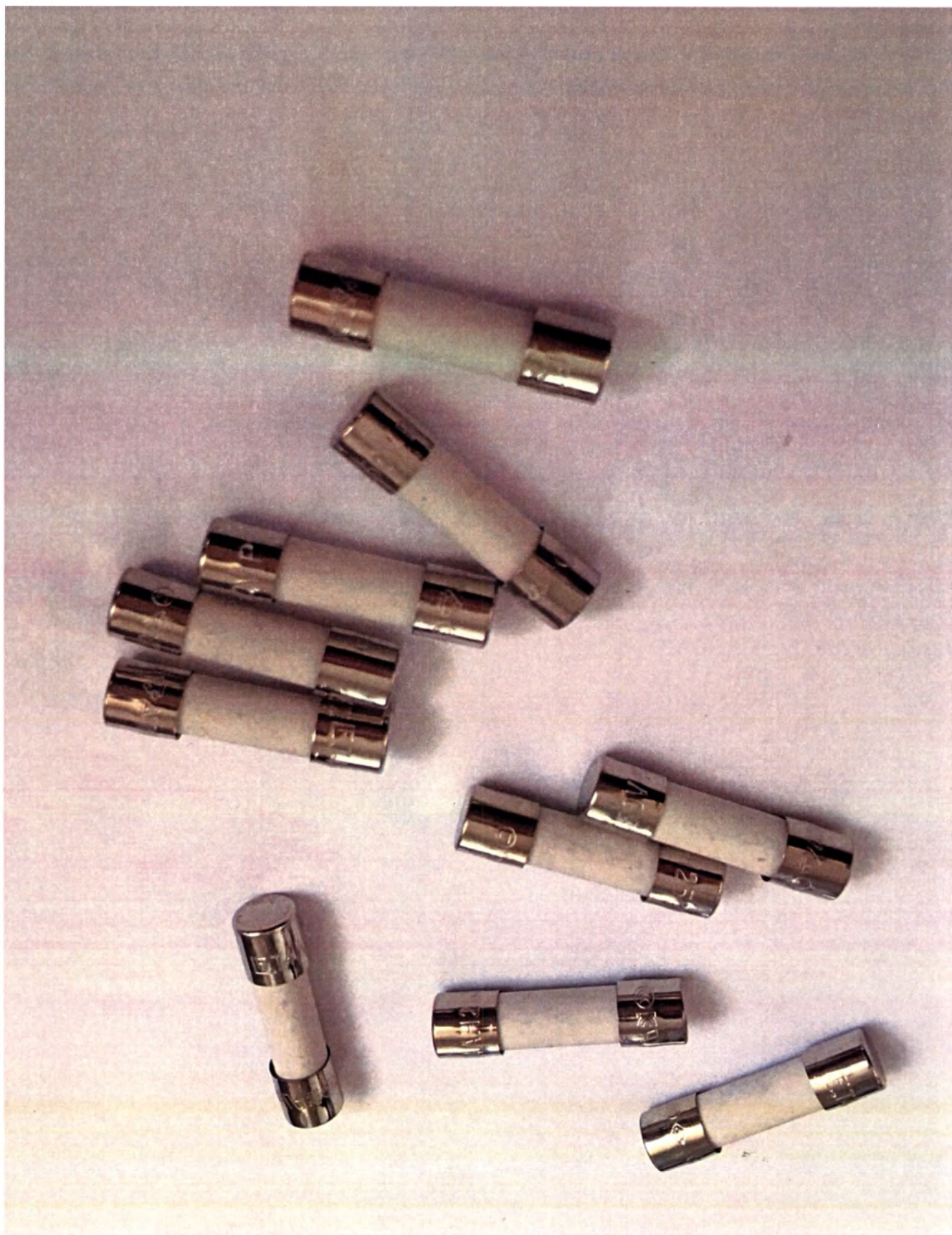
Общий вид изделия Микропредохранитель Т 4 А Н, 250 В перем. тока
