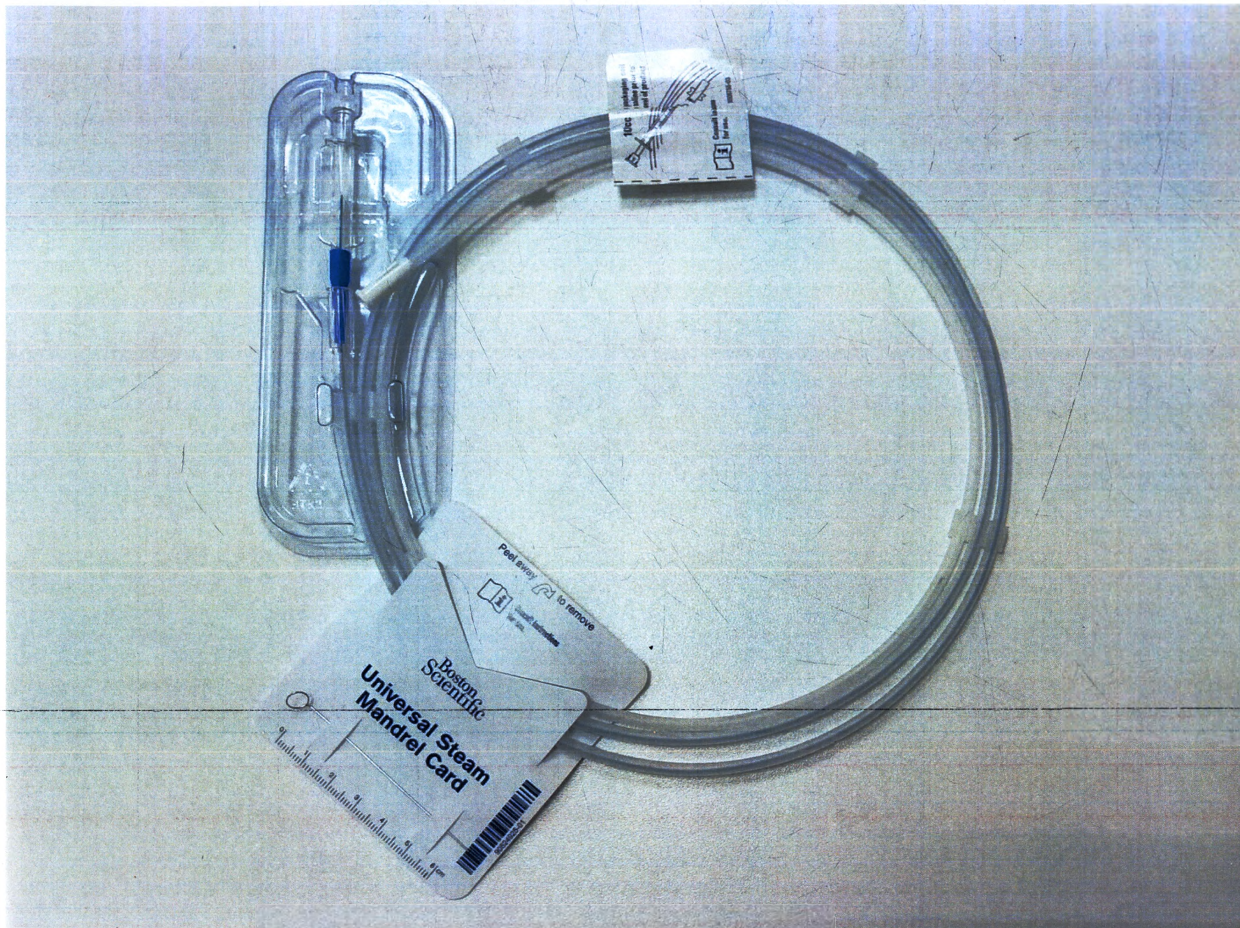
Общий вид микрокатетера с волоконной оплеткой RENEGADE прямой кончик
