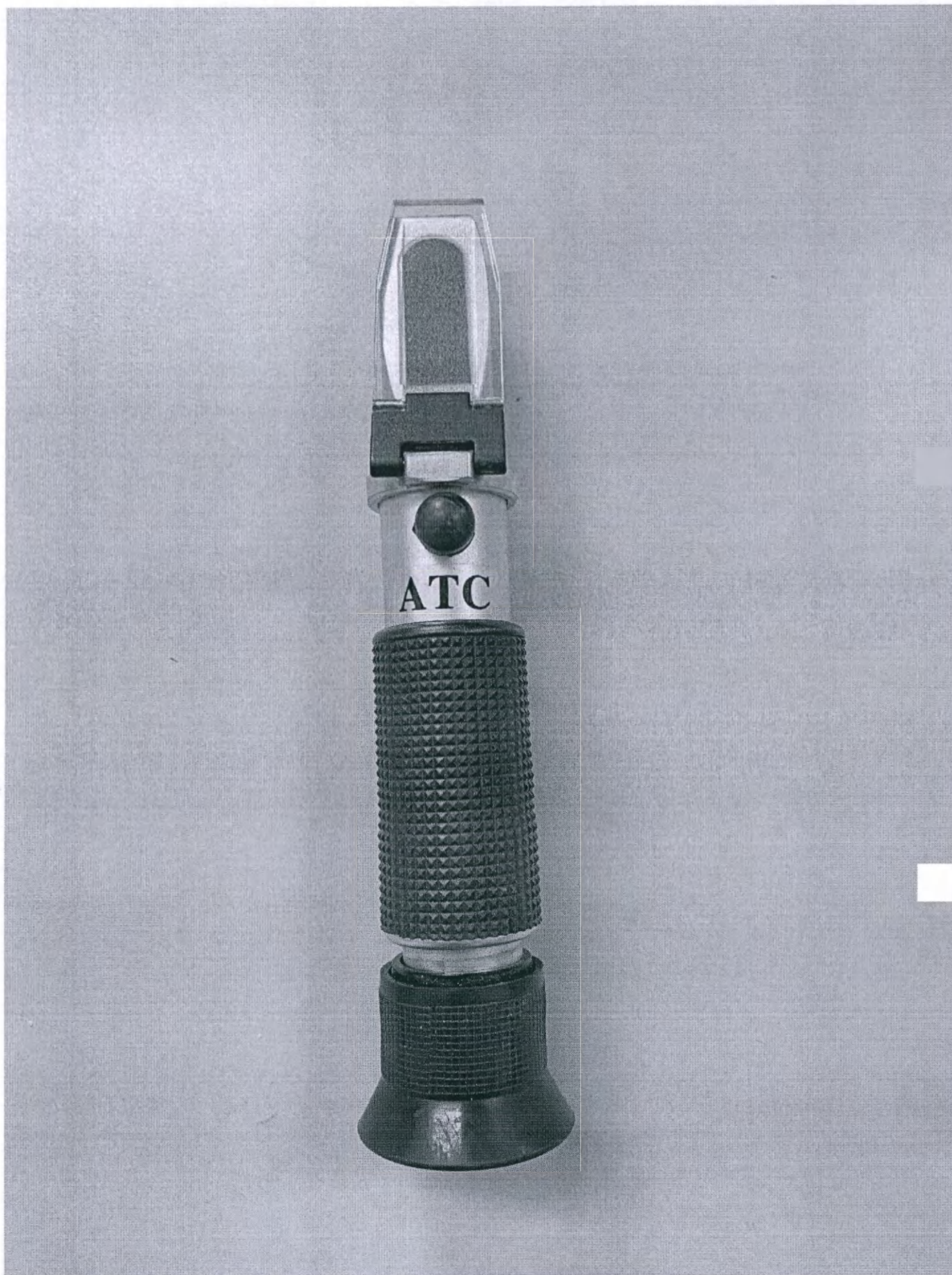
Рефрактометр для определения уровня смазочно-охлаждающей жидкости
