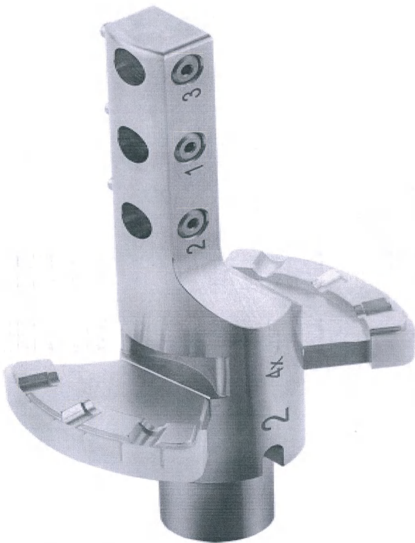
Держатель заготовок Стеклокерамика 3-х компонентный
