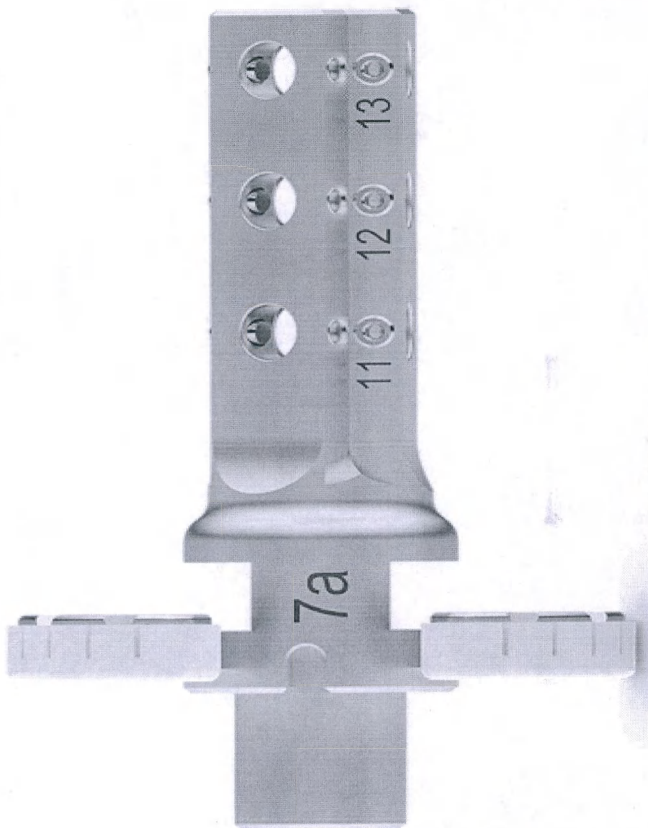
Держатель заготовок Стеклокерамика 9-ти компонентный
