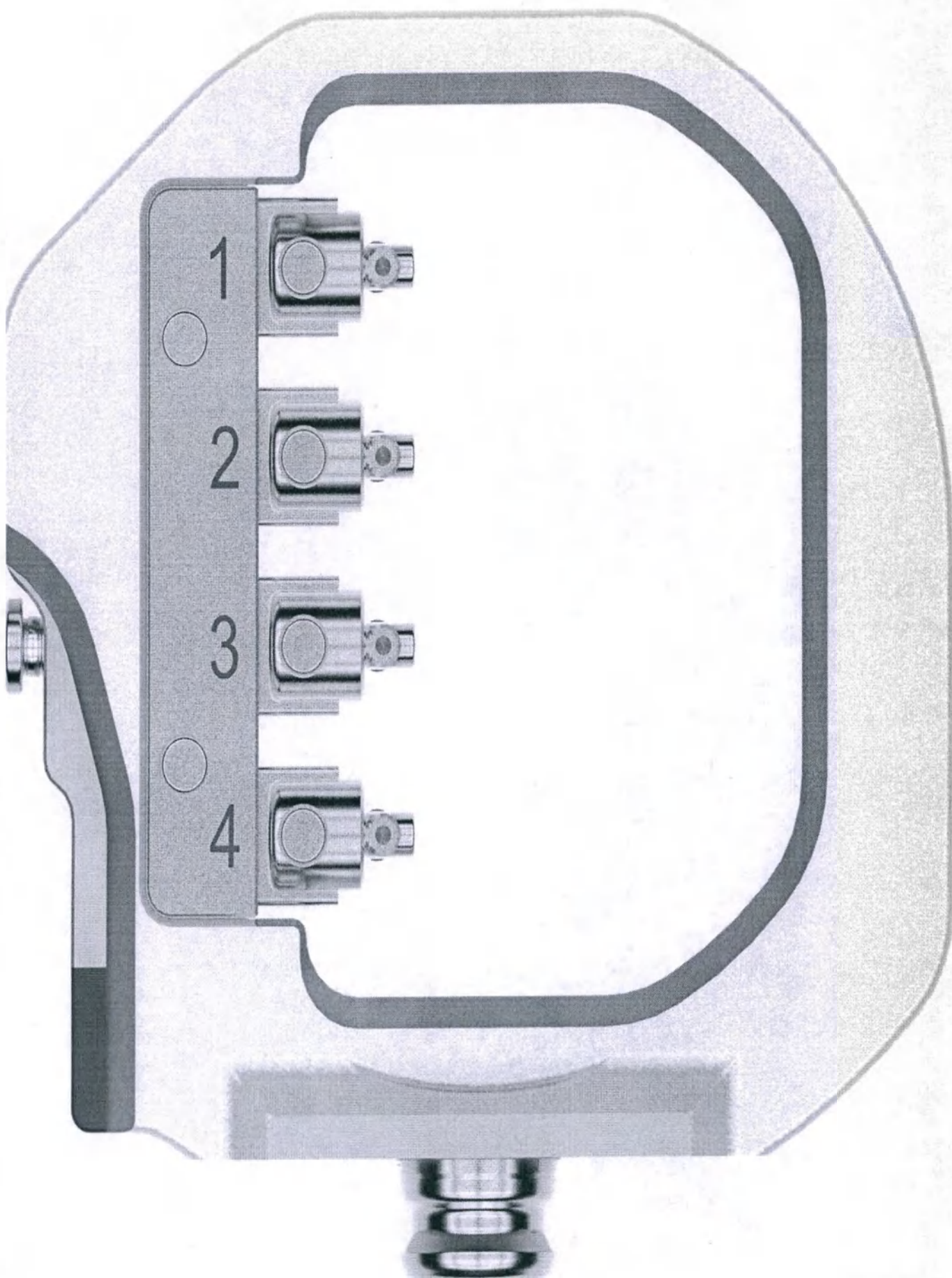
Держателей заготовок Ti-Preforms 181214
