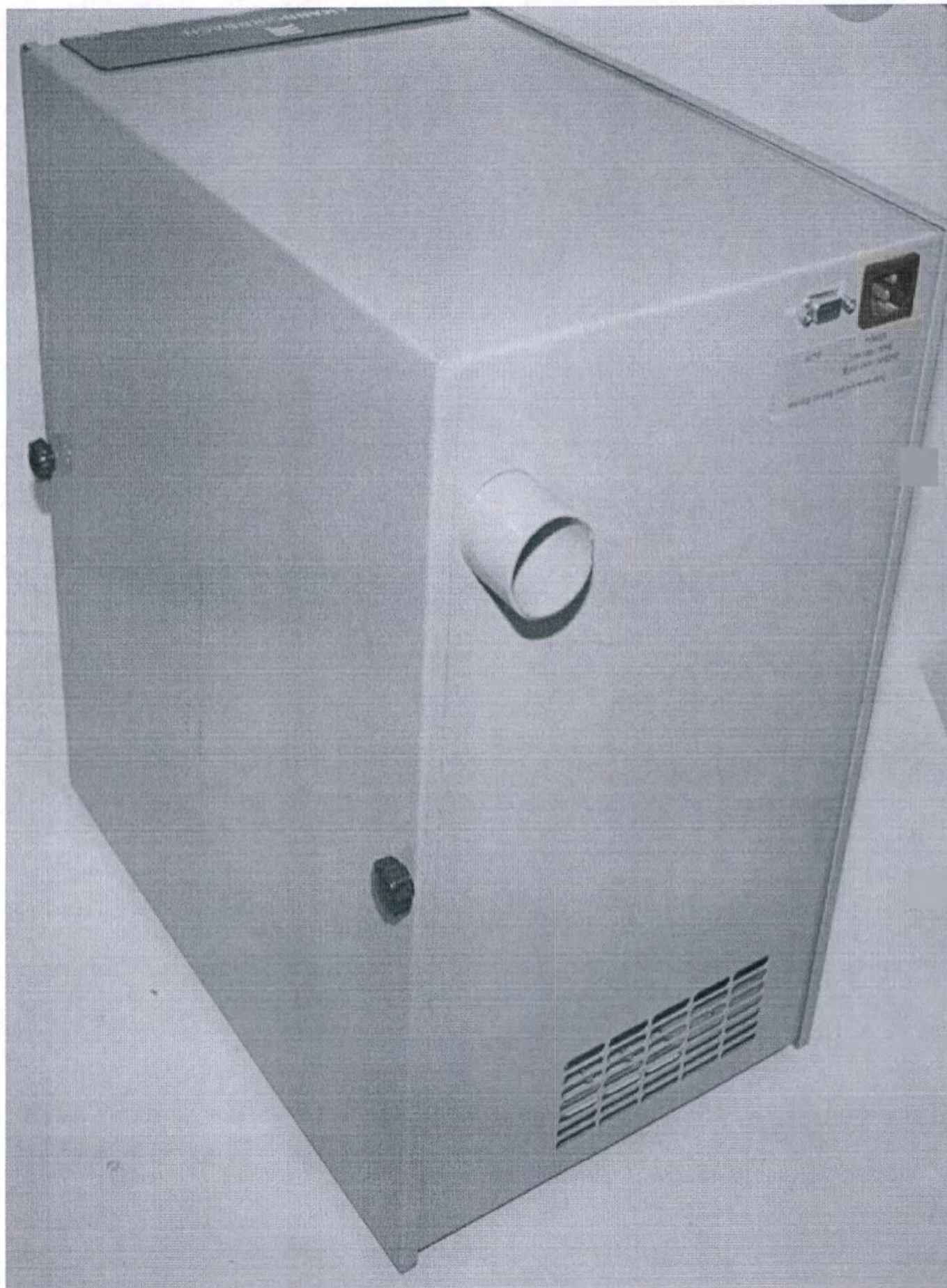
Вытяжка Ceramill Airstream. Вид сзади
