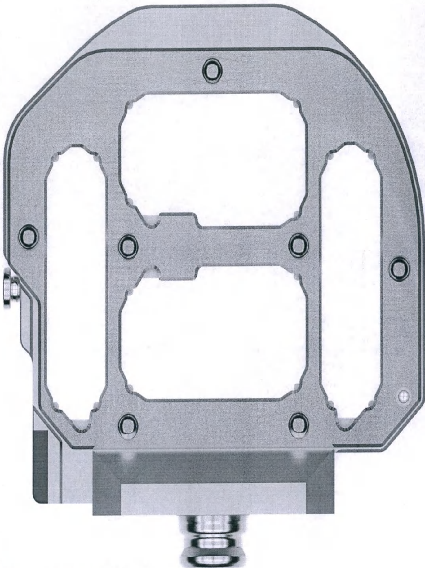
Держателей заготовок D-Set 181216
