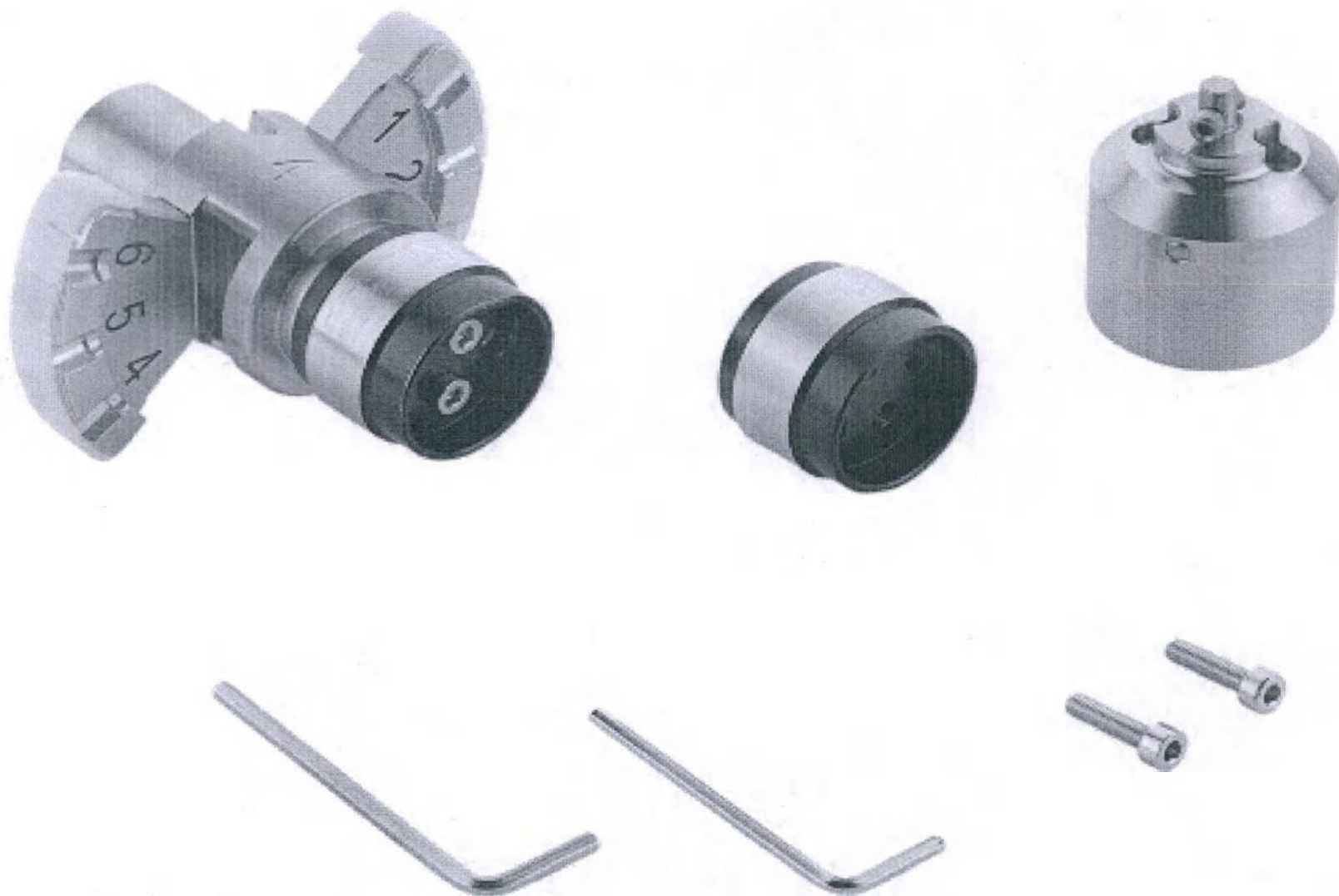
Держатель заготовок для ротационного фрезерования
