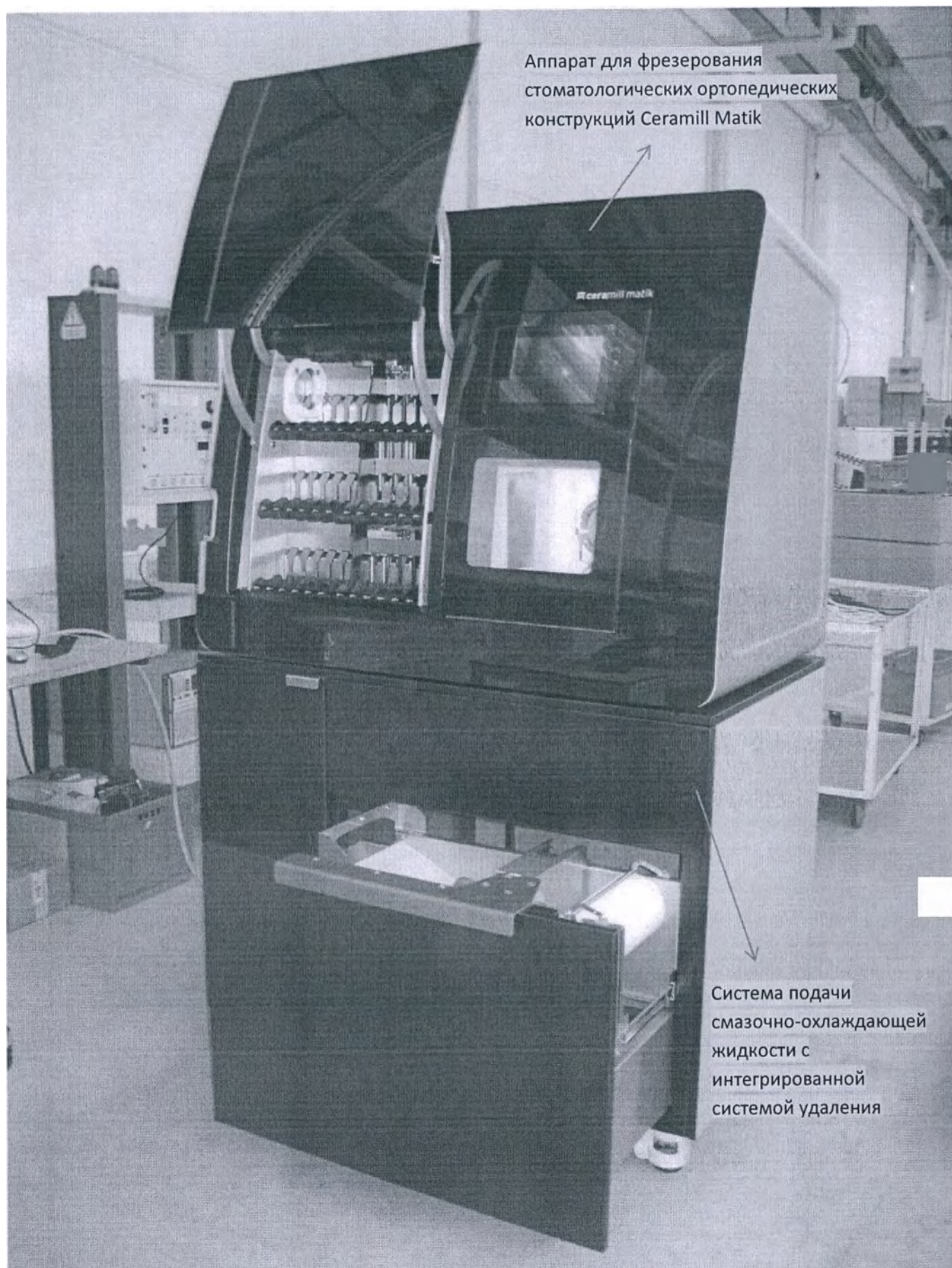
Аппарат для фрезерования стоматологических ортопедических конструкций Ceramill Matik и система подачи смазочно-охлаждающей жидкости с интегрированной системой удаления стружки Ceramill Cleanstream. Вид спереди
