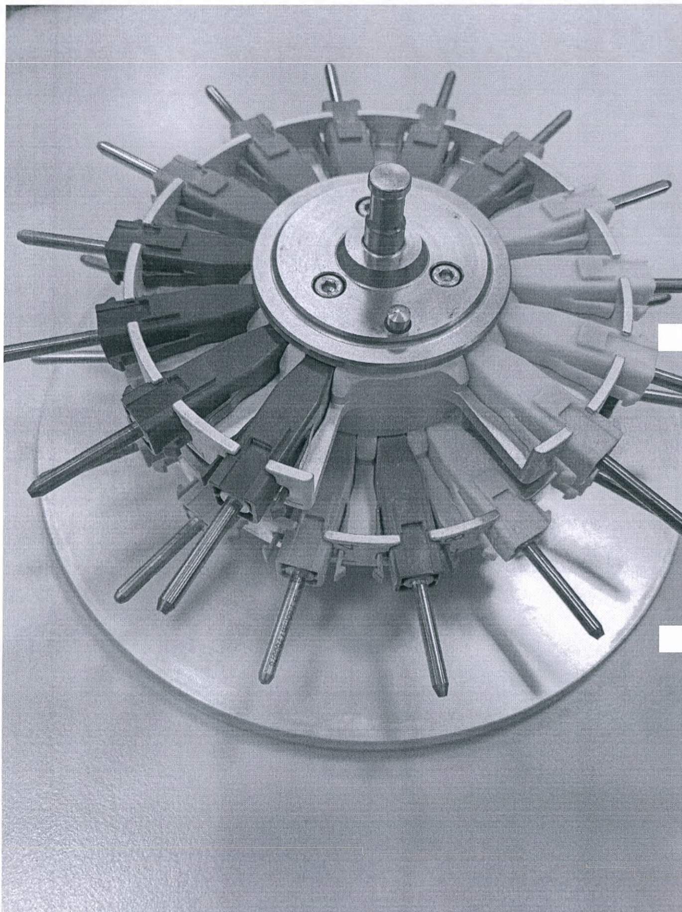
Барабан для фрезы
