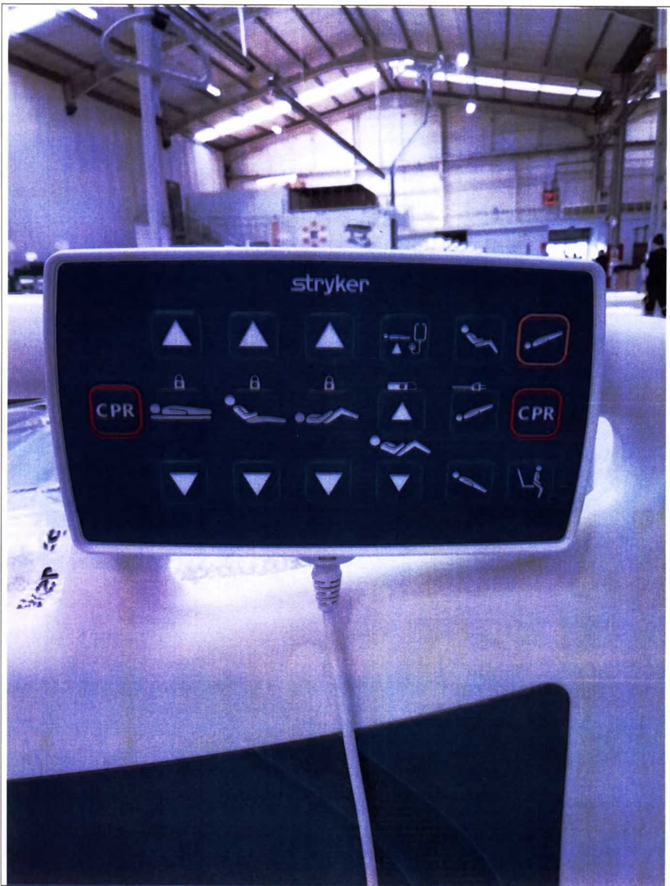
Подвесной пульт управления для медицинского персонала
