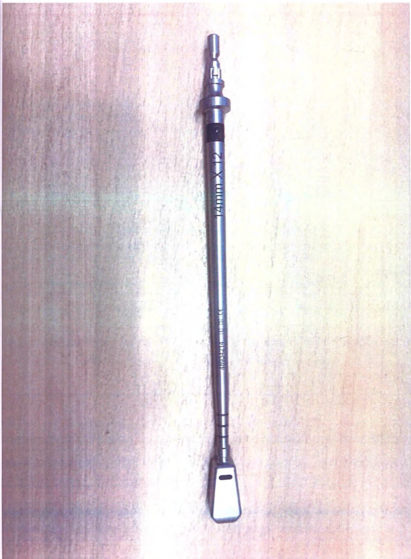
Общий вид изделия Пробный кейдж Tritanium TL
