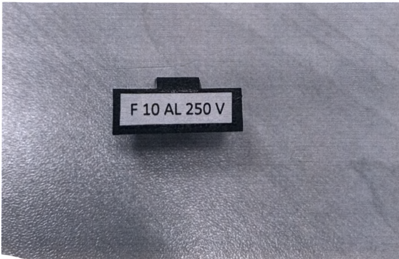
Рис. 1 - Фотоизображение общего вида маркировки держателя плавкого предохранителя
