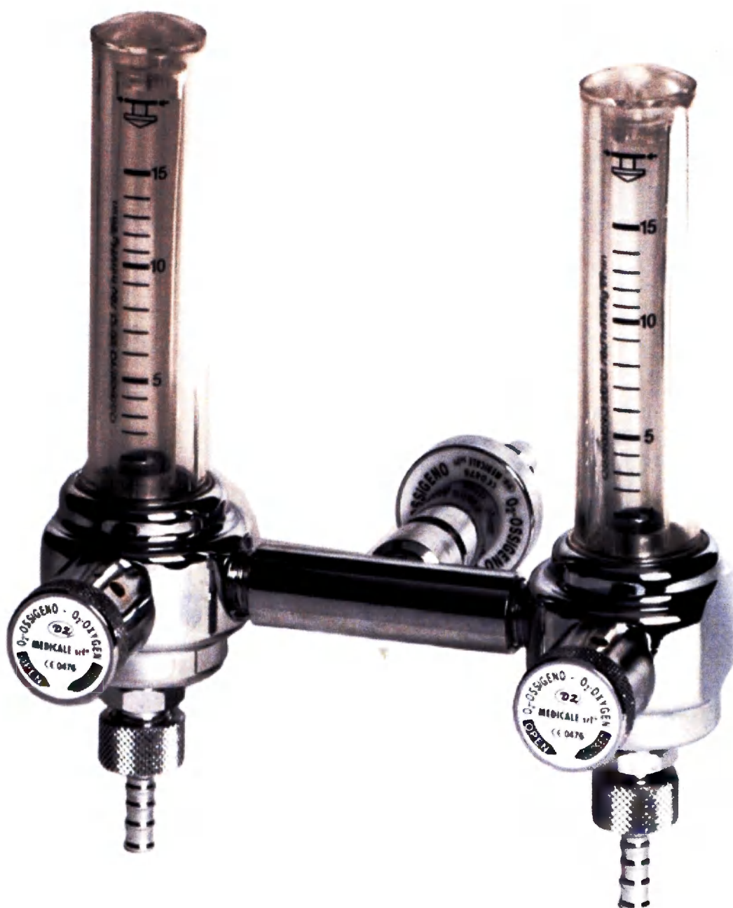
Расходомер двойной FLSM22DG
