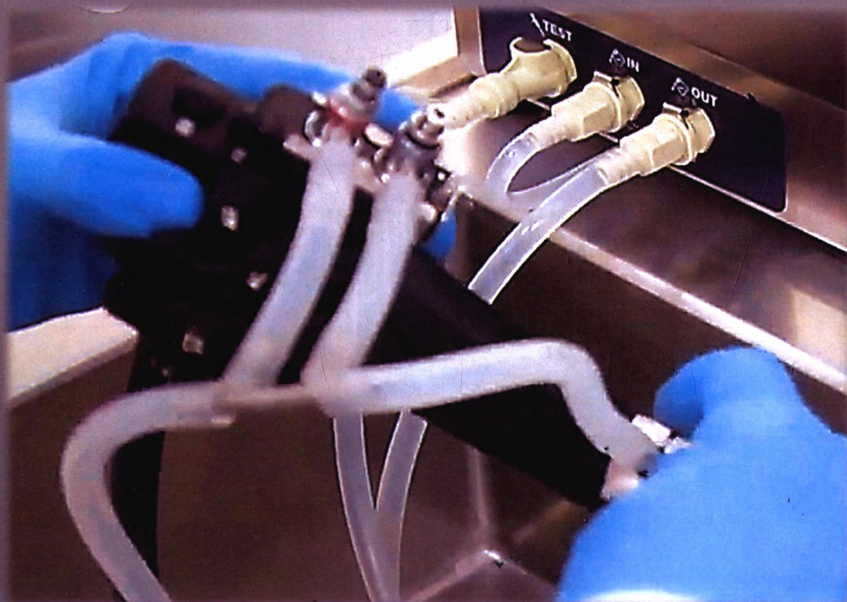
Фото 4а - Устройство предварительной очистки эндоскопов EPW 100, EPW 100 S: Коннекторы для эндоскопов
