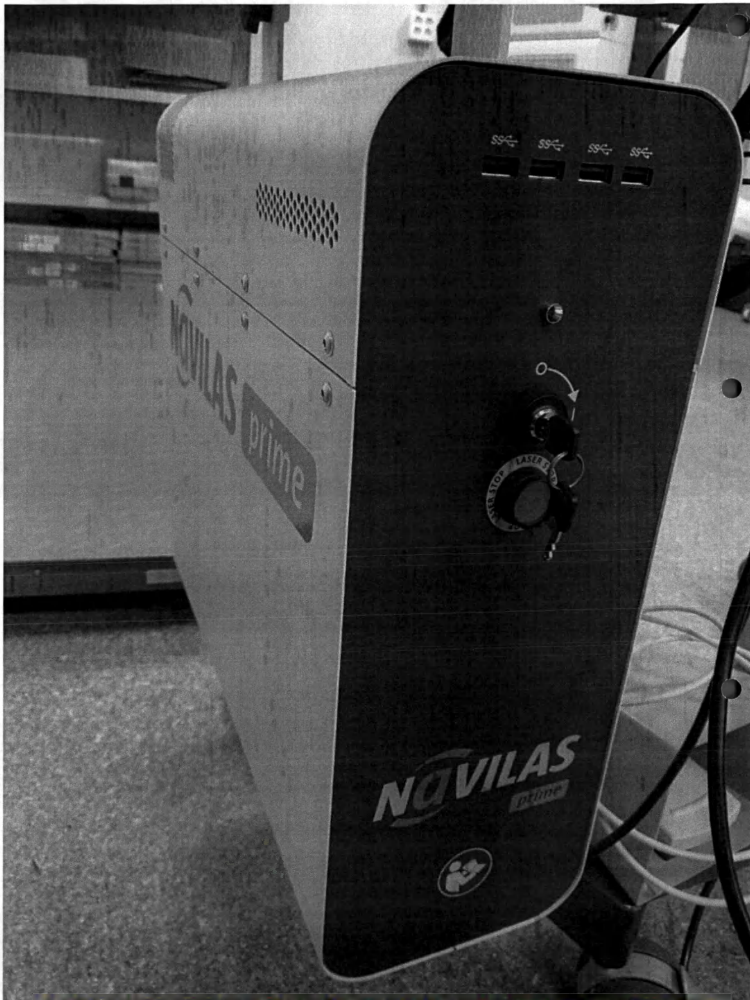
1. Электронный блок с лазерным модулем (комплект поставки №1: конфигурация «NAVILAS prime»)
