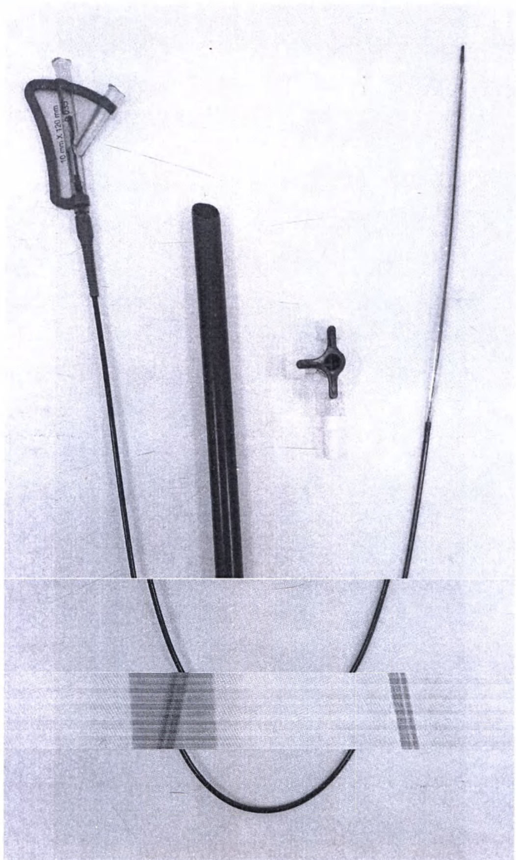
Рис. 9 Изображение Дилататора баллонного нефростомического диаметром 7 Fr (2,33 мм), длиной 55 см, с диаметром баллона 10 мм, длиной баллона 12 см.
