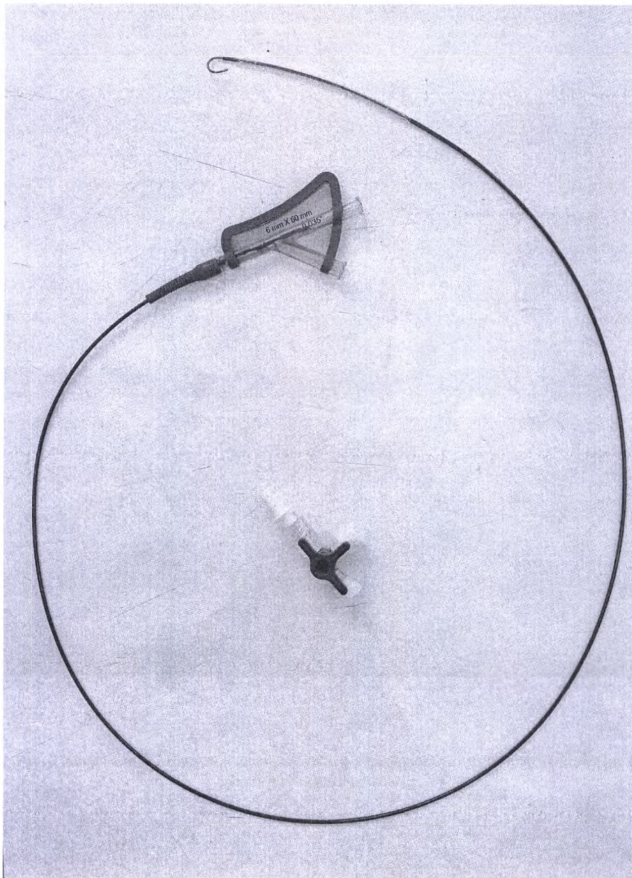
Рис. 6 Изображение Дилататора баллонного мочеточникового диаметром 4,8 Fr (1,60 мм) длиной 75 см с диаметром баллона 6 мм, длиной баллона 60 мм.
