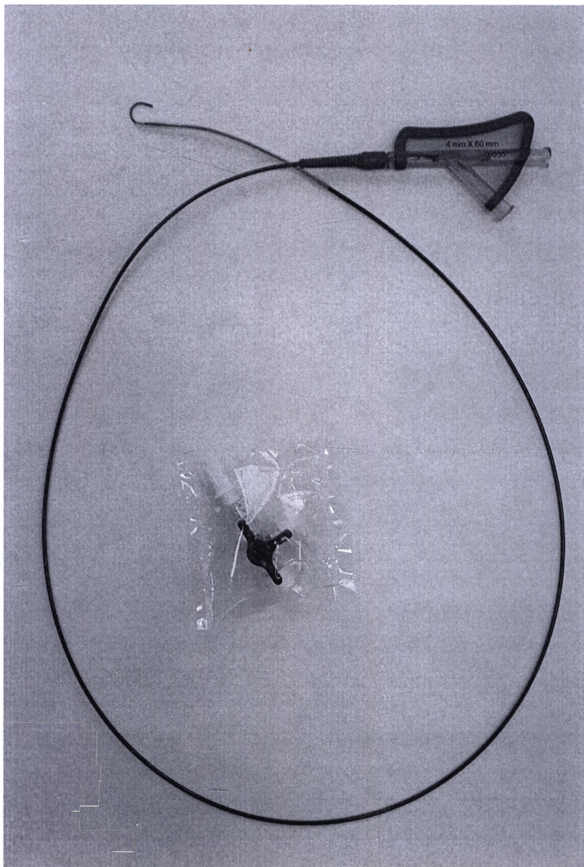
Рис. 2 Изображение Дилататора баллонного мочеточникового диаметром 4,8 Fr (1,60 мм) длиной 75 см с диаметром баллона 4 мм, длиной баллона 60 мм.
