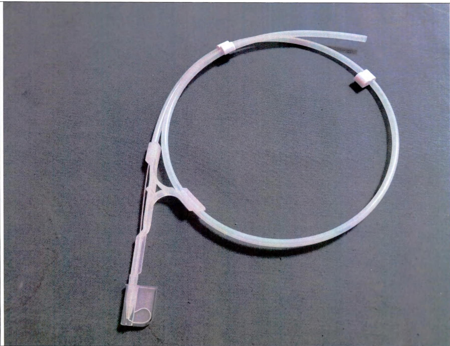
Рис. 22. Направитель проволоочный 0,032 дюйма (0,81 мм.) x 60 см.
