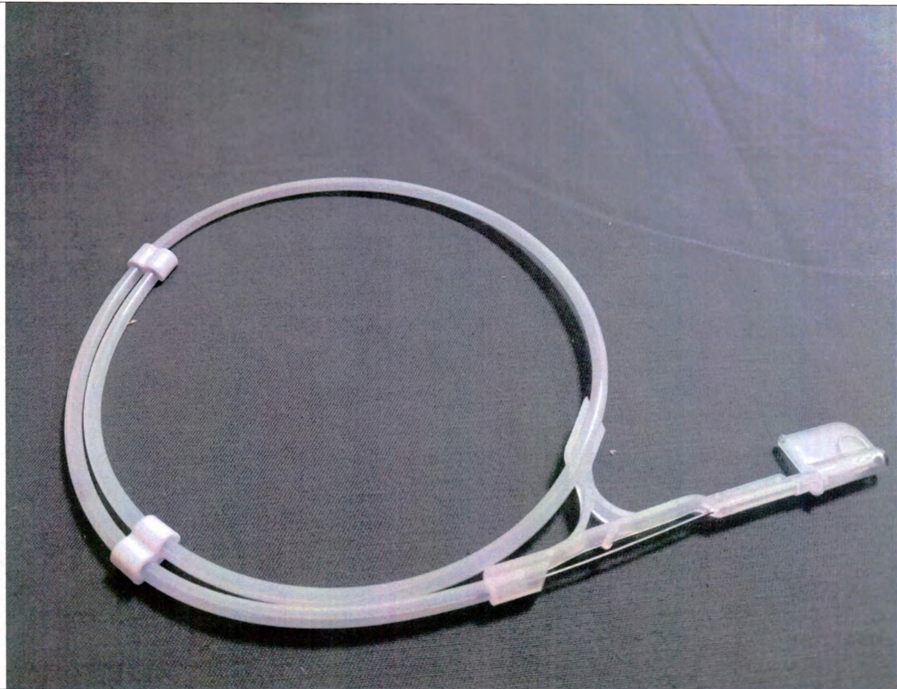
Рис. 43. Направитель проволоочный 0,032 дюйма (0,81 мм.) x 60 см.
