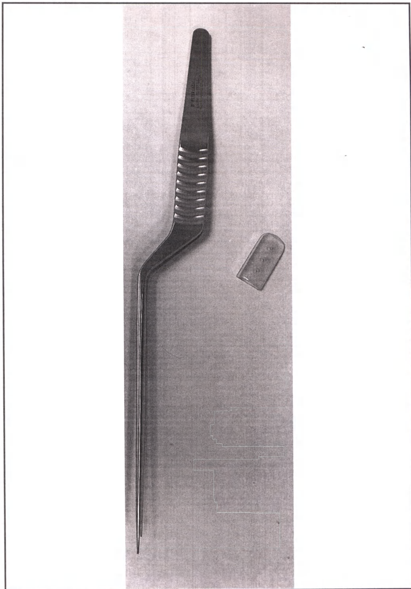
Микро-зажим L-Line Classic, бранши прямые, 0,9 мм, длина 245 мм, REF 70.157.03 – общий вид изделия
