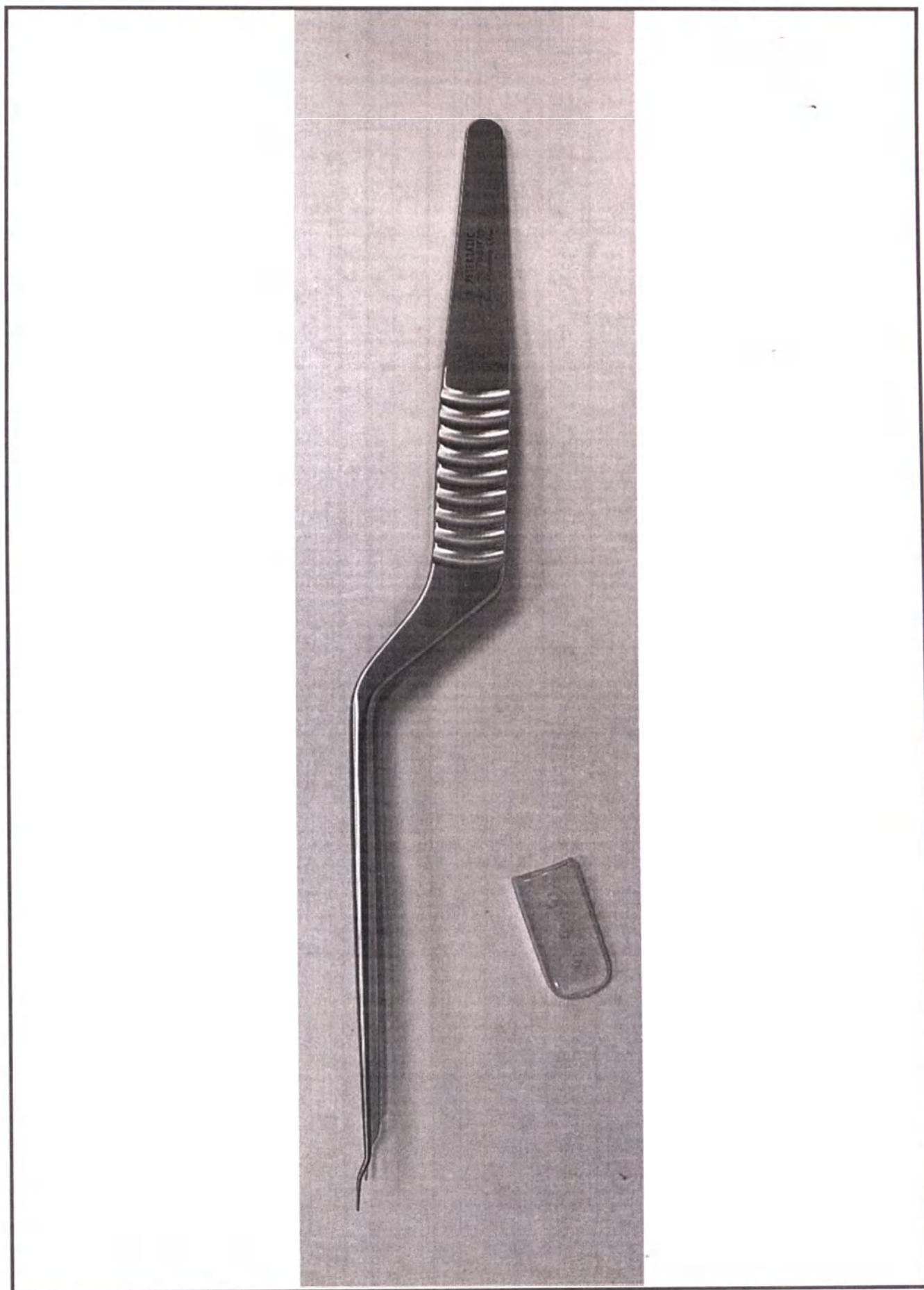
Микро-зажим L-Line Classic, бранши зубчатые, длина 180 мм, REF 70.837.03 – общий вид изделия
