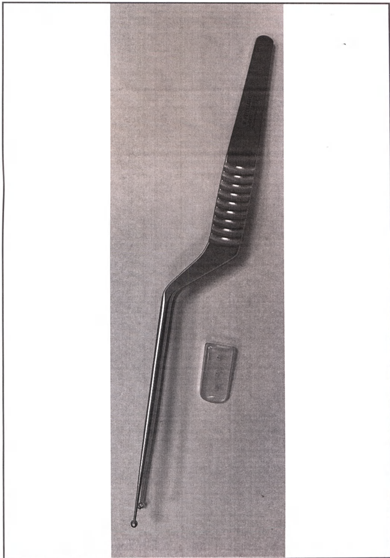
Микро-зажим L-Line Classic, Yasargil-Samii, бранши ложкаобразные Ø 3 мм, длина 220 мм, REF 72.210.03 – общий вид изделия
