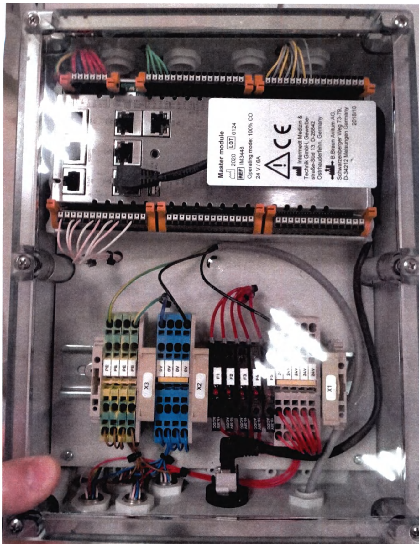
Мастер-модуль
