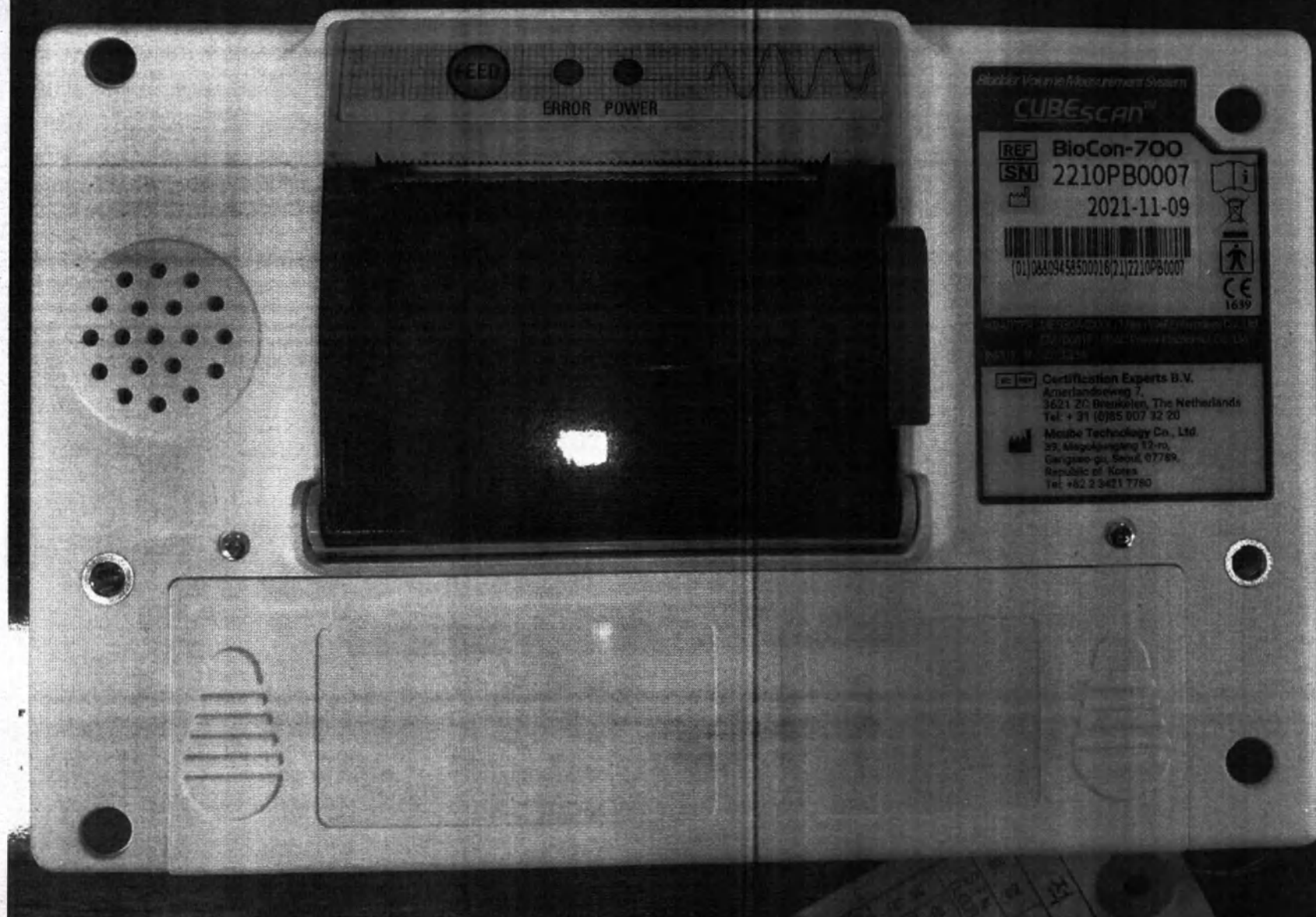
Консоль с встроенным термопринтером вид сзади
