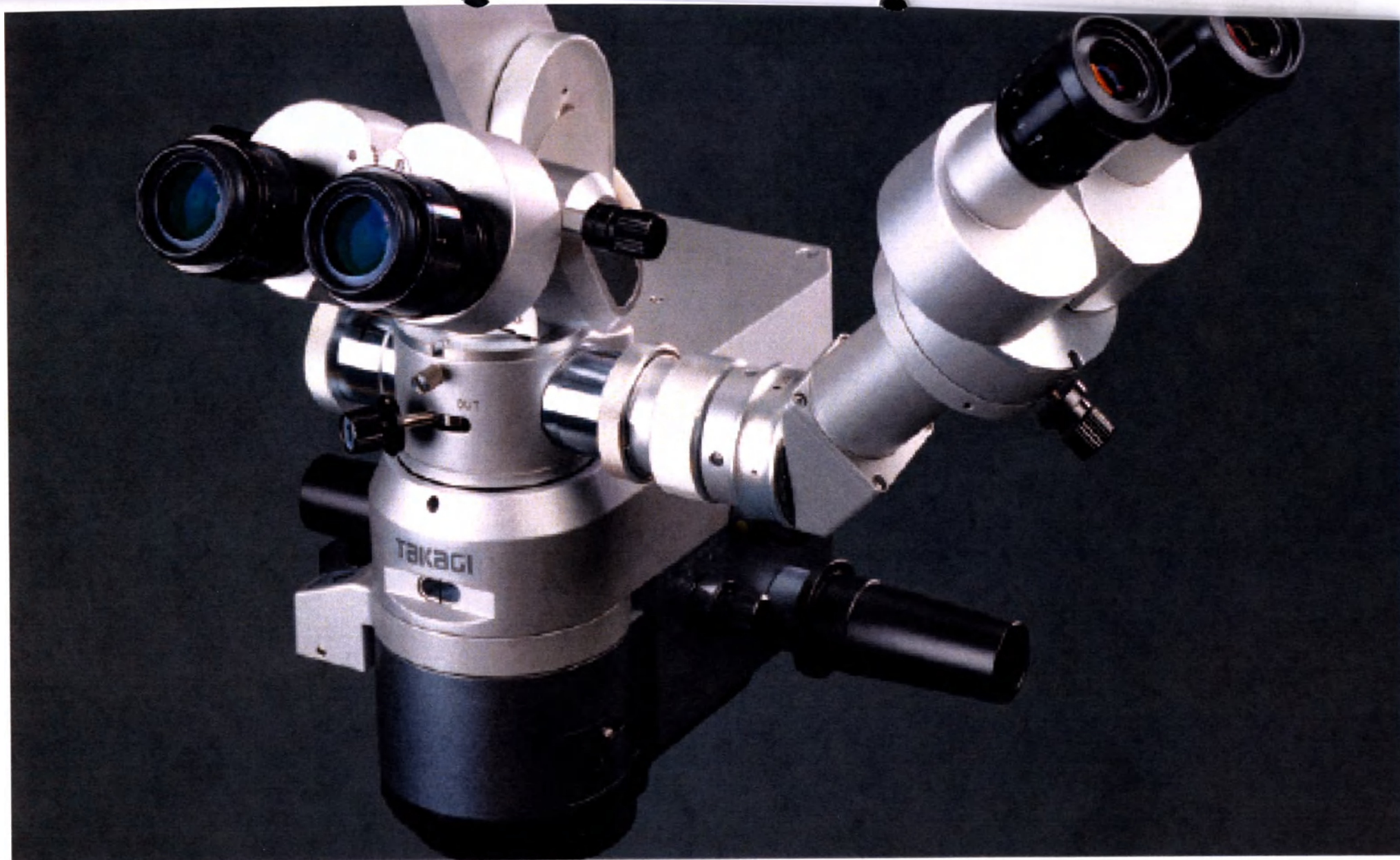
Биноклярный микроскоп ассистента с монтажным кольцом.
