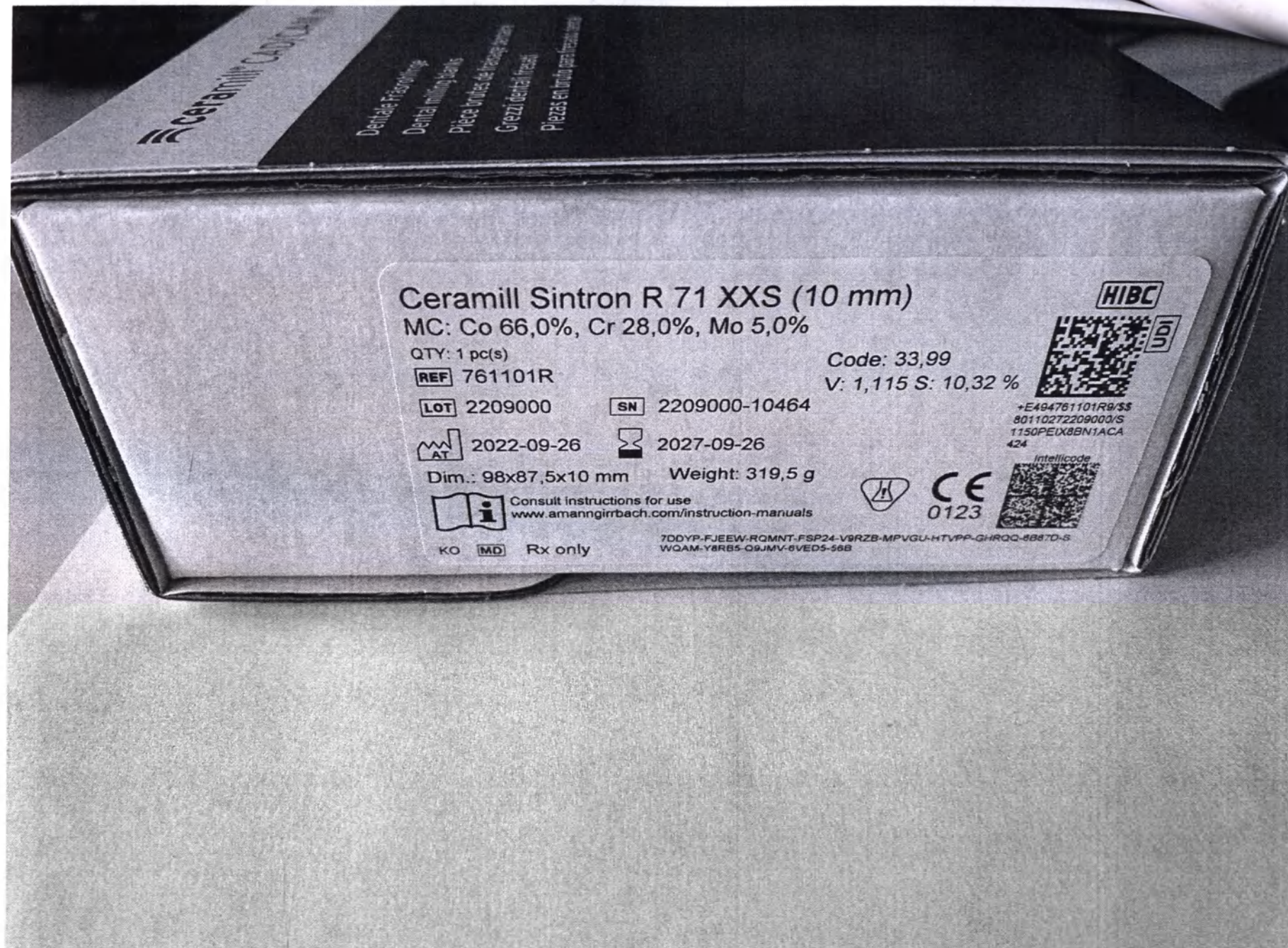
Заготовки из кобальтхромового сплава для ортопедической стоматологии Ceramill Sintron. Маркировка на упаковке (например, Заготовки из кобальтхромового сплава для ортопедической стоматологии Ceramill Sintron R 71XXS)
