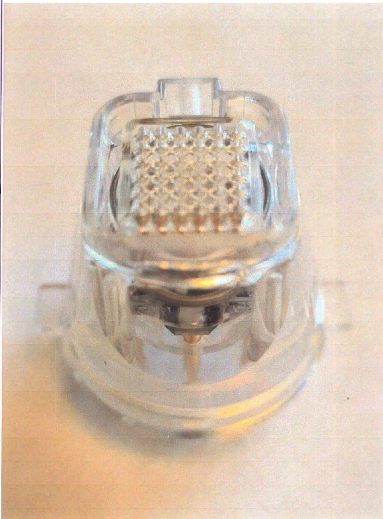
Фотографическое изображение 13. Аппарат косметологический для лифтинга Focus Dual. Наконечник стерильный одноразовый мультиигольчатый FDRK-36PN изолированный.
