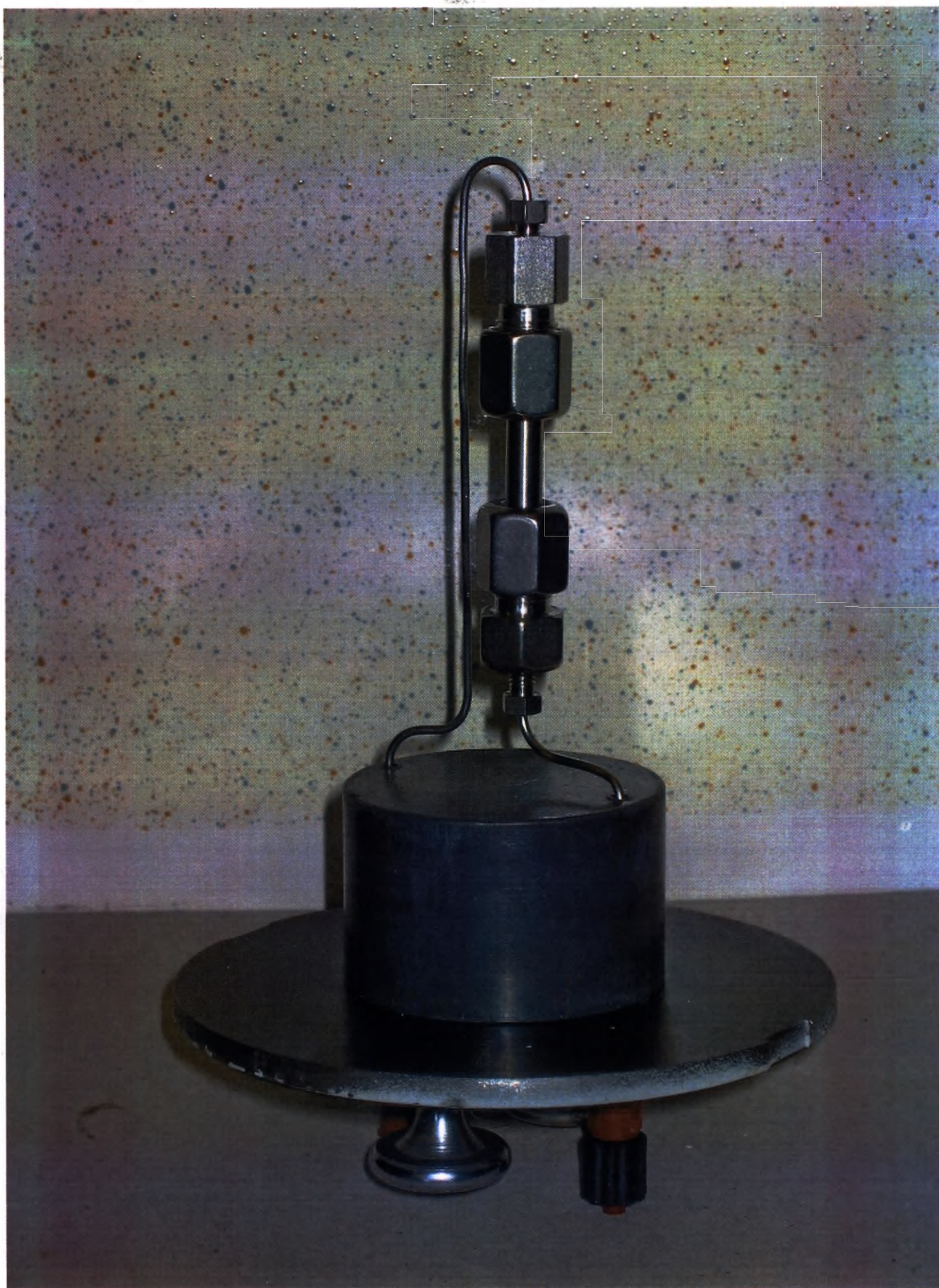
Колонка генераторная подключенная к заглушкам типа Луер Лок (Luer Lock)
