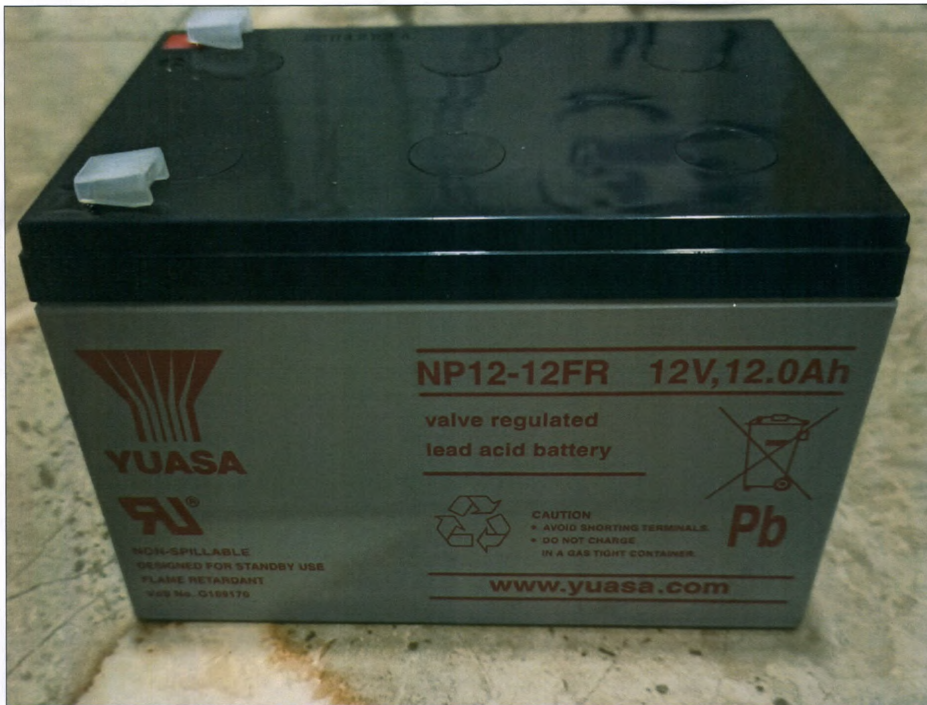
Фото 24. Аккумуляторная батарея аварийного режима работы светильника – не более 6 шт. (при необходимости)
