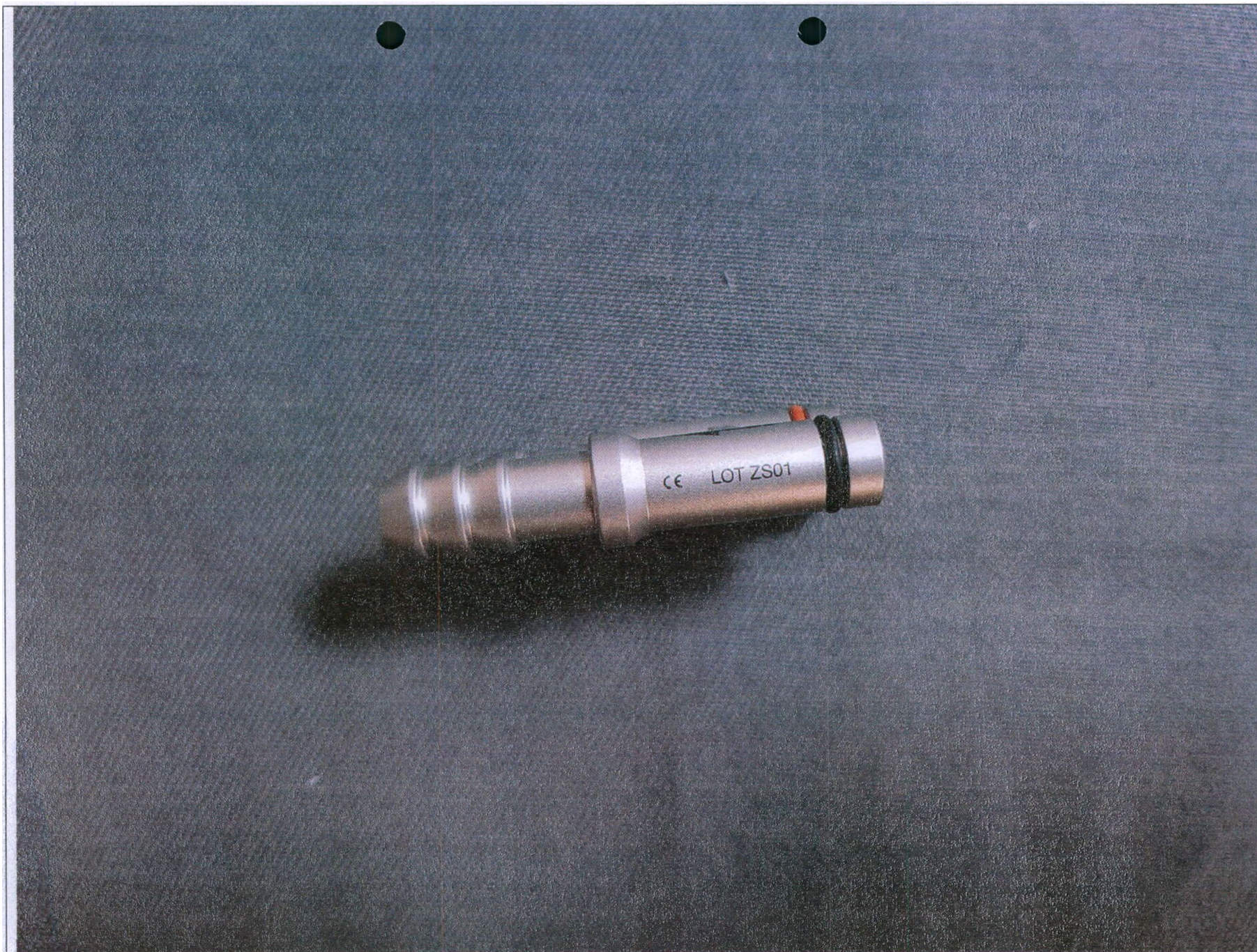
Рис. 72. Адаптер-моноблок для гистероскопа В.І.О.Н.
