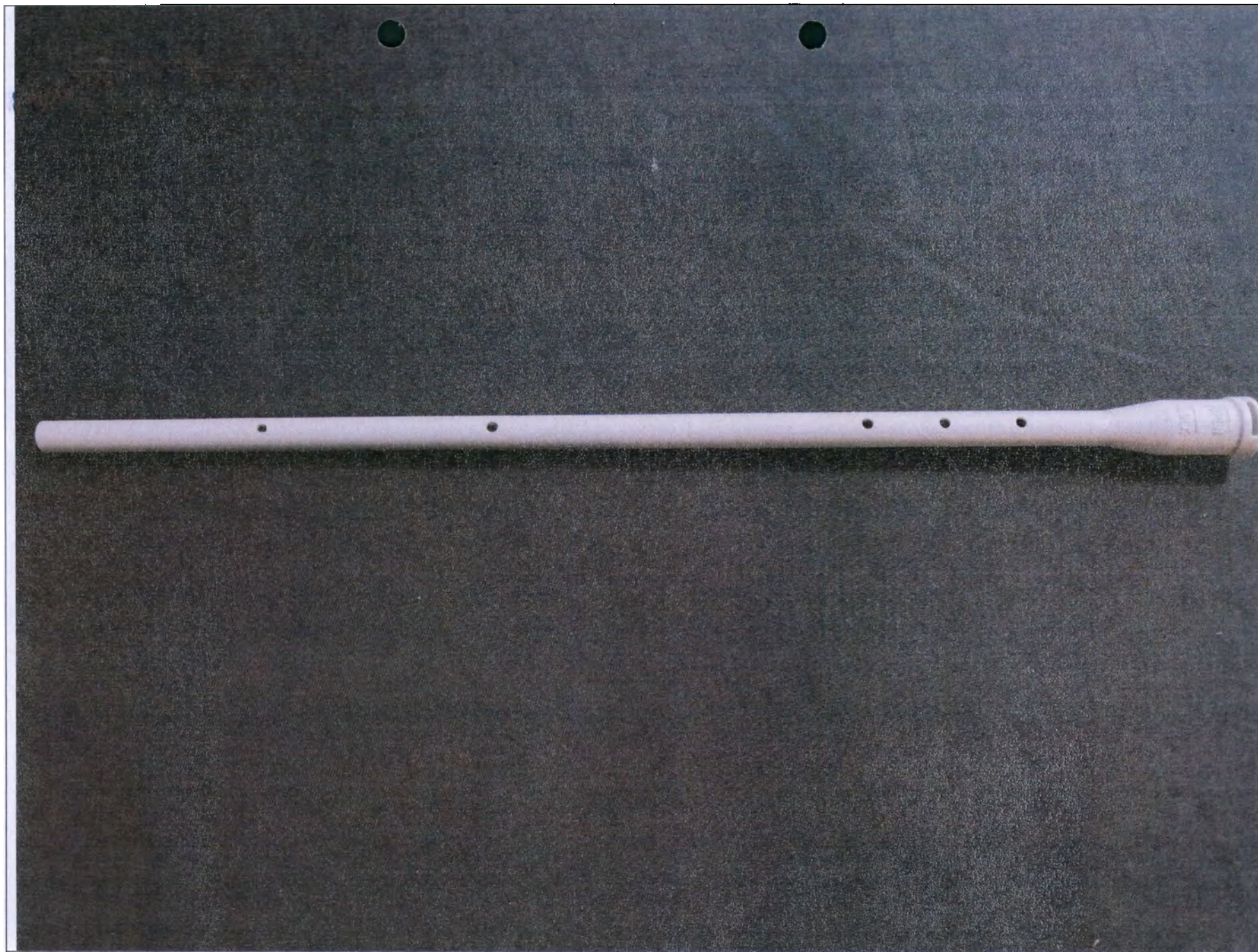
Рис. 20. Гильза защитная, для эндоскопов длиной 30 см.
