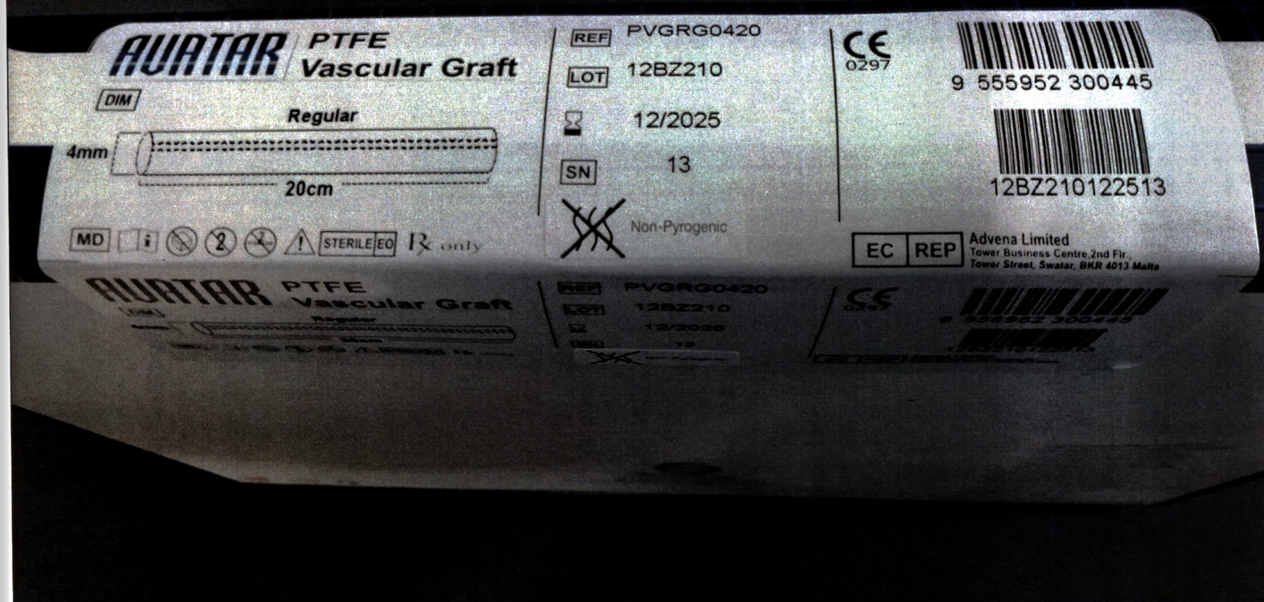
Рис. 20. Маркировка транспортной упаковки - Протез AVATAR сосудистый периферический прямой (на примере типоразмера: Длина 20 см, диаметр 4 мм).
