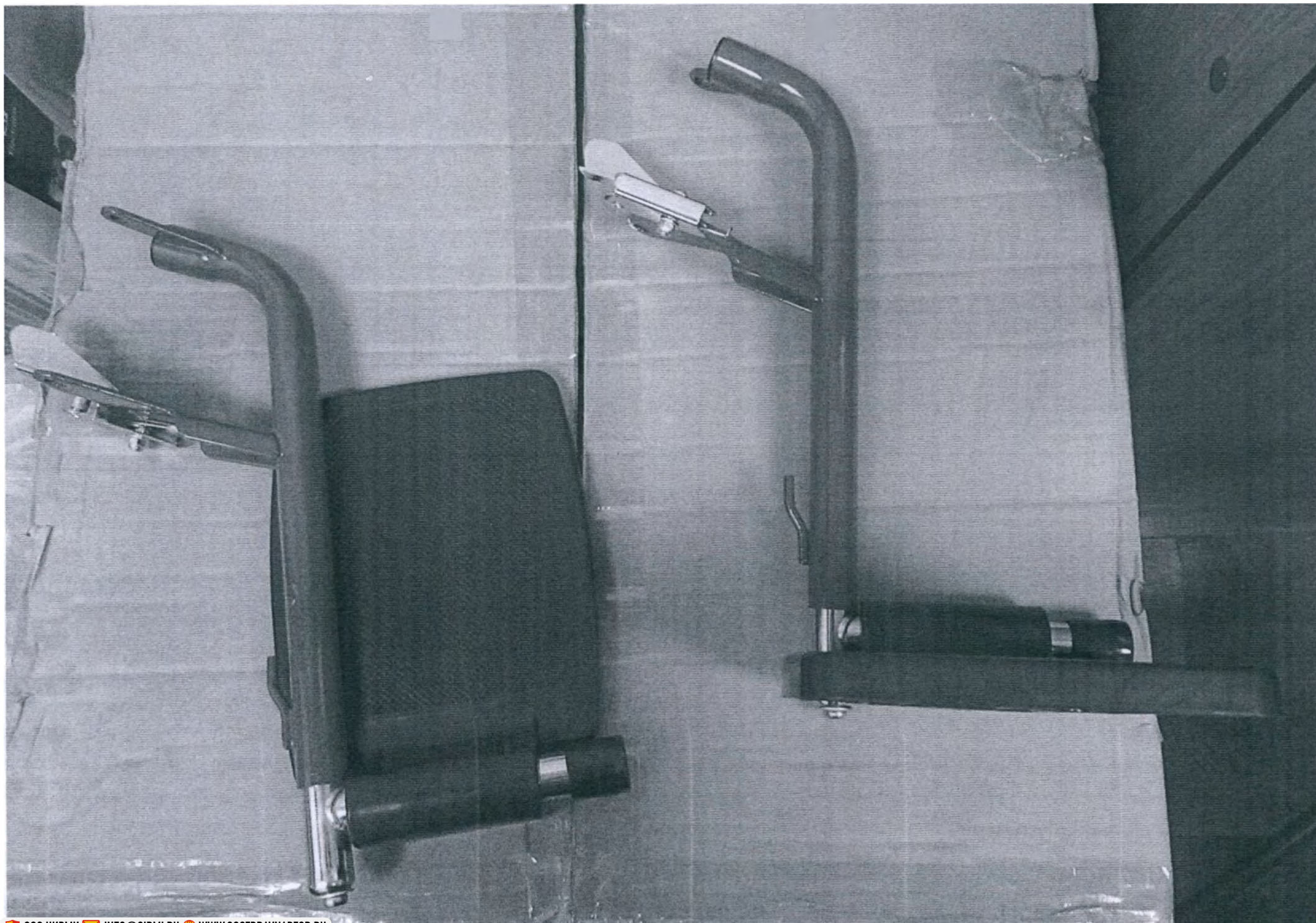
Рис. 84 – Подножка (2 шт.)
