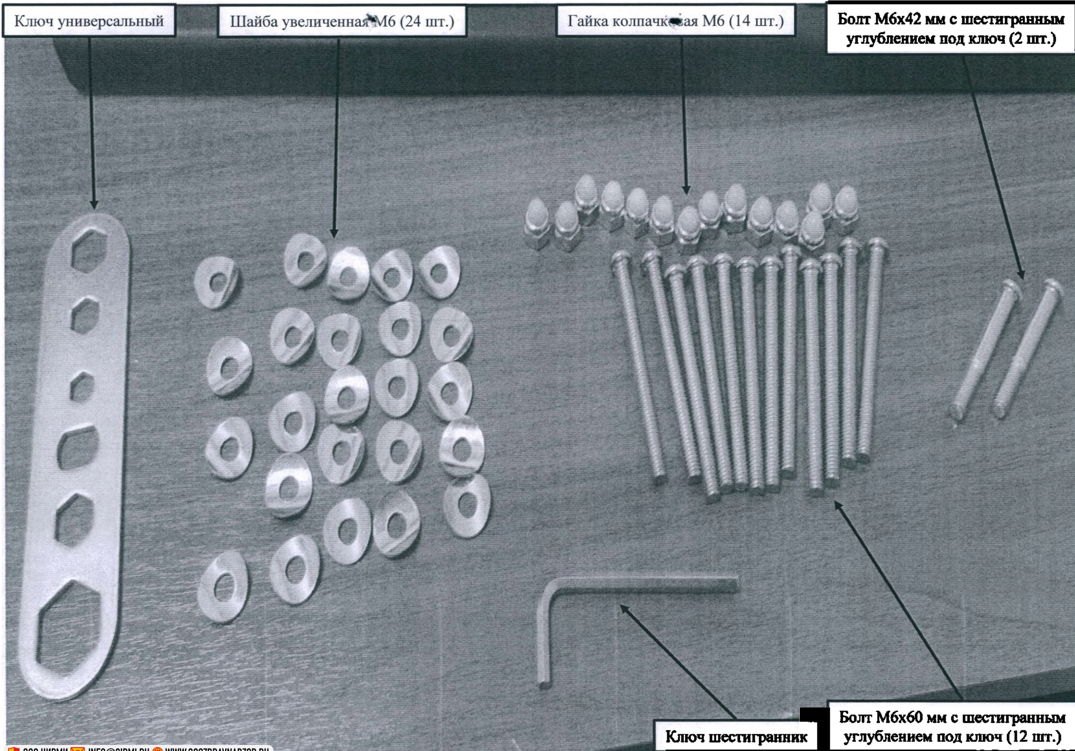
Рис. 72 – Комплект крепежа
