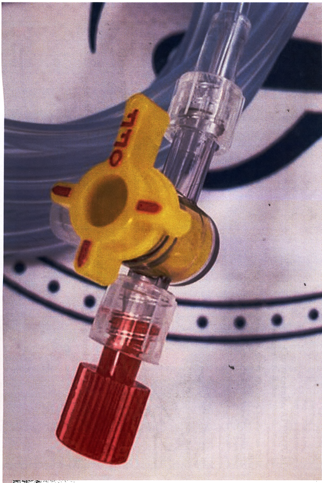
Фото 3 - Набор ирригационных трубок SmartAblate для электрофизиологических процедур в кардиологии в составе: Стопорный клапан.
