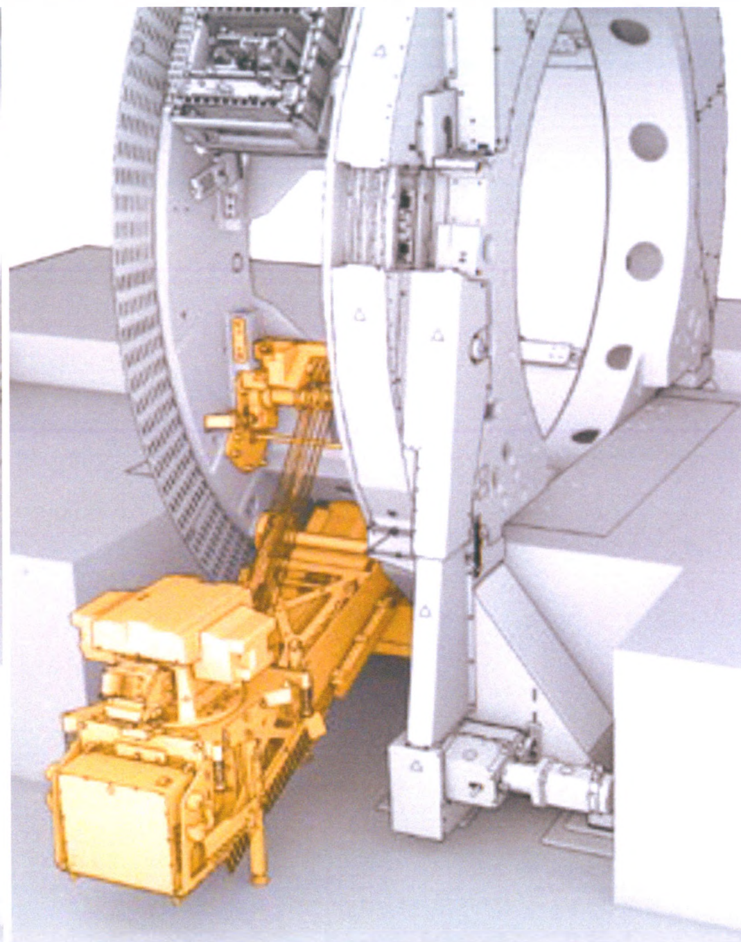
Линейный ускоритель медицинский Elekta Unity: Механизм SISO.
