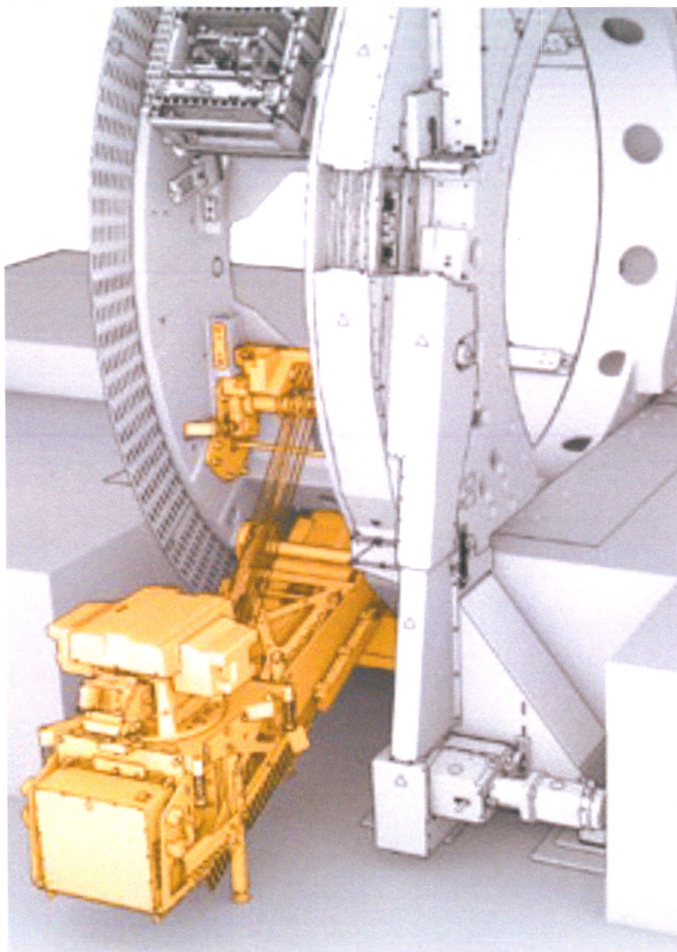
Линейный ускоритель медицинский Elekta Unity: Механизм SISO.
