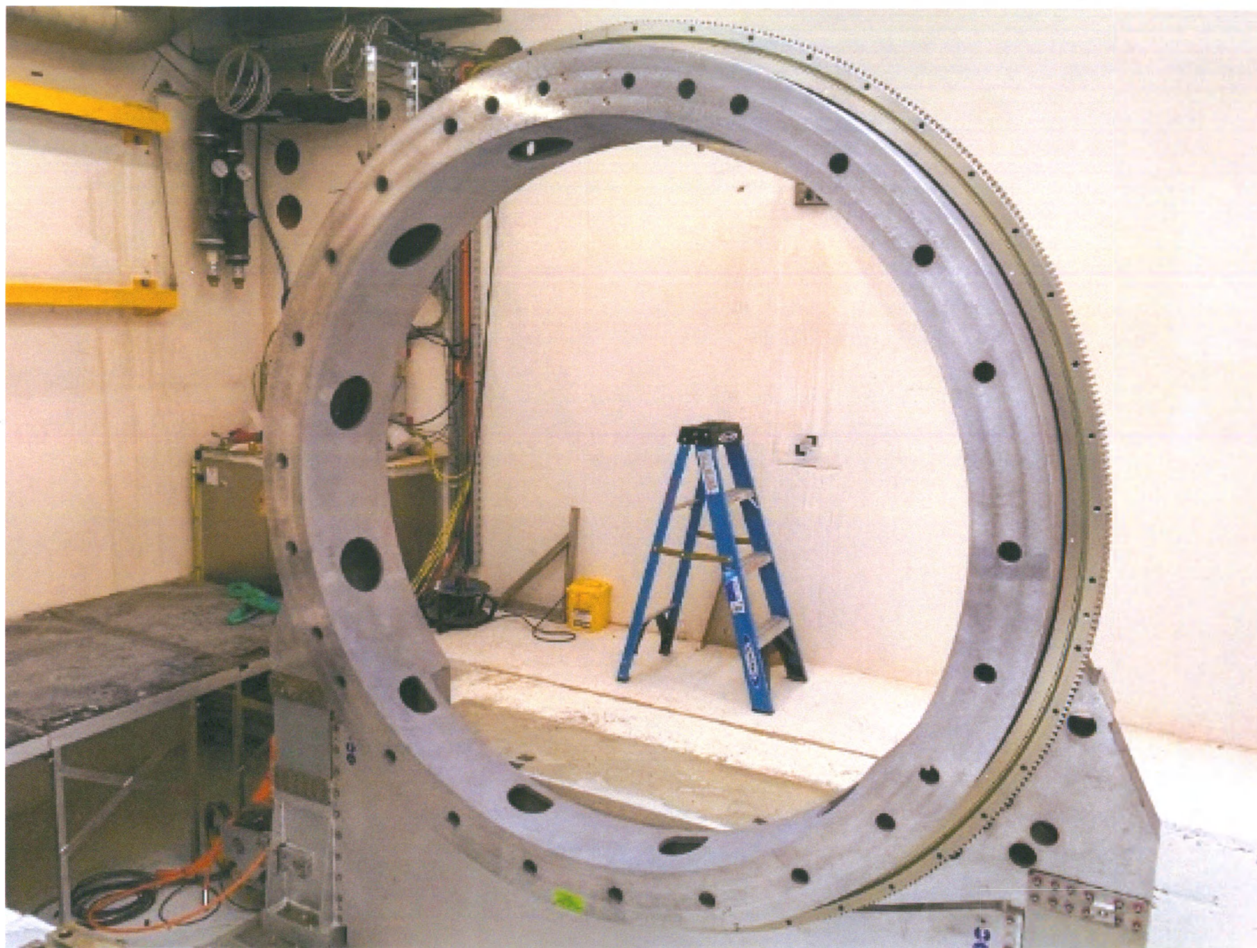
Линейный ускоритель медицинский Elekta Unity: Кольцо токосъемное
