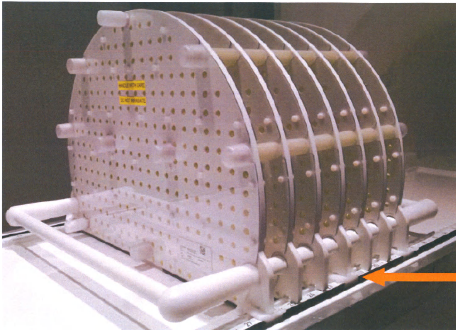
12.14. Фантом трехмерный геометрический 3D Geometric QA
