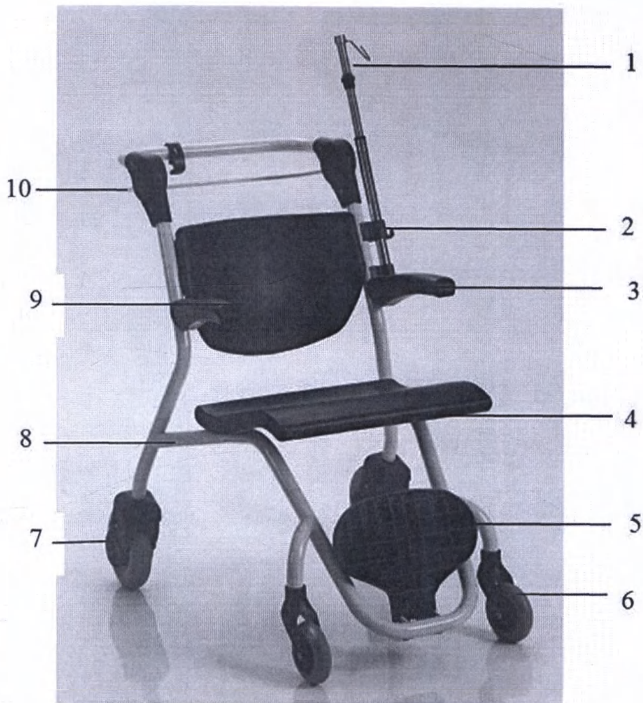
Средства медицинские NITROCARE для транспортирования пациентов. Кресло-каталка NTS X10: 1 – инфузионная стойка, 2 – подвес, 3 – открытие/закрытие поручня, 4 – сиденье, изготовленное в соответствии с требованиями эргономики, 5 – аппарат открытия/закрытия подножки, 6 – переднее колесо Ø 125 мм, 7 – заднее колесо Ø 200 мм, 8 – профиль корпуса, 9 – спинка, 10 – центральная система блокировки колес с педалью (центральный тормоз, заблокированный в парковочном положении)
