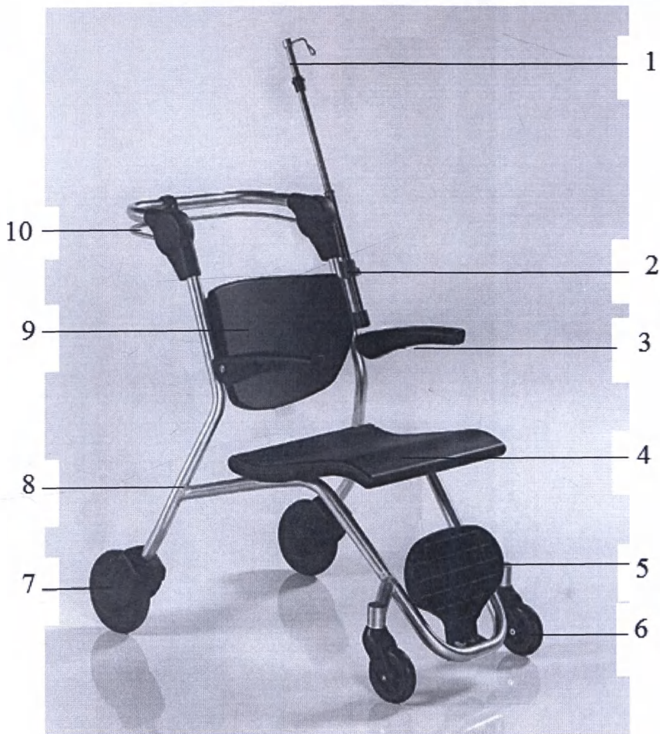
Средства медицинские NITROCARE для транспортирования пациентов. Кресло-каталка NTS X5: 1 - инфузионная стойка, 2 – подвес, 3 - открытие/закрытие поручня, 4 – сиденье, 5 – подножка, 6 - колесо Ø 125 мм, 7 - колесо Ø 200 мм, 8 - профиль корпуса, 9 –спинка, 10 - центральная система блокировки колес с педалью (центральный тормоз, заблокированный в парковочном положении)
