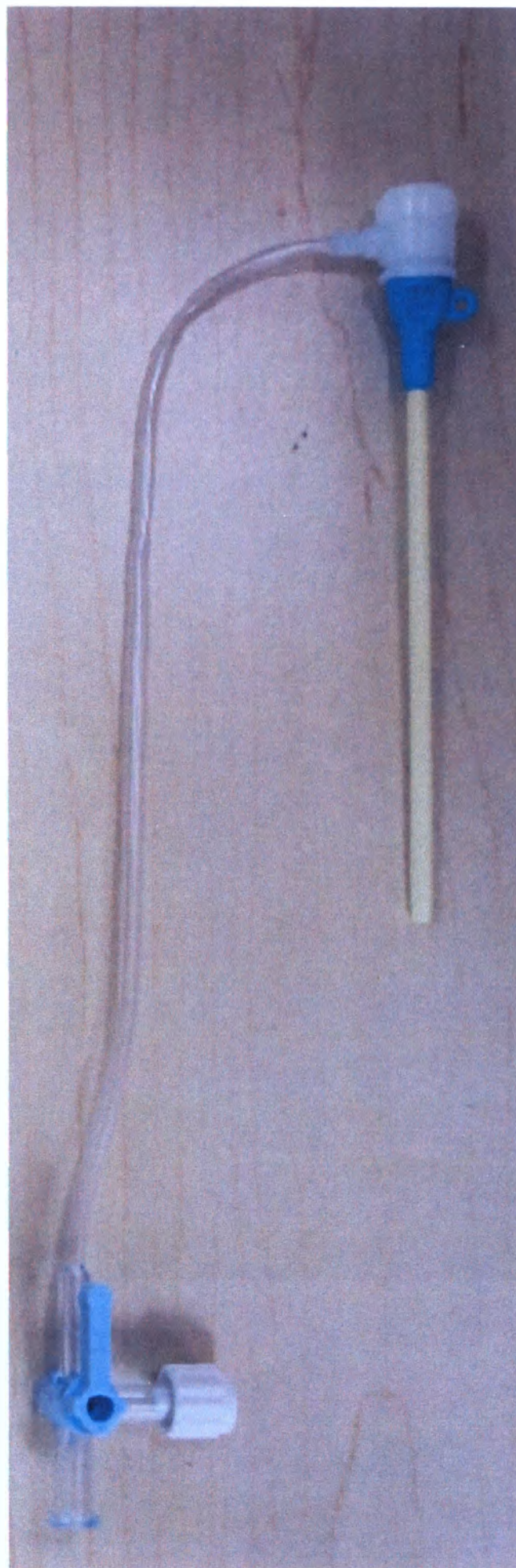
Рисунок 8. Внешний вид Интродьюсера с гемостатическим клапаном с номинальным наружным диаметром 3,4 мм и эффективной длиной 8 см
