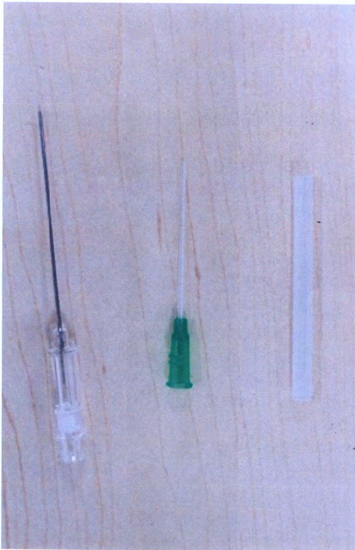
Рисунок 6. Внешний вид Иглы троакарной с номинальным внешним диаметром 0,90 мм и эффективной длиной 65 мм в комплекте с интродьюсерным катетером с номинальным внешним диаметром 1,3 мм и эффективной длиной 44 мм
