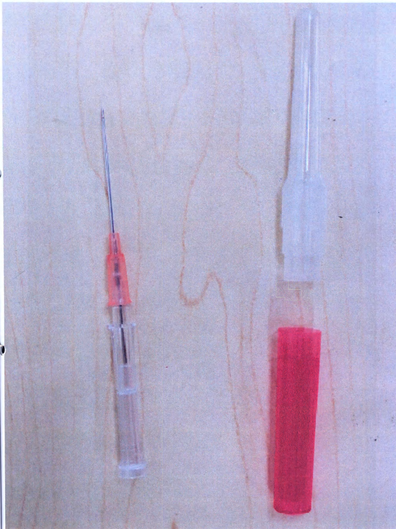
Рисунок 5. Внешний вид Иглы троакарной с номинальным внешним диаметром 0,70 мм и эффективной длиной 47 мм в комплекте с интродьюсерным катетером с номинальным внешним диаметром 1,1 мм и эффективной длиной 32 мм
