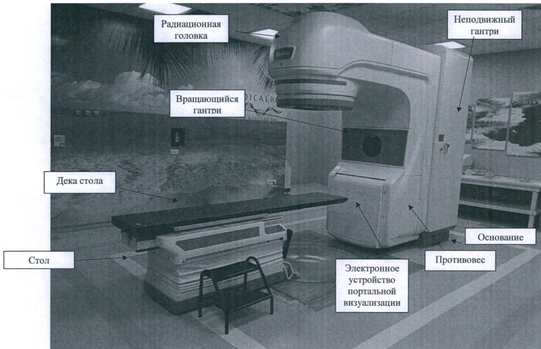
SHINVA XNA600E
