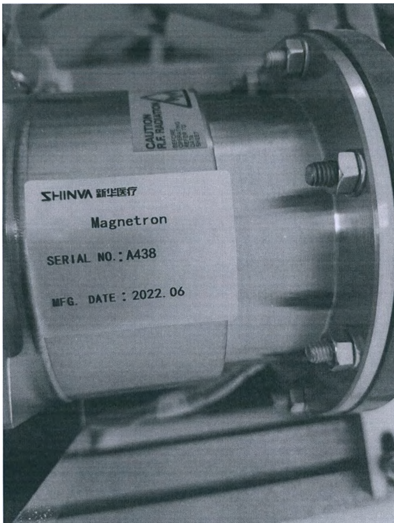
Маркировка: магнетрон
