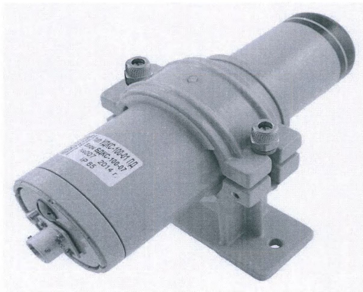
Система радиационного контроля - Устройство детектирования
