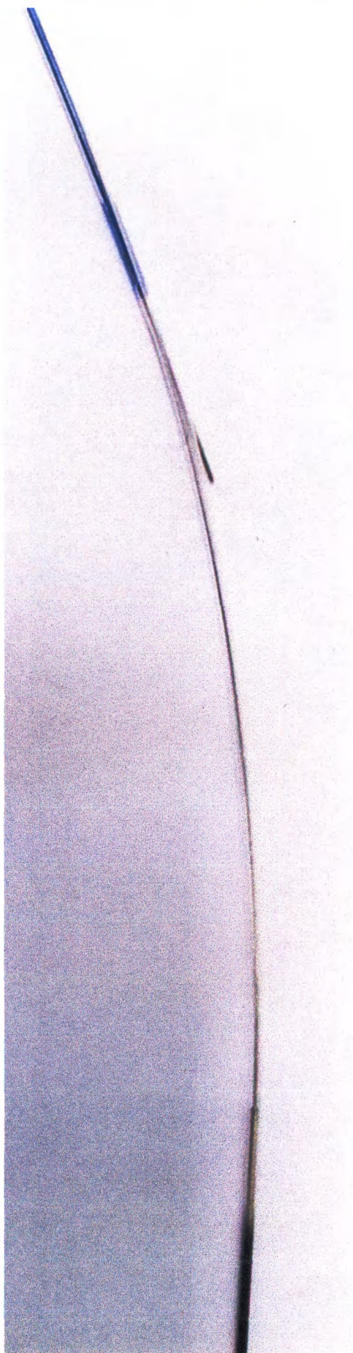
Рисунок 4. Внешний вид доставочного катетера, Rx порта и внутренней трубки
